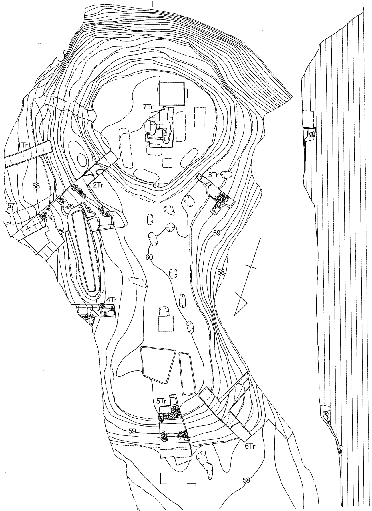
第5图 井原1号填調査区配置图 (1/200)
