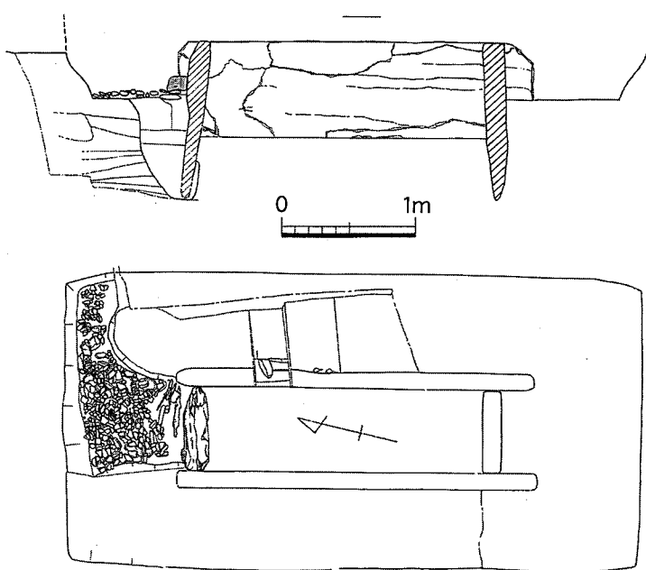
第18図 後円部箱式石棺構造復元図 (1/50)
