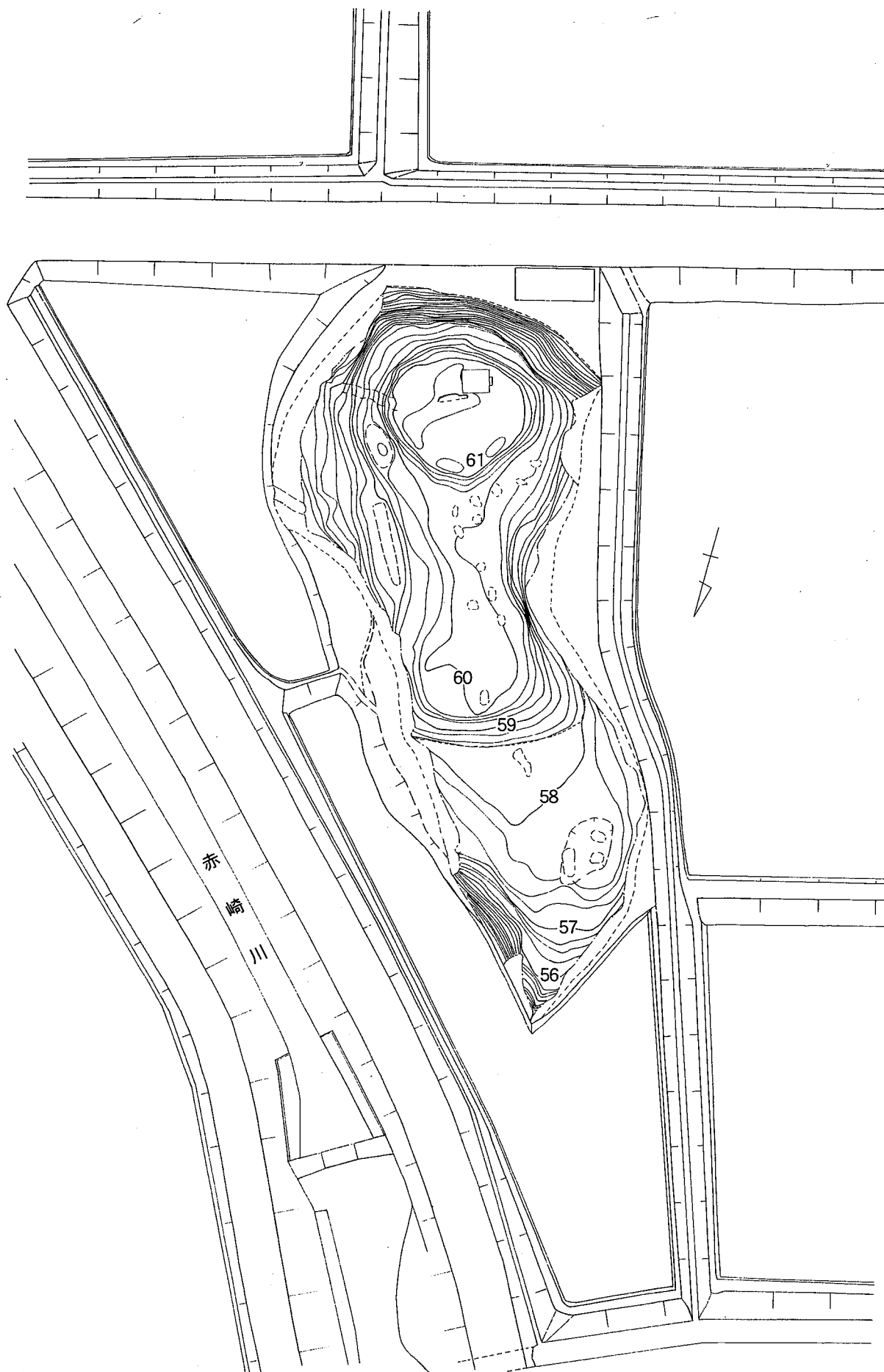
第4図 井原1号墳現況図 (1/500、平成14年6月現在)
