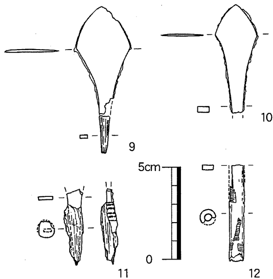
第16図 鉄器群B出土鉄器実測図 (1/2)
