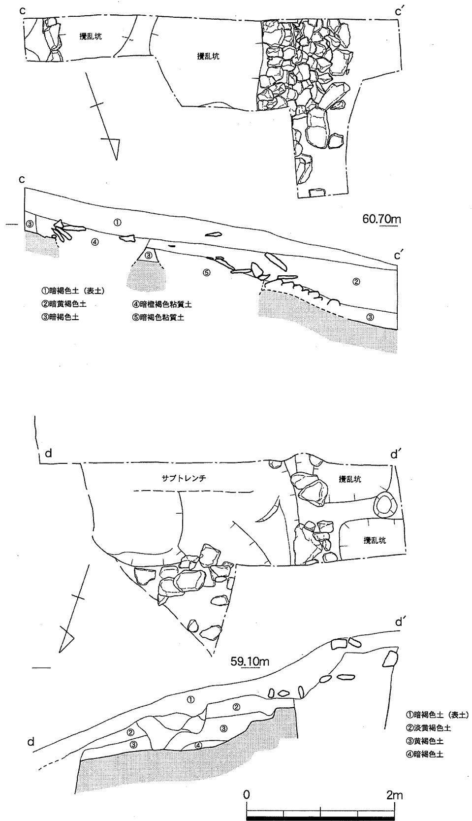
第8図 3、4トレンチ平面・土層断面図 (1/40)
