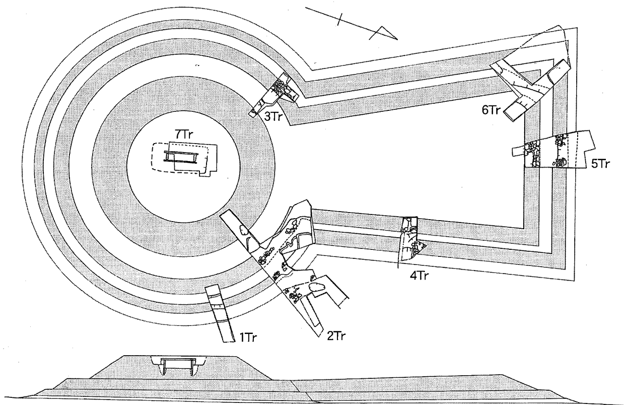
第17図 井原1号墳墳丘復元図 (1/300、アミかけ部は葺石範囲)
