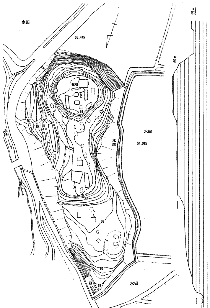
第3図 井原1号墳現況図(1/500、昭和61年当時)
