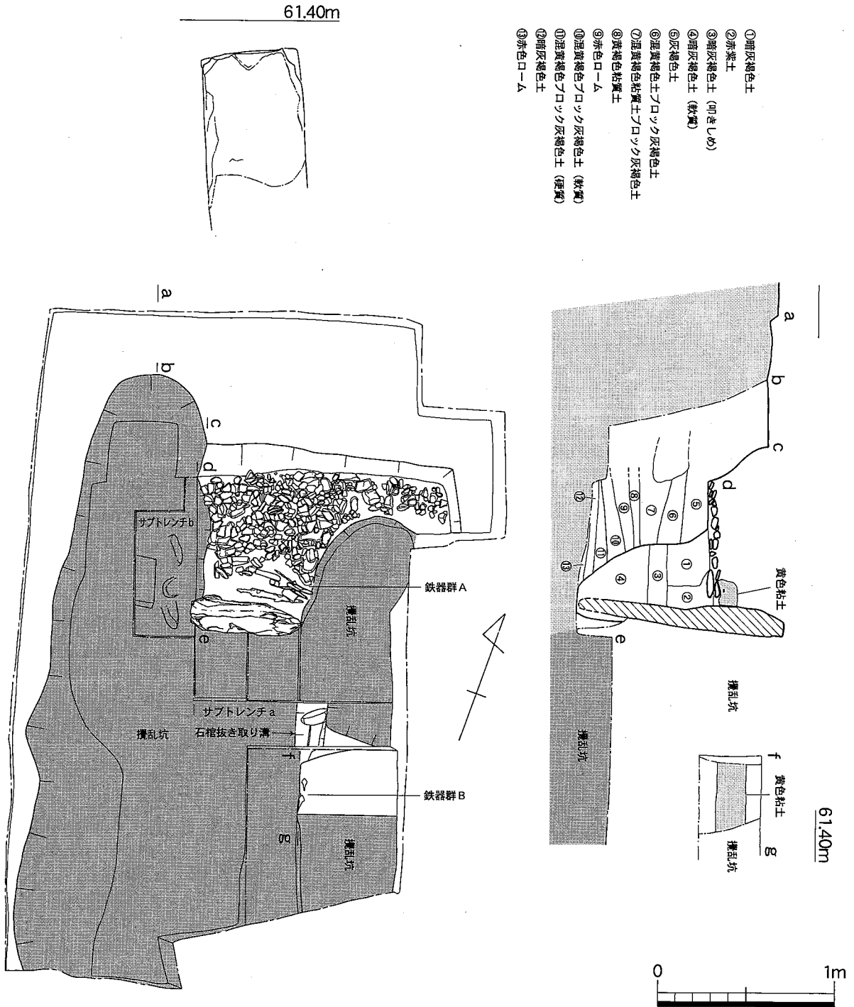
第12図 7トレンチ平面・土層断面図 (1/60)
