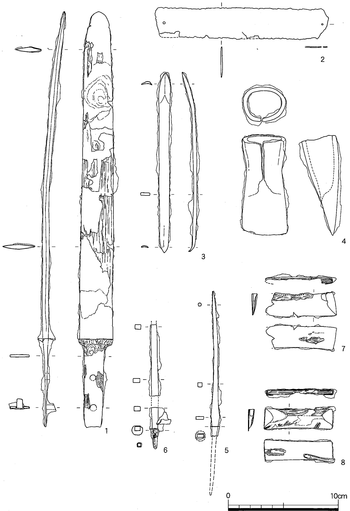
第15図 鉄器群A出土鉄器実測図 (1/2)
