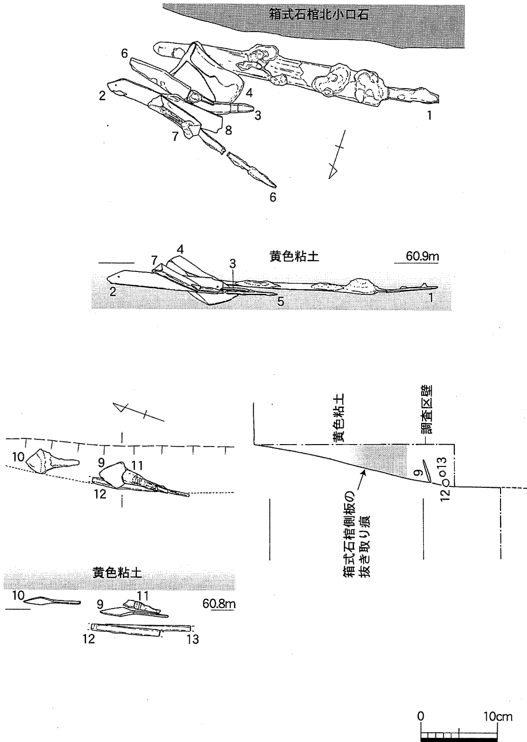
第14図 箱式石棺副葬鉄器出土状況図 (1/5)
