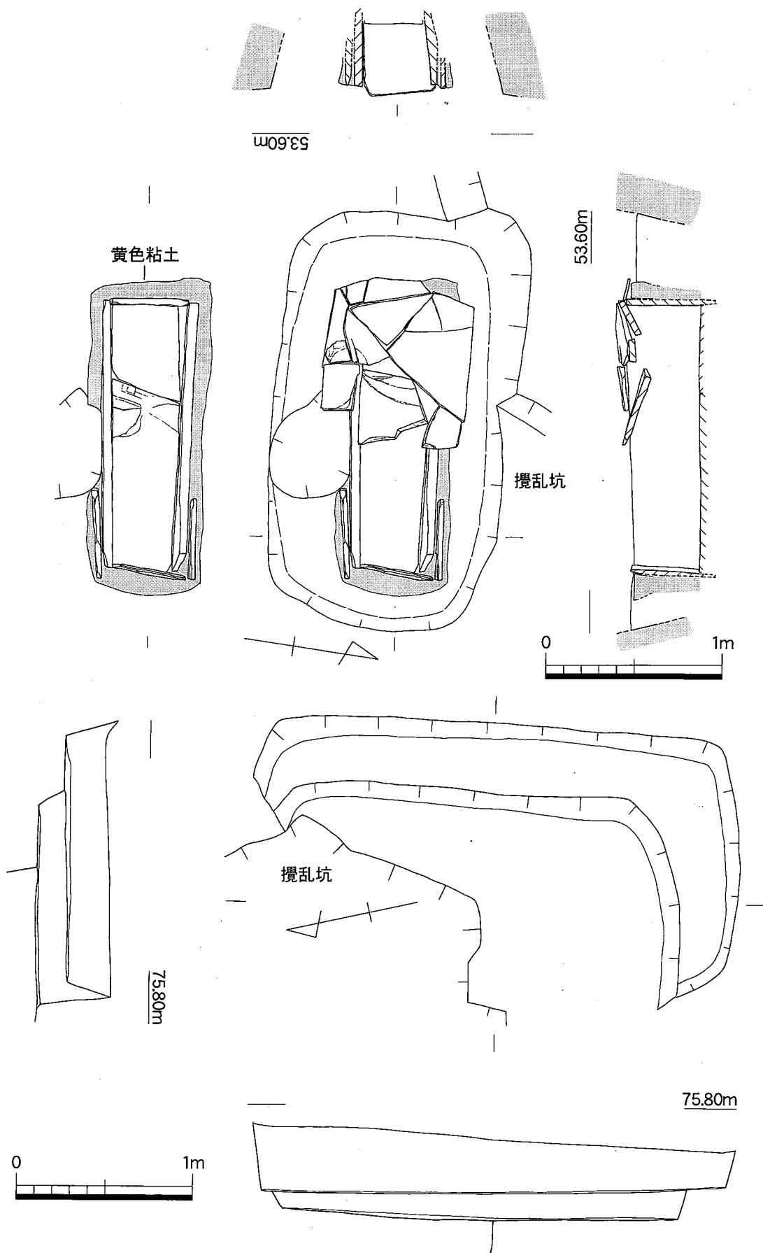
第26图 箱式石棺 (上)、土坑 (下) 实测图 (1/30)
