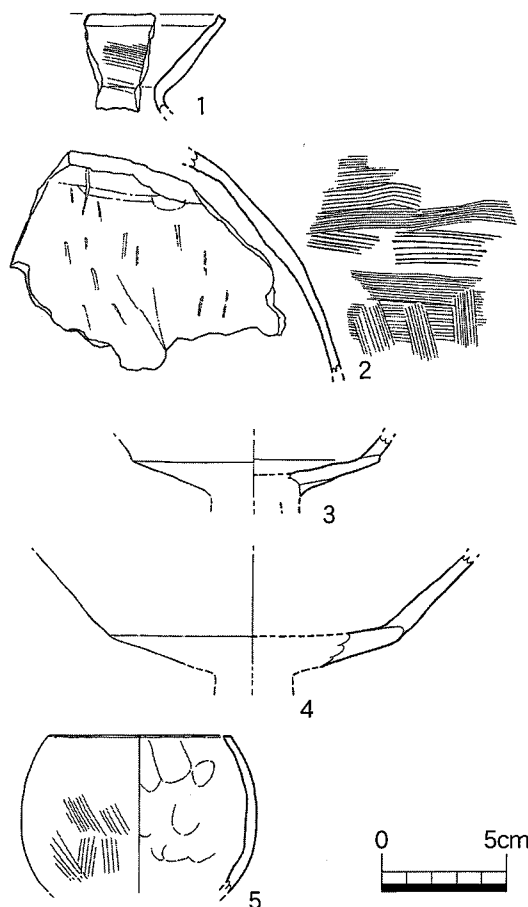
第11図 2 トレンチ出土土器実測図 (1/3)
