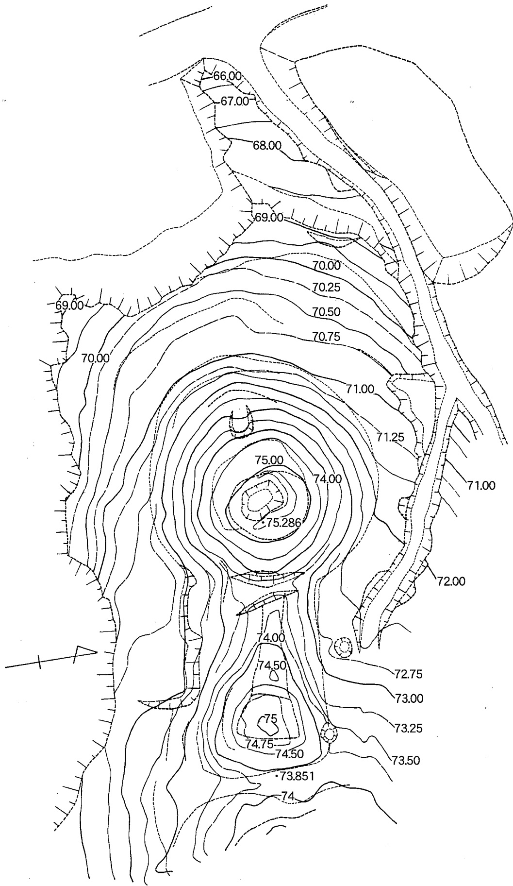
第21図 高祖東谷1号墳調査前現況図 (1/300)
