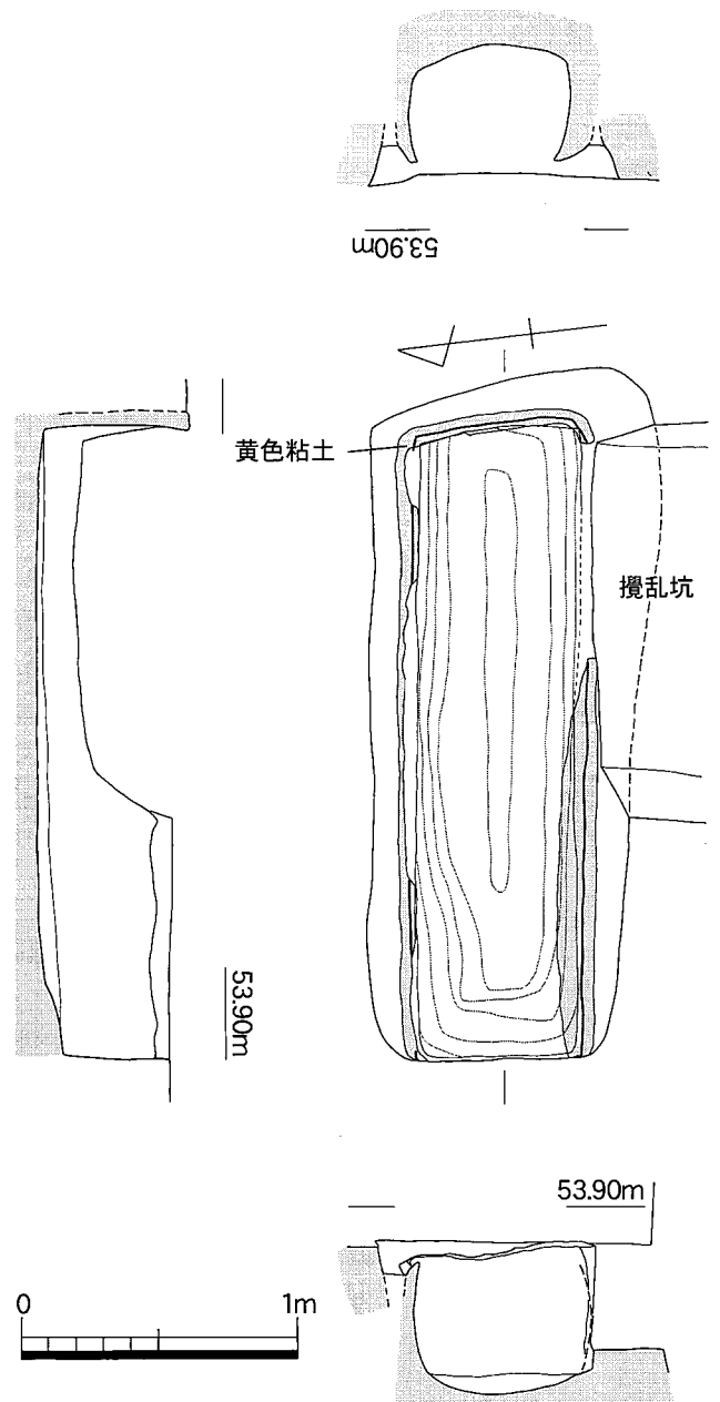
第25図 舟形木棺実測図（1/30）
