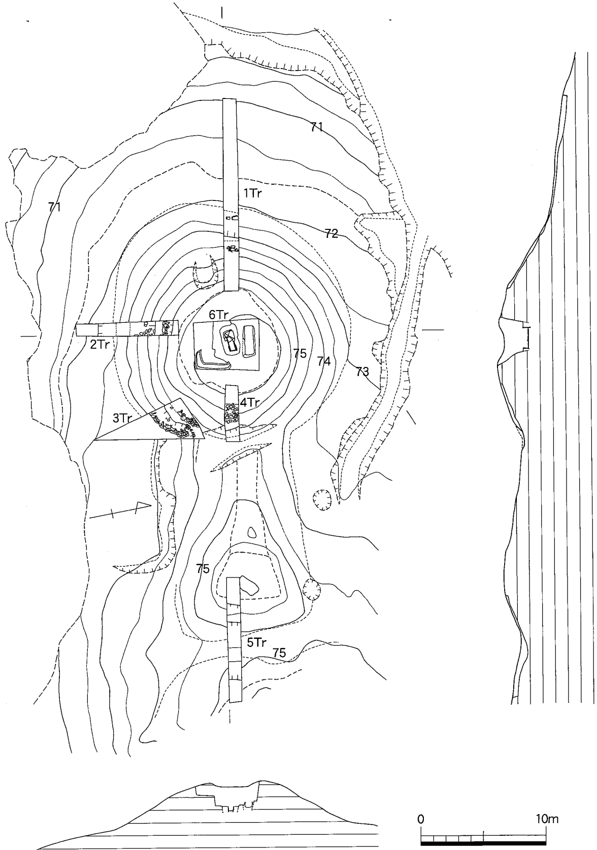
第22図 高祖東谷1号墳調査区配置図 (1/300)
