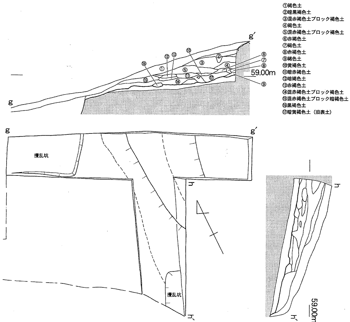
第10図 6 トレンチ平面・土層断面図 (1/60)
