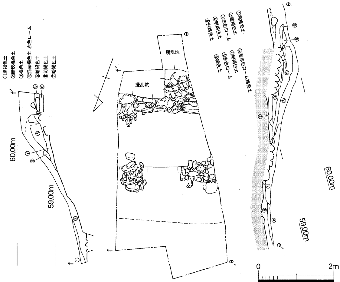
第9図 5 トレンチ平面・土層断面図 (1/60)
