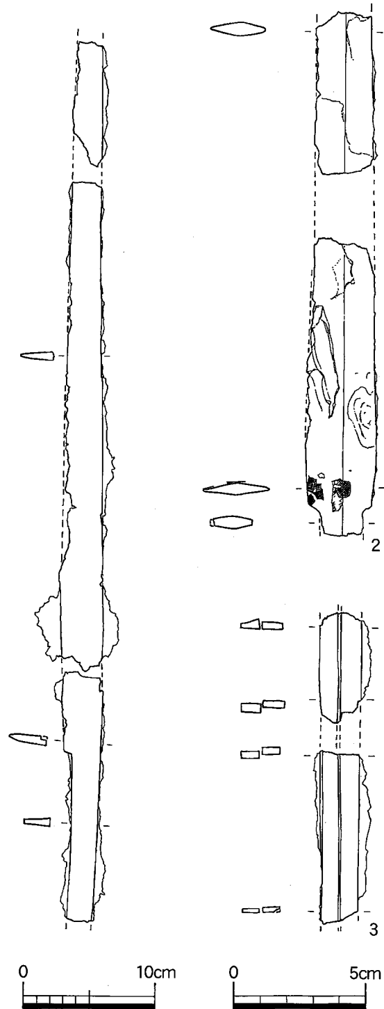
第27図 カクラン坑出土鉄器実測図 (1/4、1/2)
