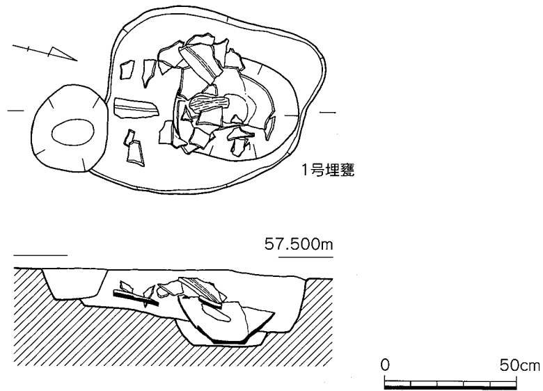
第9图 1号掘立柱建物·1号埋甕平断面实测图 (1/40·1/20)
