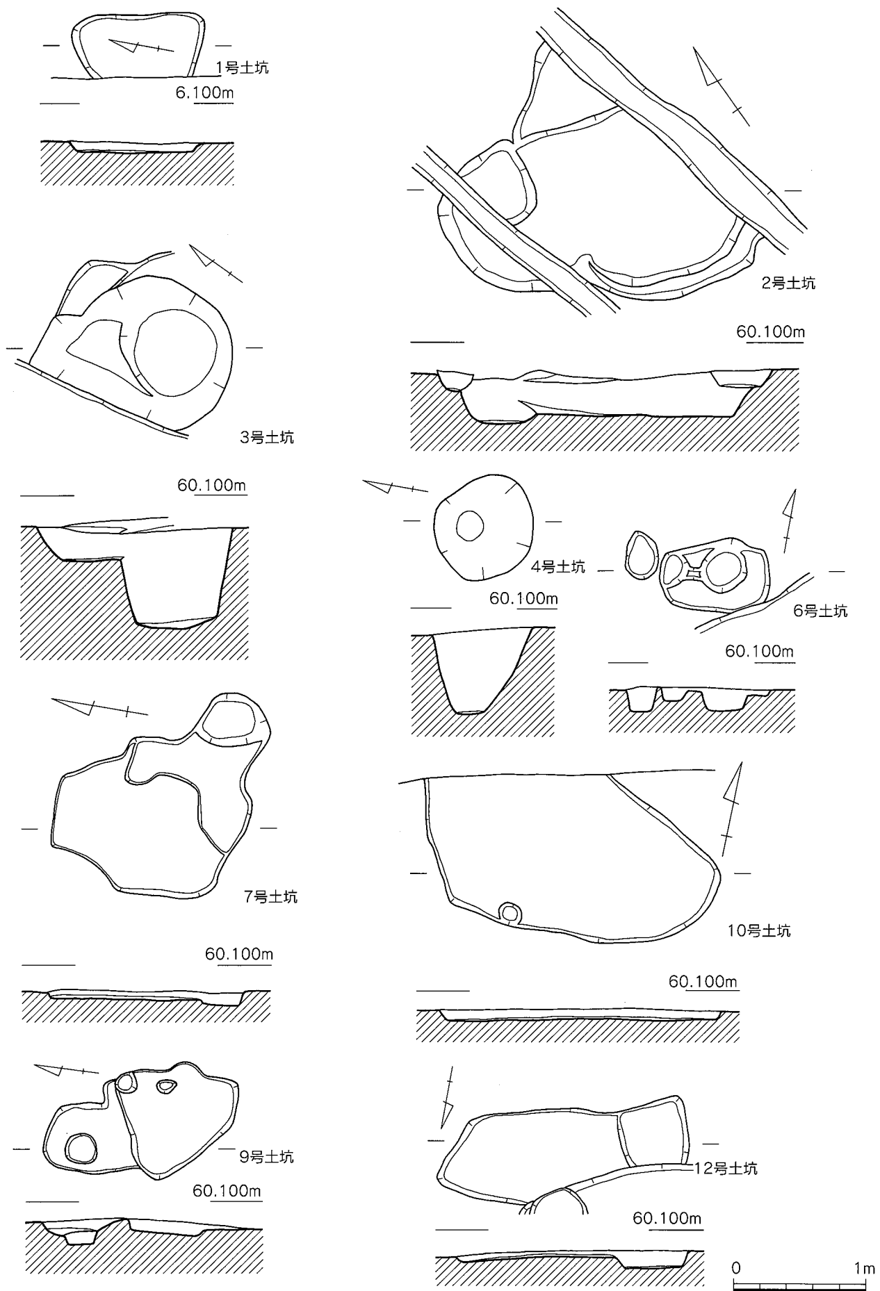
第18图 1~4、6、7、9、10、12号土坑平断面实测图 (1/40)
