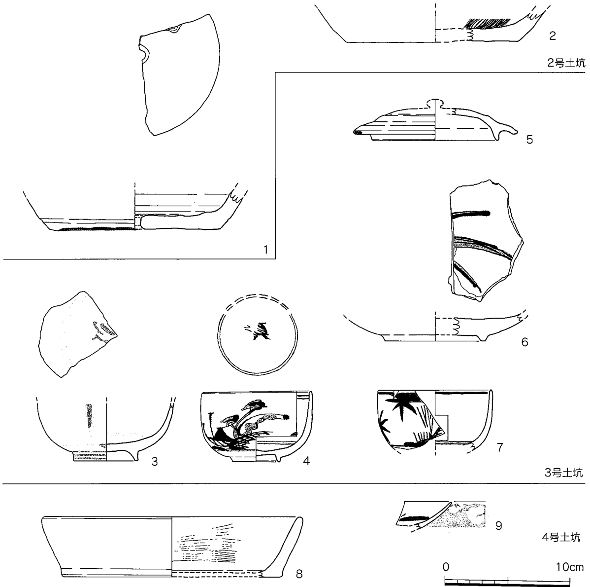
第19図 2～4号出土遺物実測図 (1/3)
