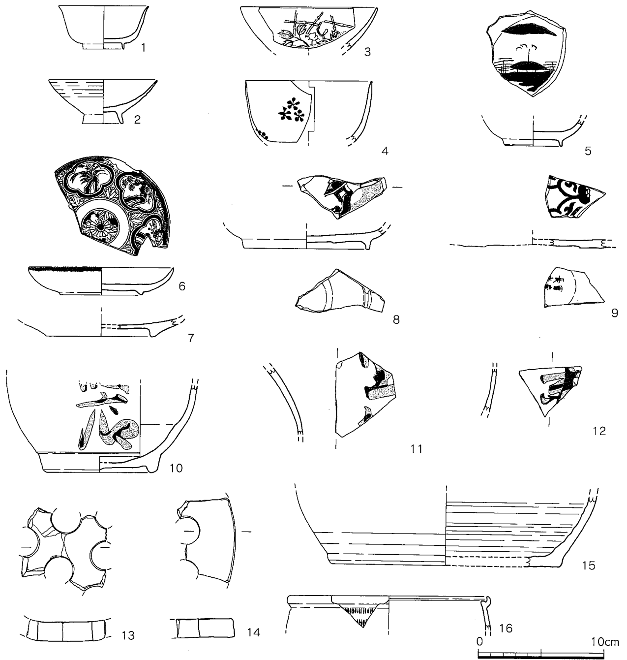
第5図 石垣状遺構出土遺物実測図 (1/3)
