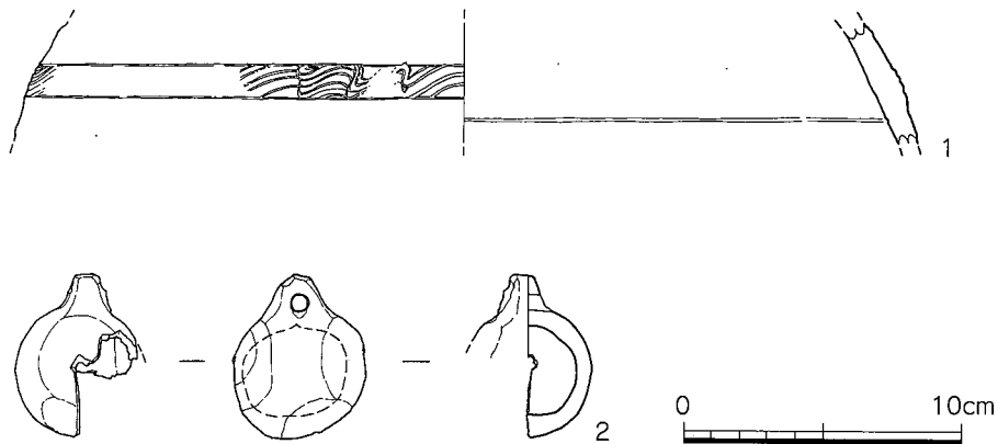
第21図 1・2号ピット出土遺物実測図 (1/3)
