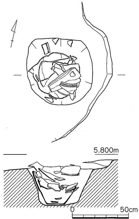
第15図 2号埋甕平断面実測図 (1/20)
