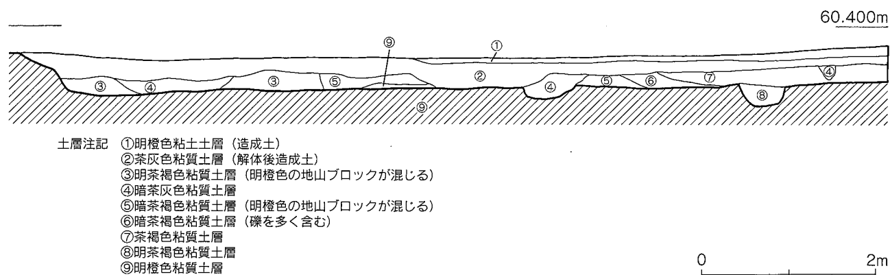
第3図 東壁土層断面実測図 (1/60)
