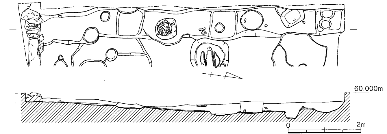
第6図 布振り基礎建物平断面実測図 (1/60)
