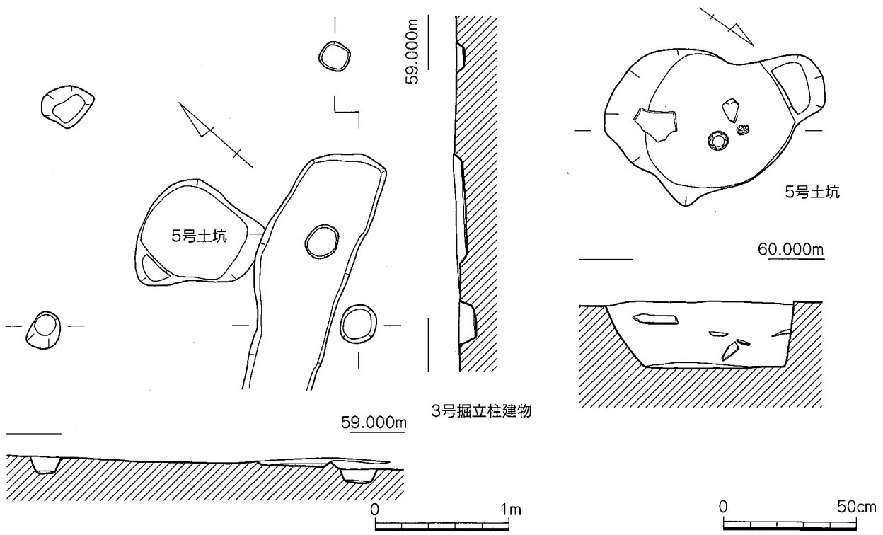
第11图 3号掘立柱建物、5号土坑平面断面实测图 (1/40、1/20)
