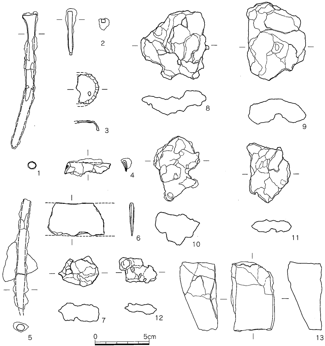
第22図 鉄器・石器実測図 (1/2)
