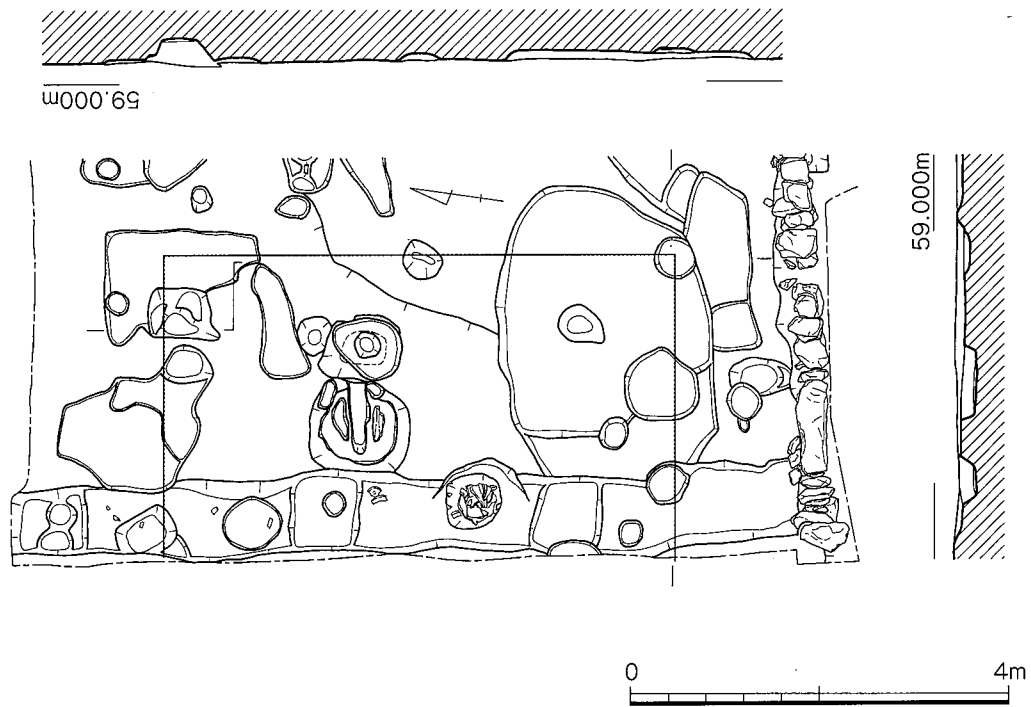
第10図 2号掘立柱建物平断面実測図 (1/80)
