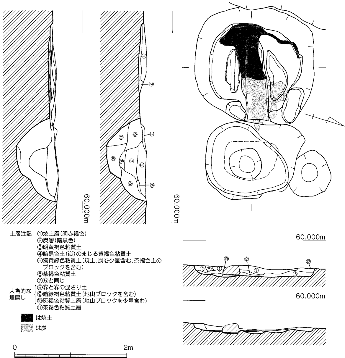
第13図 焼土坑平面断面実測図 (1/20)
