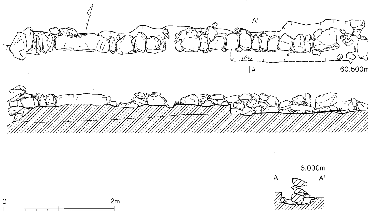
第4図 石垣状遺構平面実測図 (1/40)
