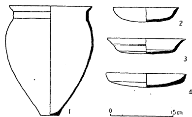
第27図 真間式土器
