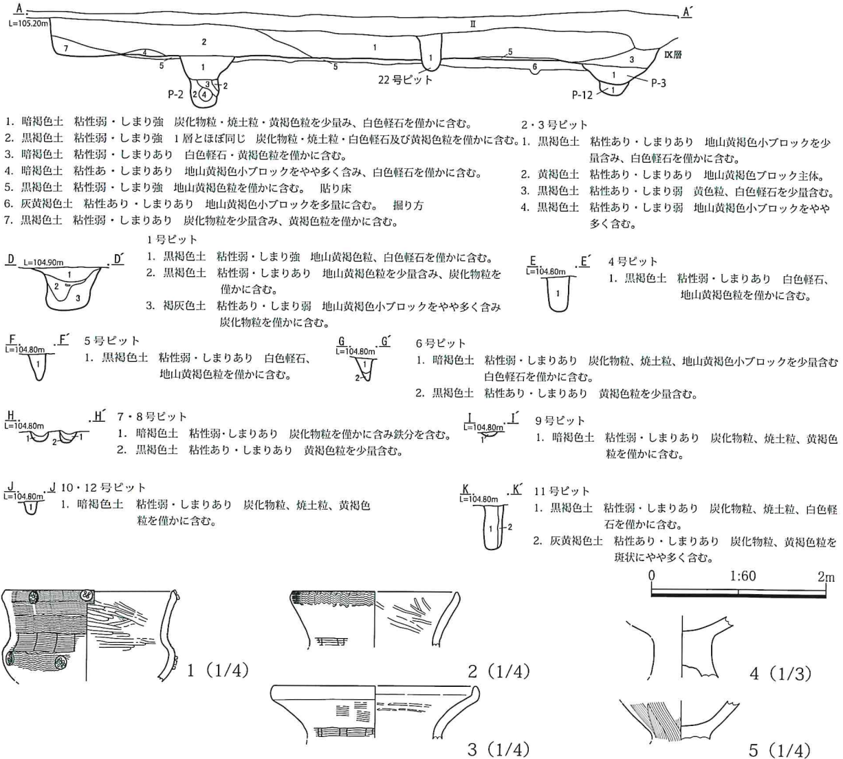
第7図 1号住居 断面図 (1/60) 出土遺物図
