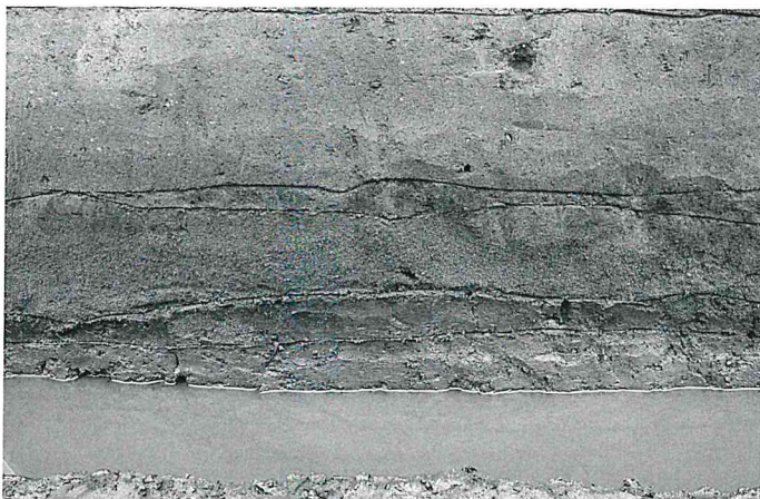
B下水田畦畔断ち割りセクション 北から
