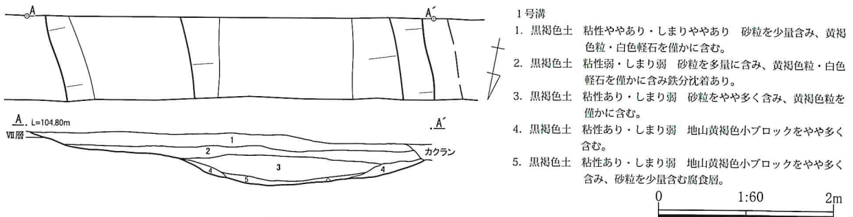
第16図 1号溝 平面図・断面図(1/60)
