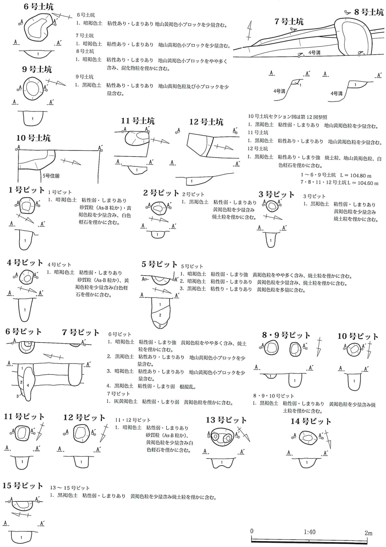
第21図 6～12号土坑 1～15号ピット 平・断面図 (1/40)
