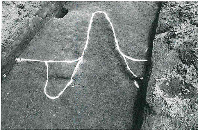
2号住居カマド全景 西から
