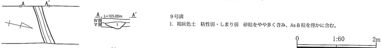
第19図 6~9号溝 平面図・断面図 (1/60)
