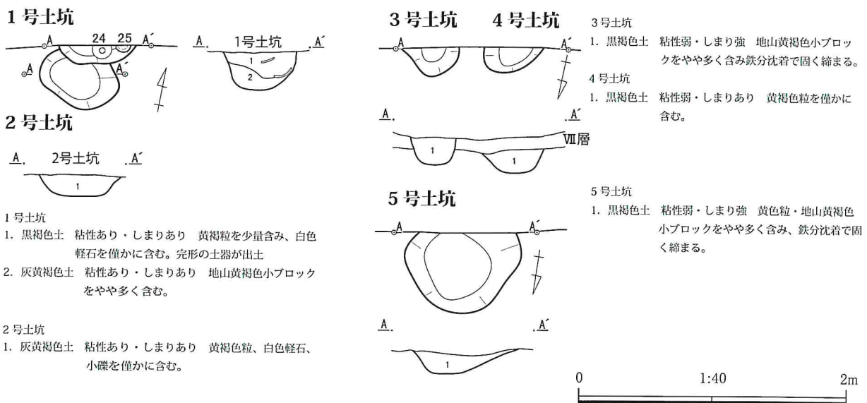
第20図 1～5号土坑 平面図・断面図(1/40)
