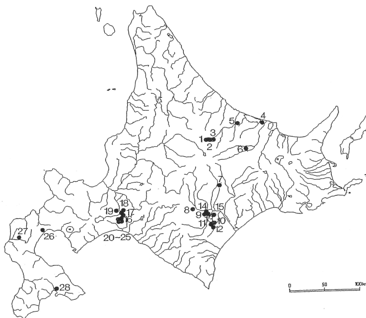
図27 北海道地方における後期旧石器時代前半期の遺跡位置図
