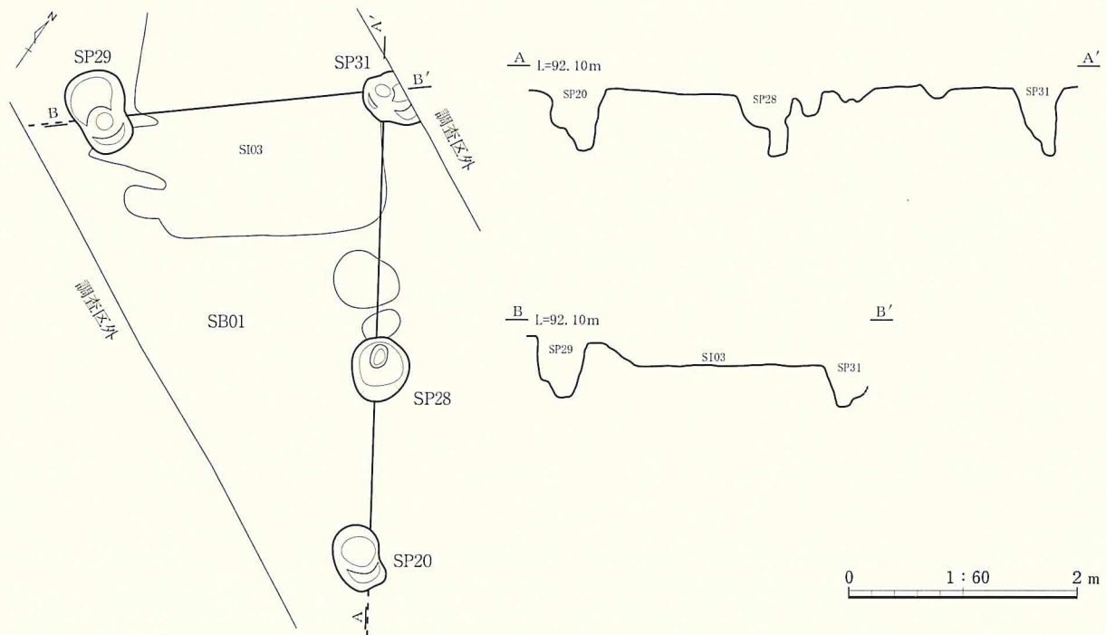
第13図 1号掘立柱建物平面図・断面図
