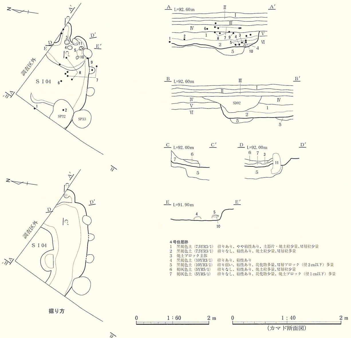
第11図 4号住居跡平面図・断面図
