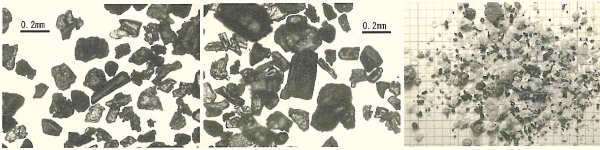
SZ01南西部・試料18(Hr-FA混在) 中央:角閃石 中央左上:中間型ガラス
