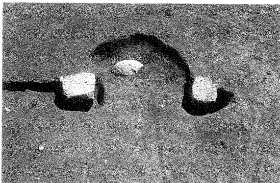
48号住居跡カマド (W→)
