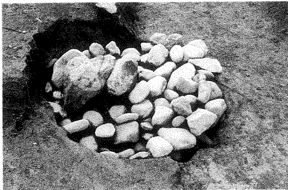
51号土坑 礫出土状態 (N→)
