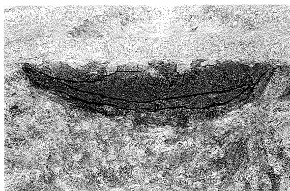
北側側溝 土層堆積状態 (W→)
