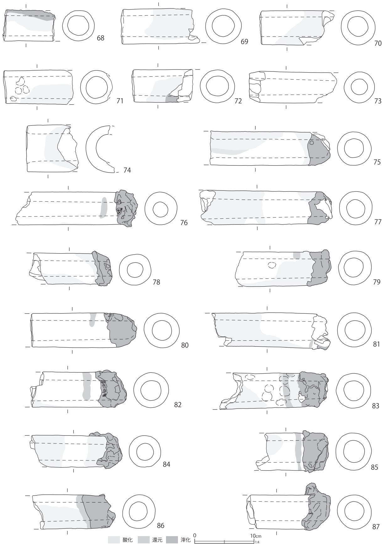
第 591 図 鍛冶関連遺物 (6)
