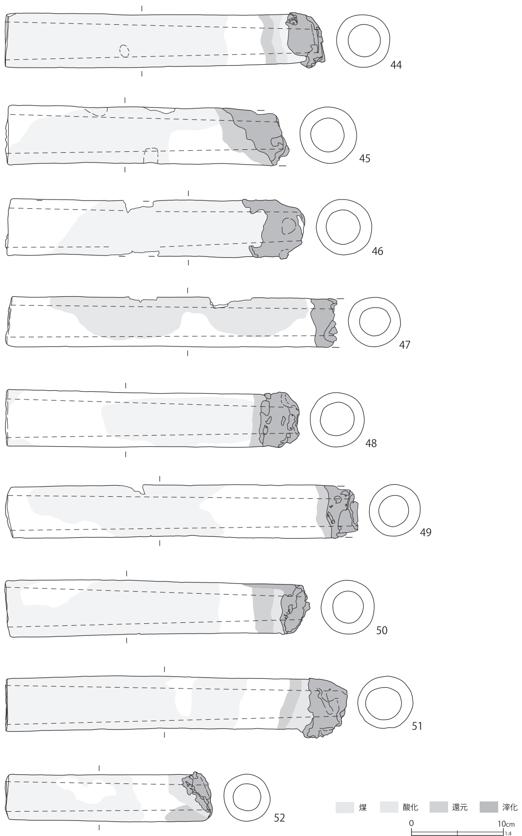
第 589 図 鍛冶関連遺物（4）
