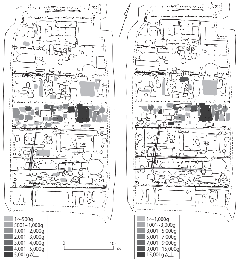
第 608 図 鉄滓（右）と鞆の羽口（左）の重量別分布図
