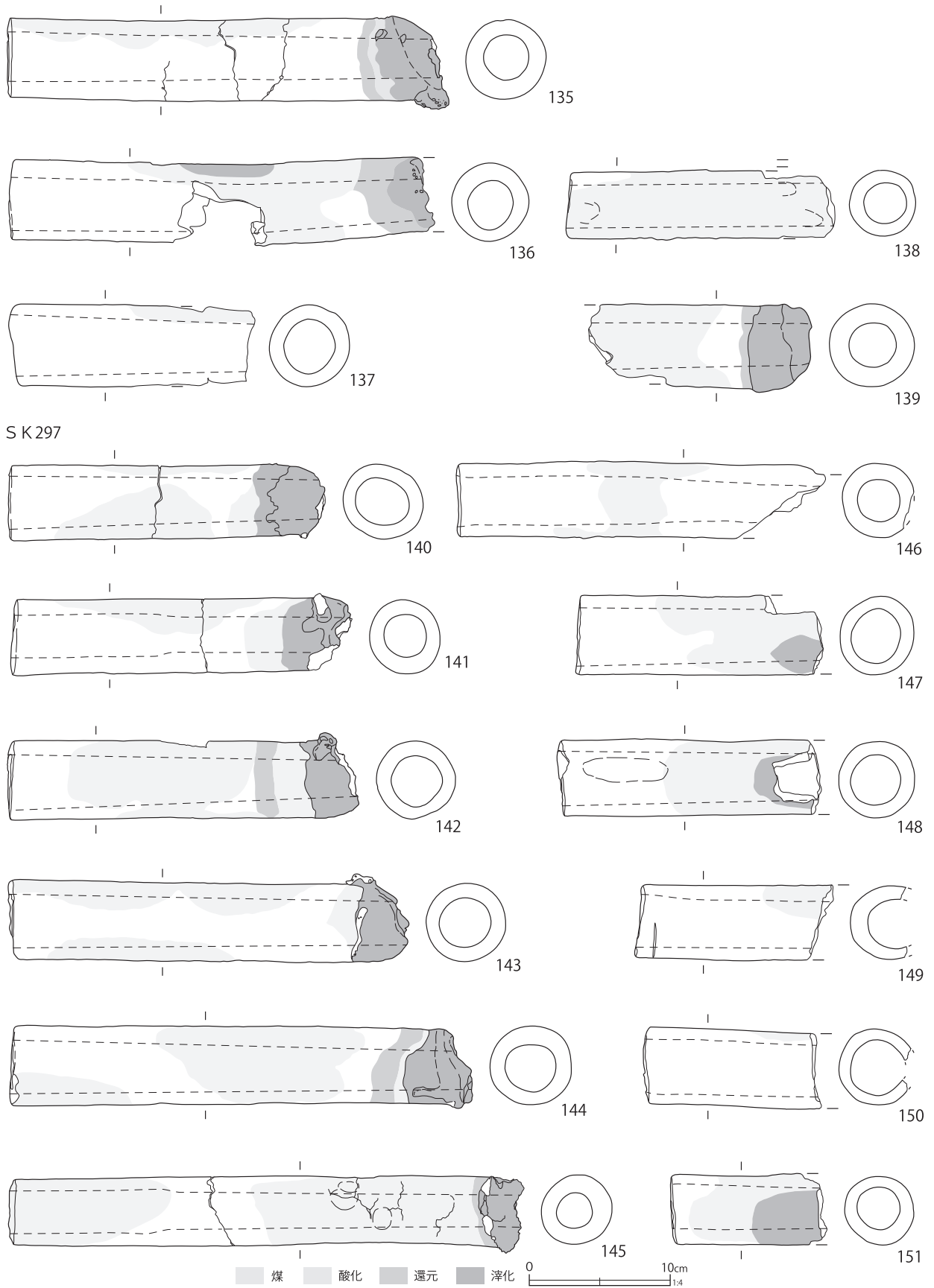
第 595 図 鍛冶関連遺物 (10)
