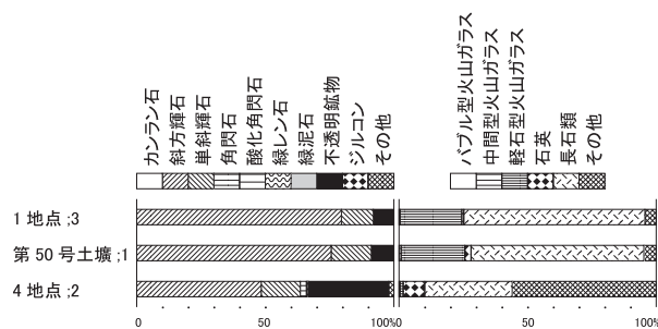
第 603 図 重軽鉱物組成
