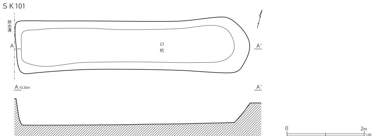
第 477 図 第 101 号土坑
