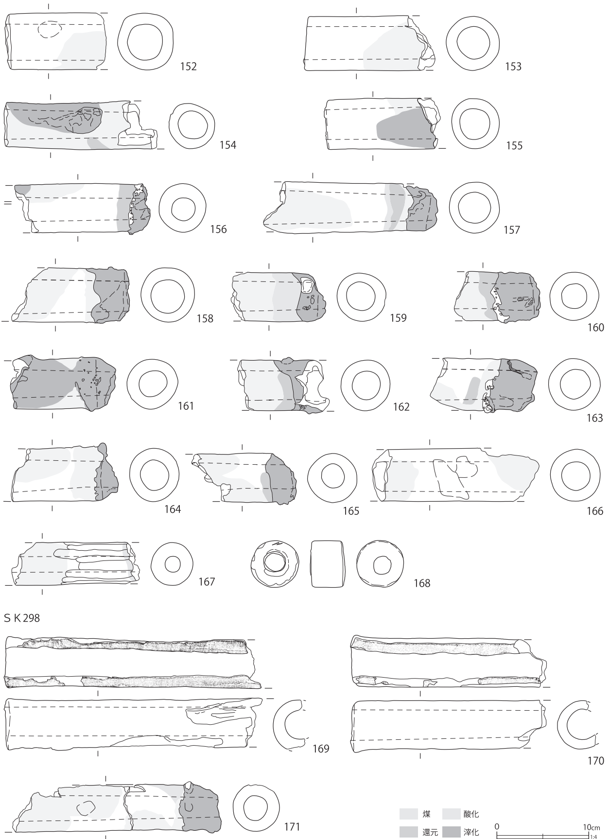
第 596 図 鍛冶関連遺物 (11)
