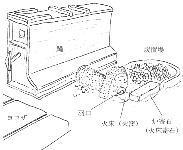
第 607 図 鍛冶炉周辺の想定図（魚水環 画）
