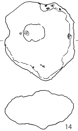
第 600 図 鍛冶関連遺物 (15)
