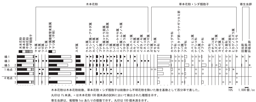
第604図 花粉化石群集・寄生虫卵
