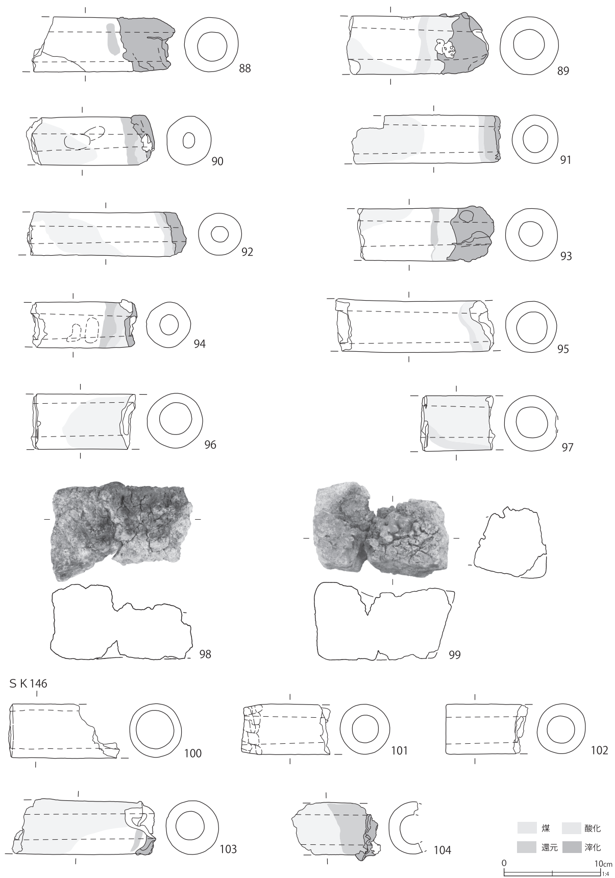
第 592 図 鍛冶関連遺物 (7)
