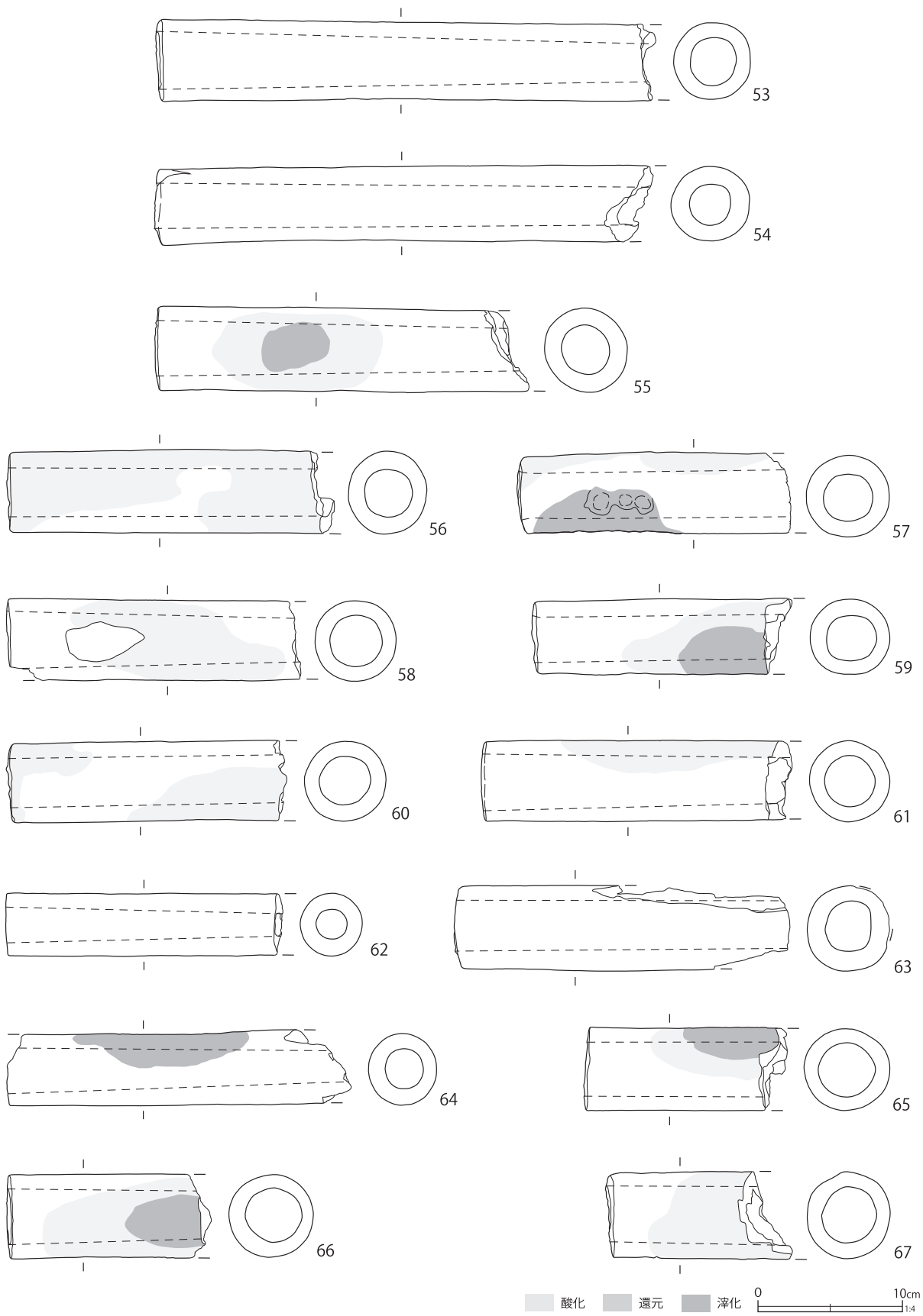
第 590 図 鍛冶関連遺物 (5)
