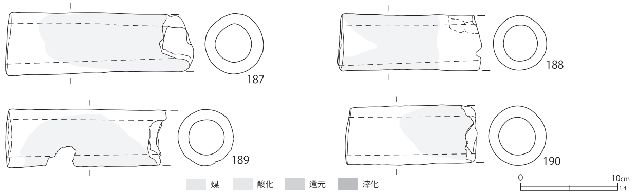
第 597 図 鍛冶関連遺物 (12)
