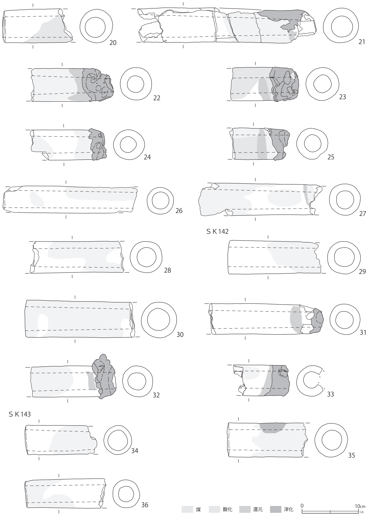
第 587 図 鍛冶関連遺物 (2)
