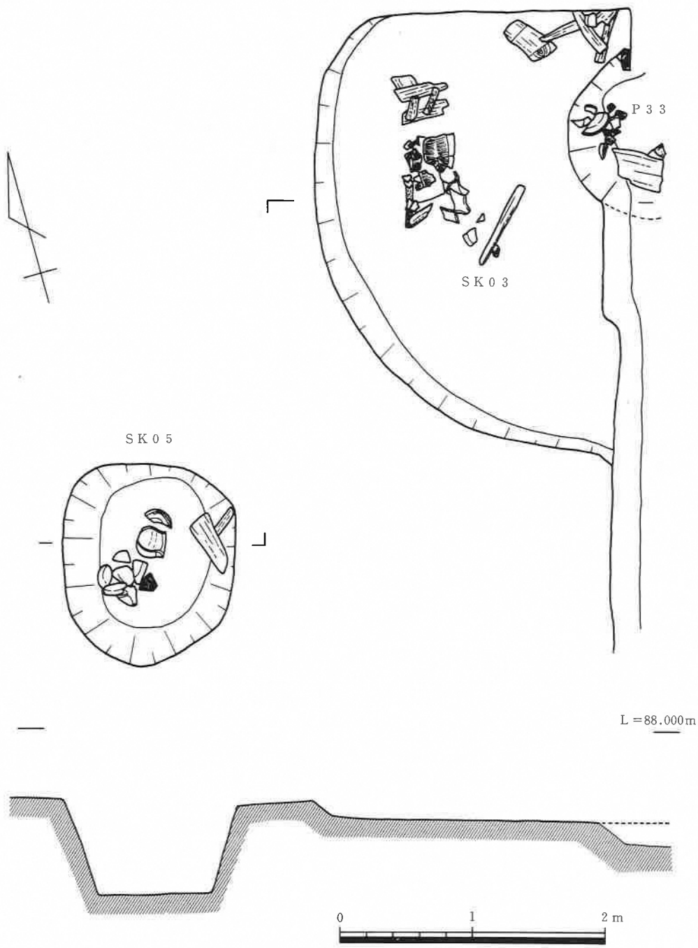
fig 12 24トレンチSK03,SK05,P33実測図
