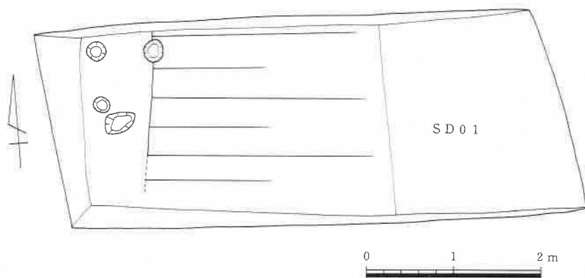
fig 3 12トレンチ遺構平面図
