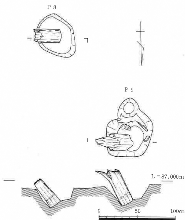
fig 8 18トレンチSB01実測図
