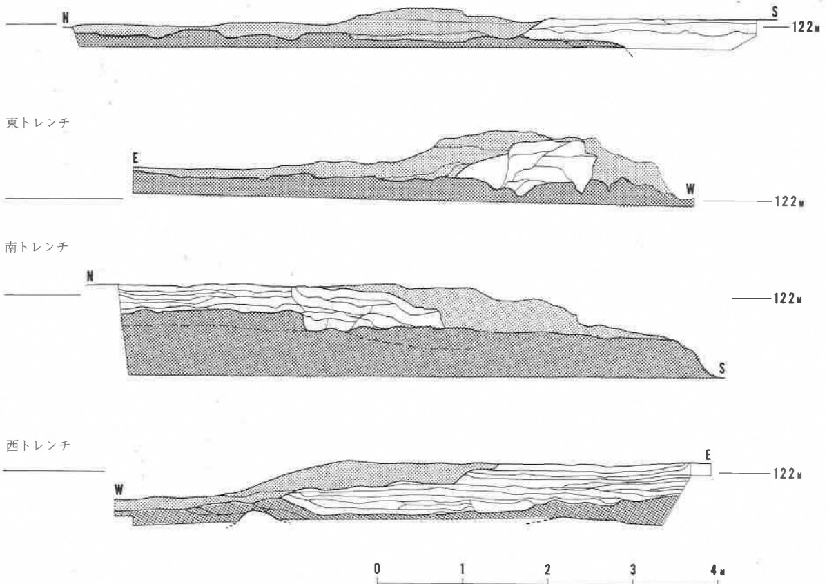
図7 基壇断面土層実測図(白ヌキが版築部分)
