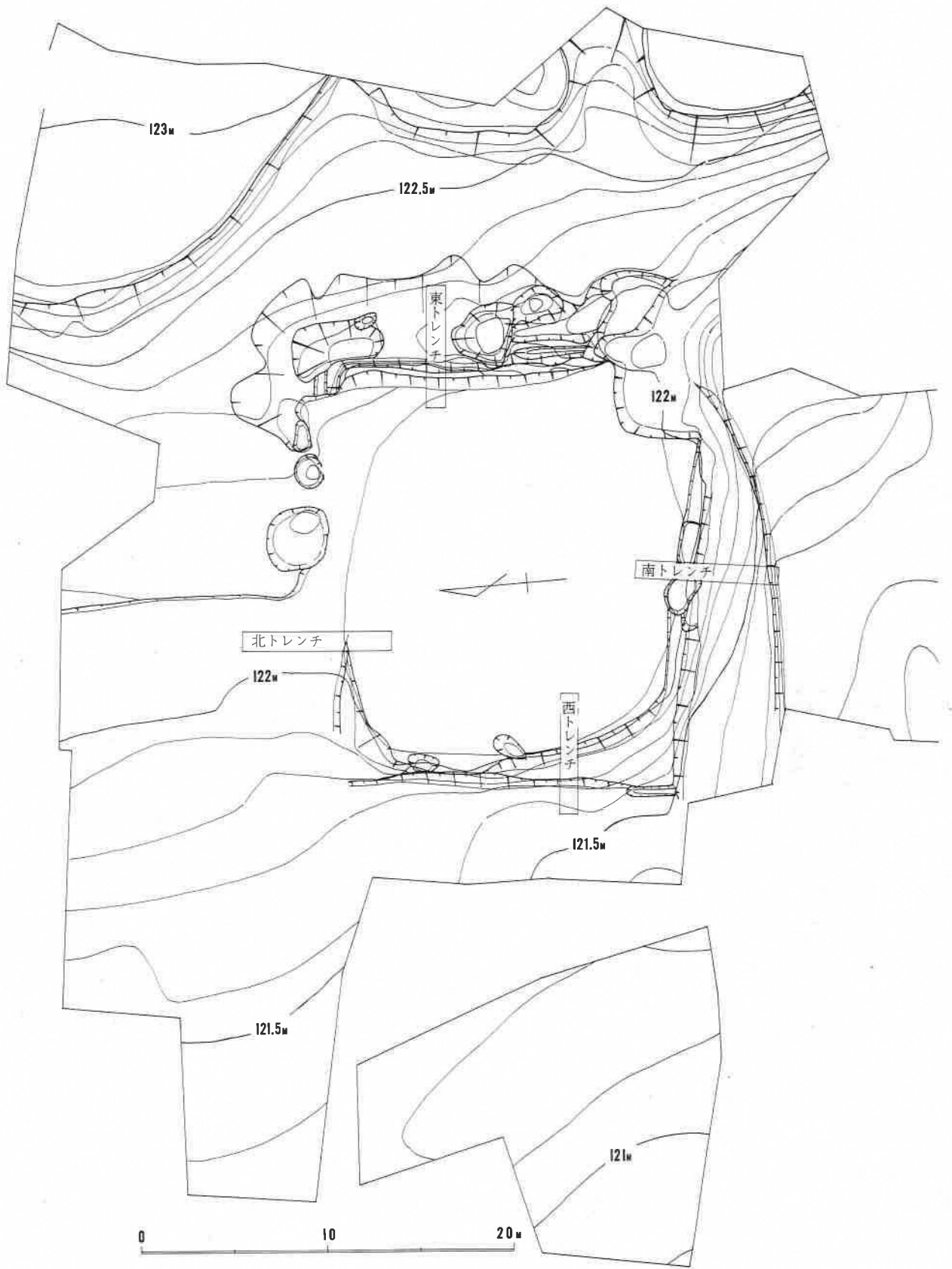
図6 基壇跡測量図
