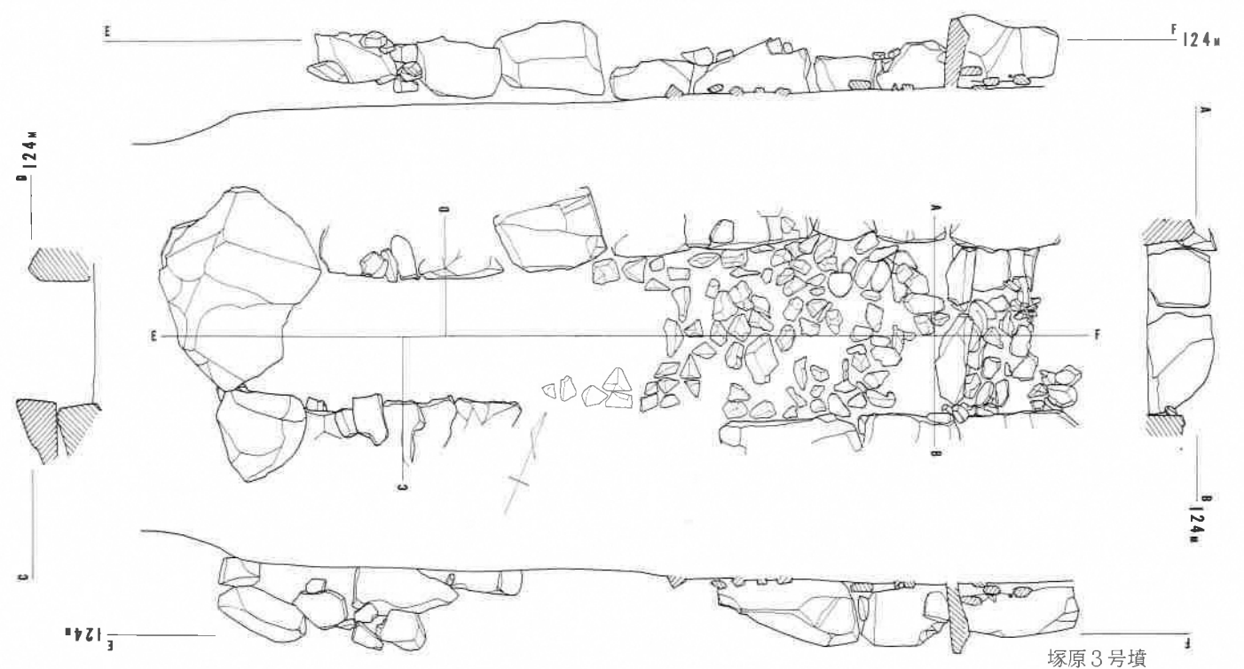
图4 塚原2号·3号墳石室实测图
