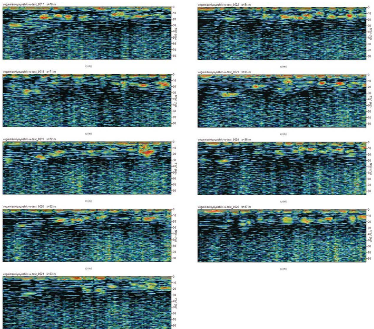
第 87 図 金沢城数寄屋敷西堀縁石垣 GPR 探査成果 (Profile-2)
