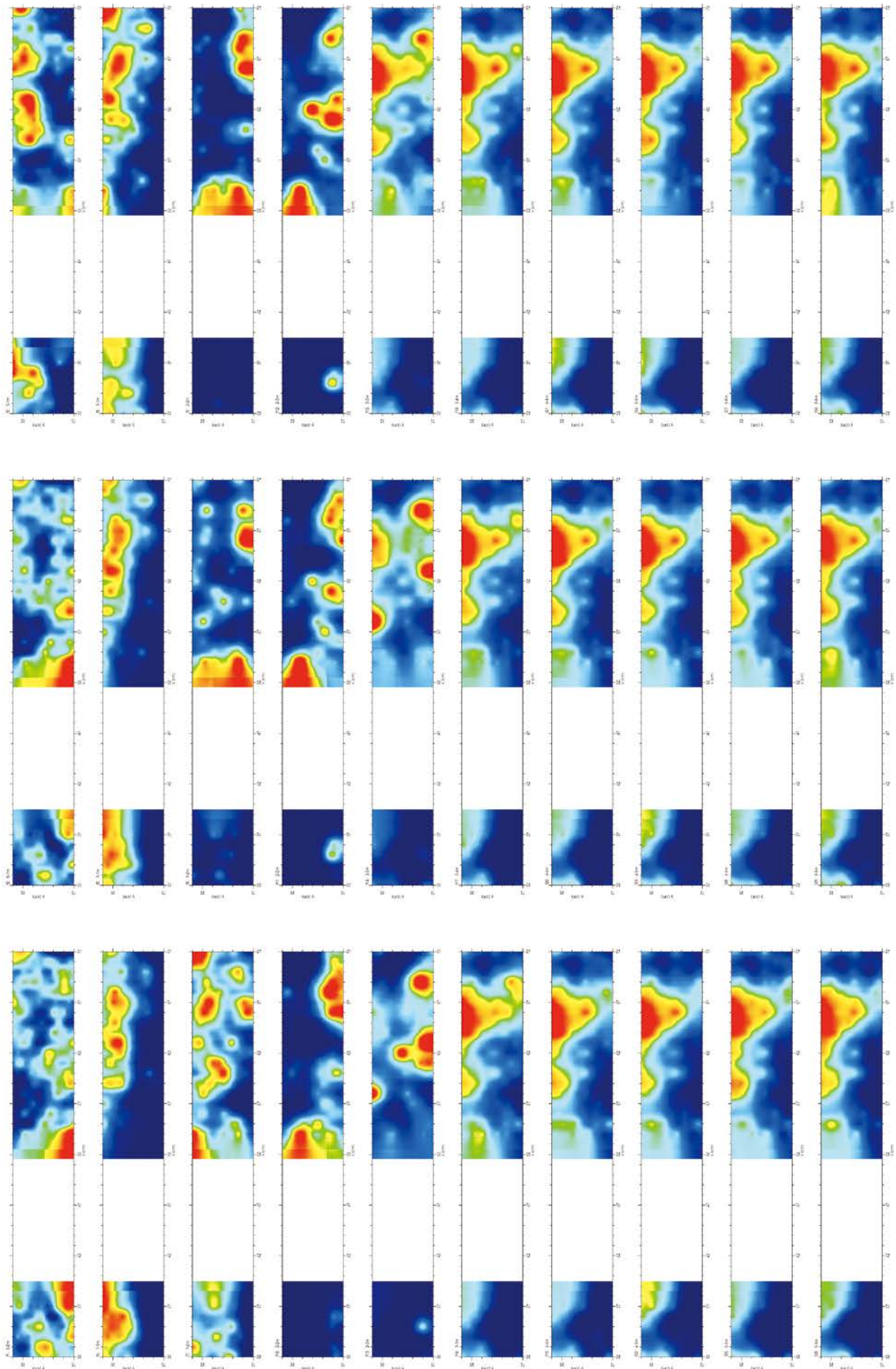
第 85 図 金沢城数寄屋敷西堀縁石垣 GPR 成果 (Time-Slice)
