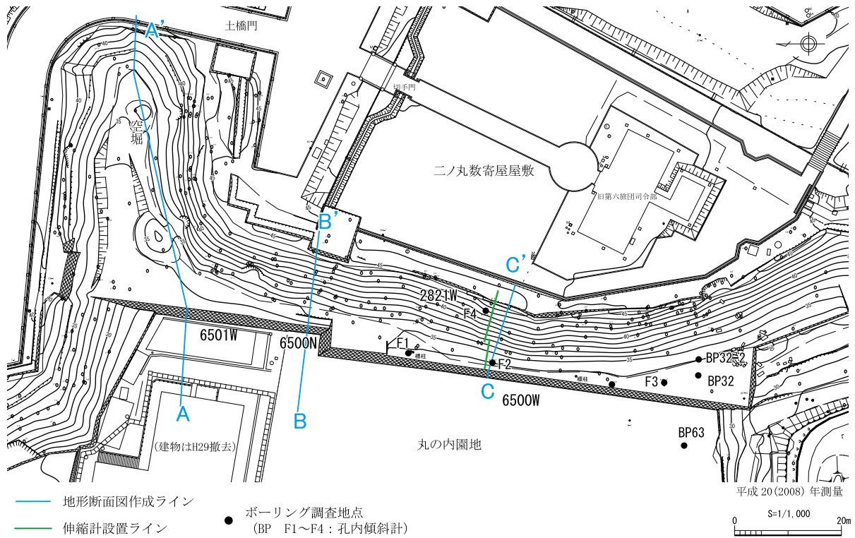
現況平面図
