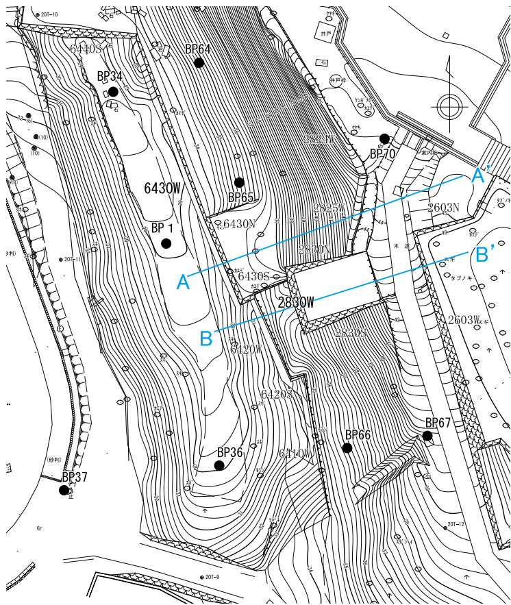
現況平面図
