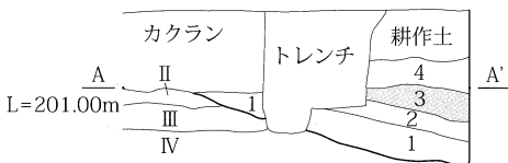
第5図 周堀北側立ち上がり断面図
