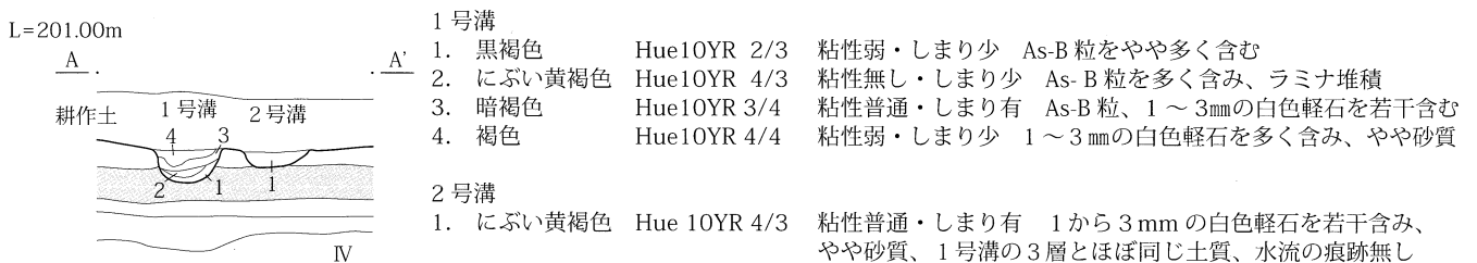
第4図 1・2号溝断面図
