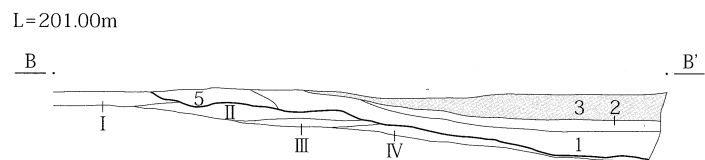
第6図 周堀ベルト断面図
