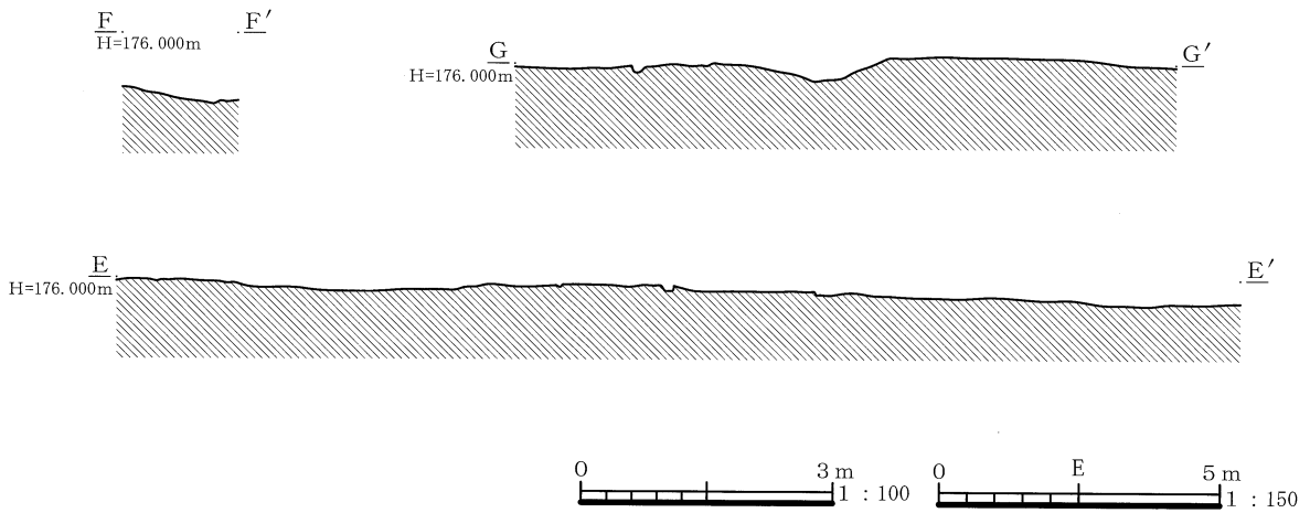
第6図 水田跡②
