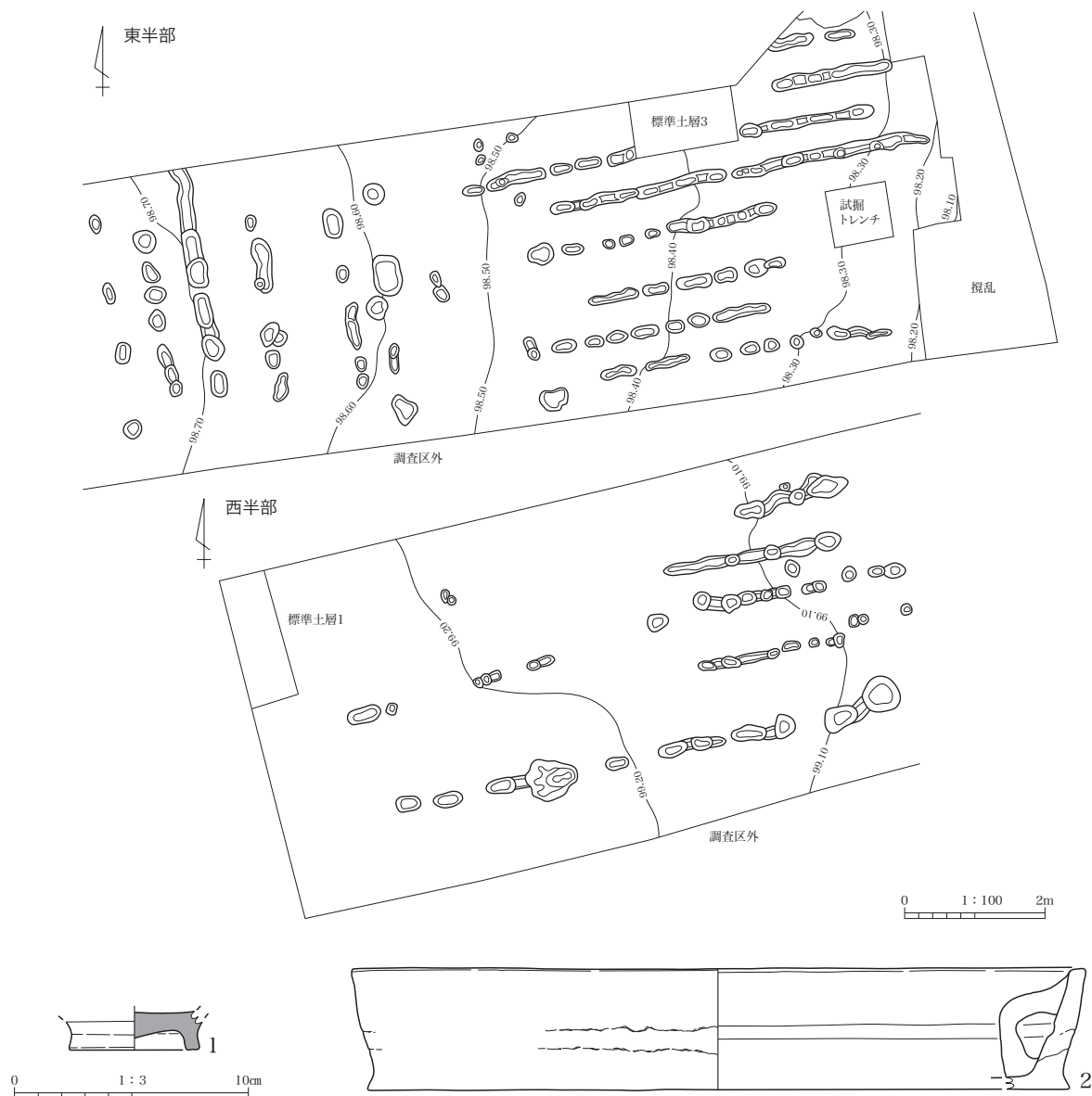
第11図 SY01平面図・出土遺物図
