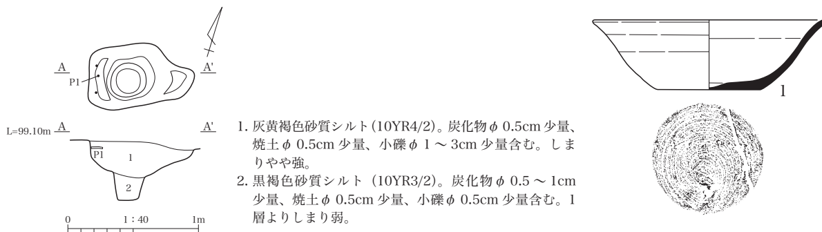
第9図 SK01 平・断面図・出土遺物図
