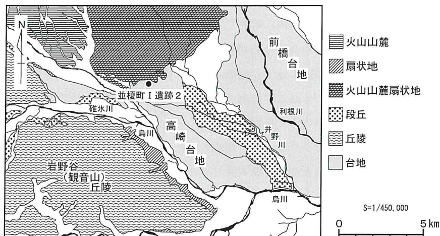
第 2 図 遺跡周辺の地形区分図
