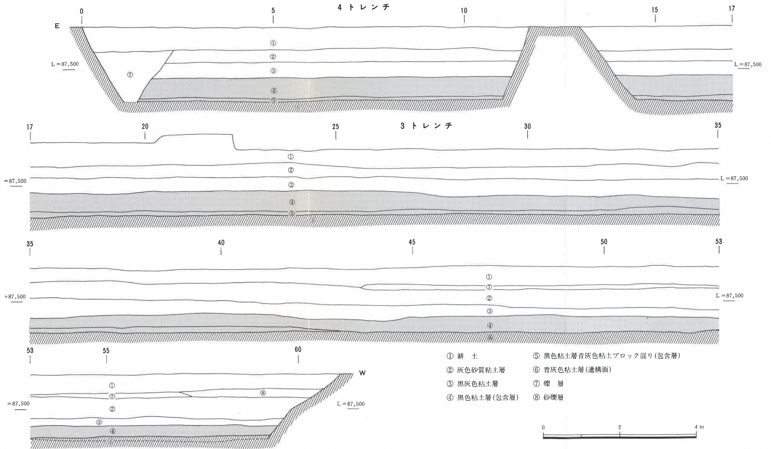
fig7. 3,4トレンチ南壁土層断面図
