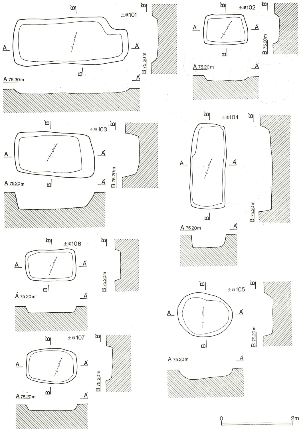
第183图 第101~107号土坑
