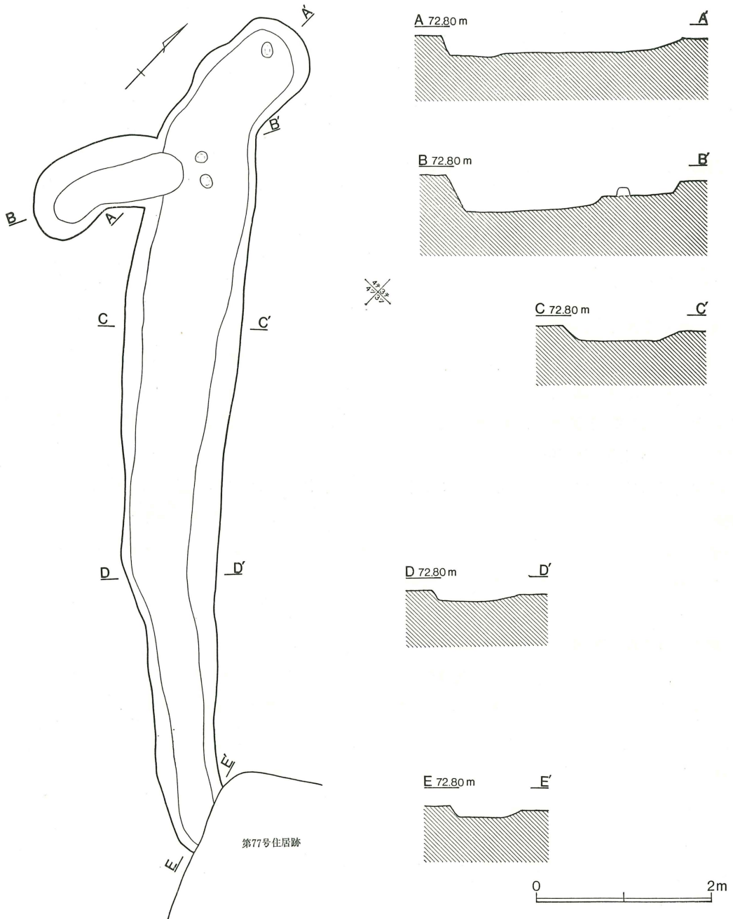
第188図 第1号溝状遺構
