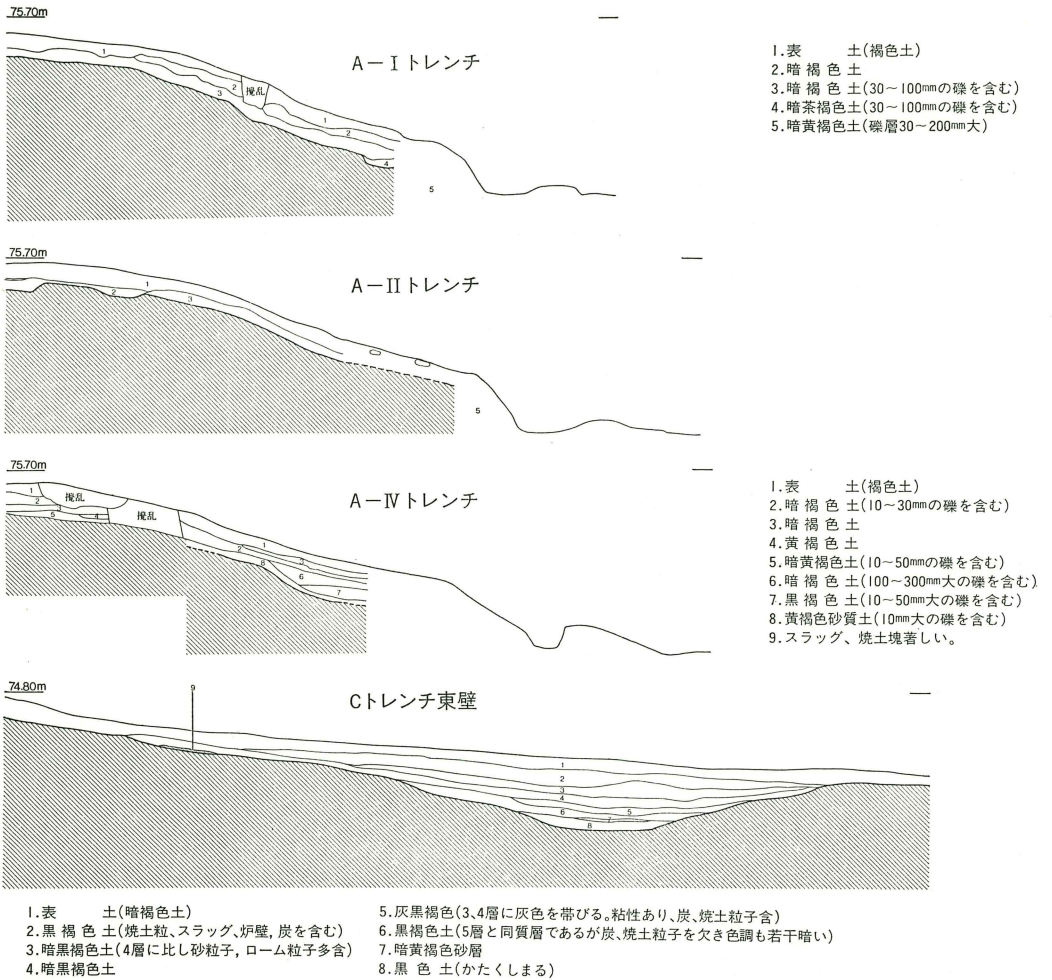
第198図 IV区トレンチ土層図
