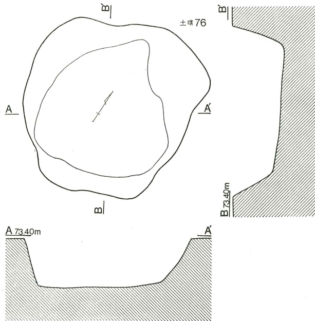
第180图 第71~76号土坑
