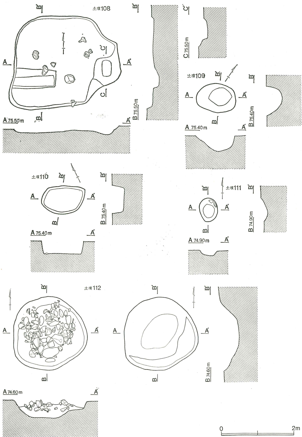
第184图 第108~112号土坑
