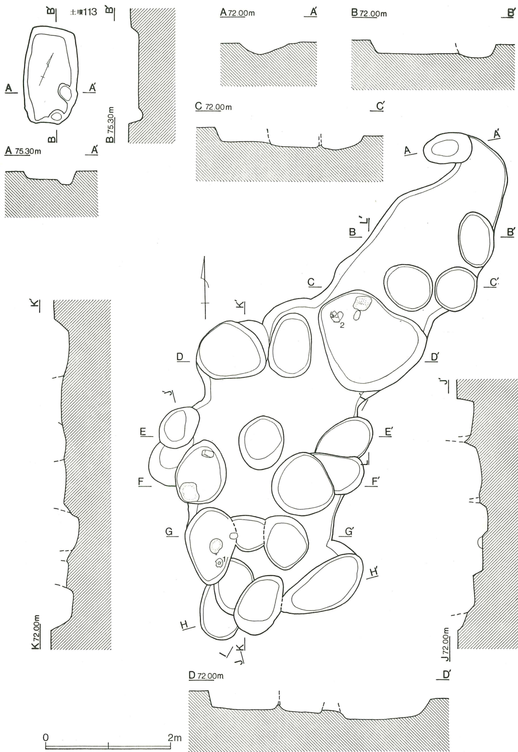
第185图 第113号土坑、土坑群
