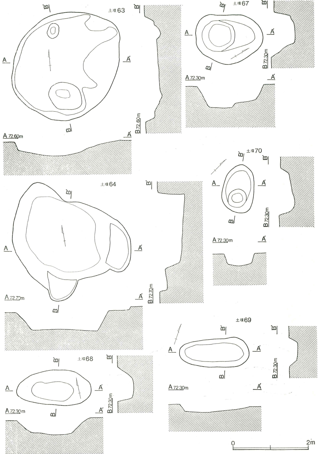
第179图 第63·64·67~70号土坑
