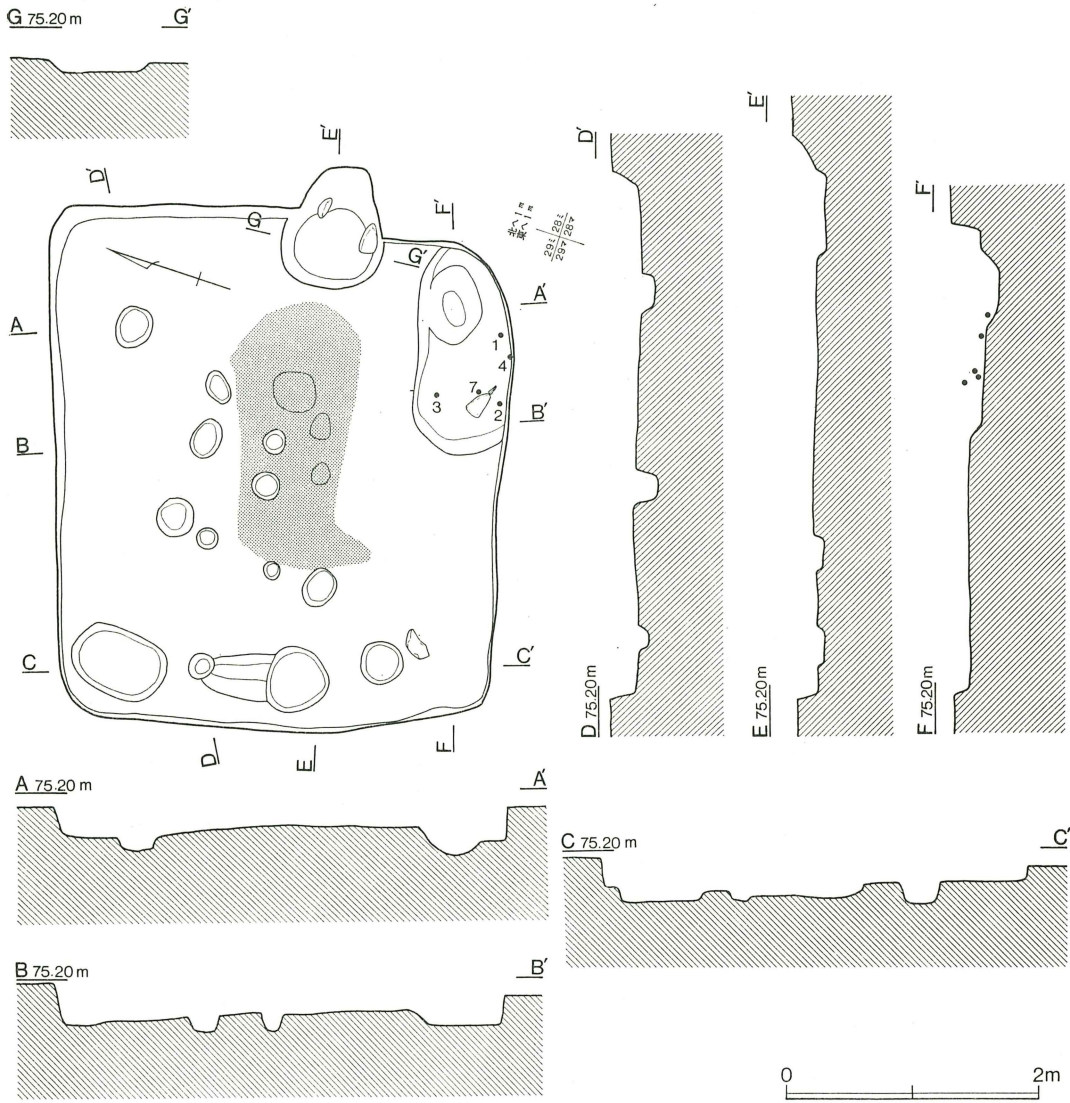
第129図 第79号住居跡
