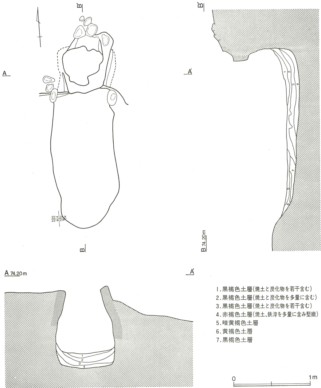
第173図 第3号製錬炉
