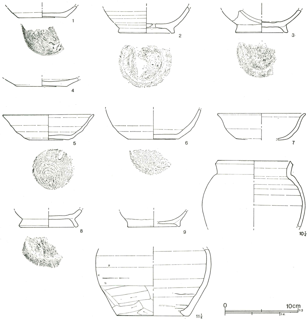
第174図 第3号製錬炉近辺出土遺物
