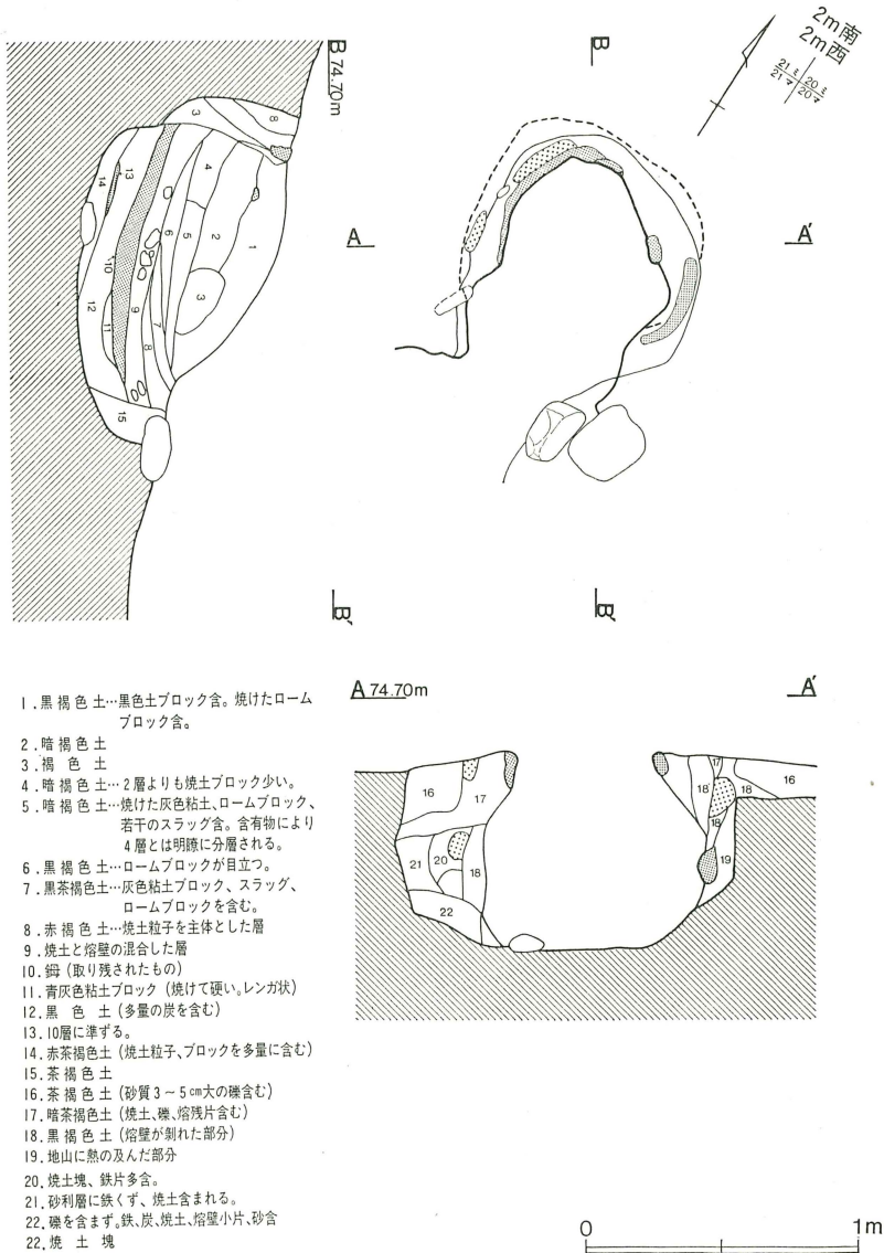
第170図 第1号製鉄炉
