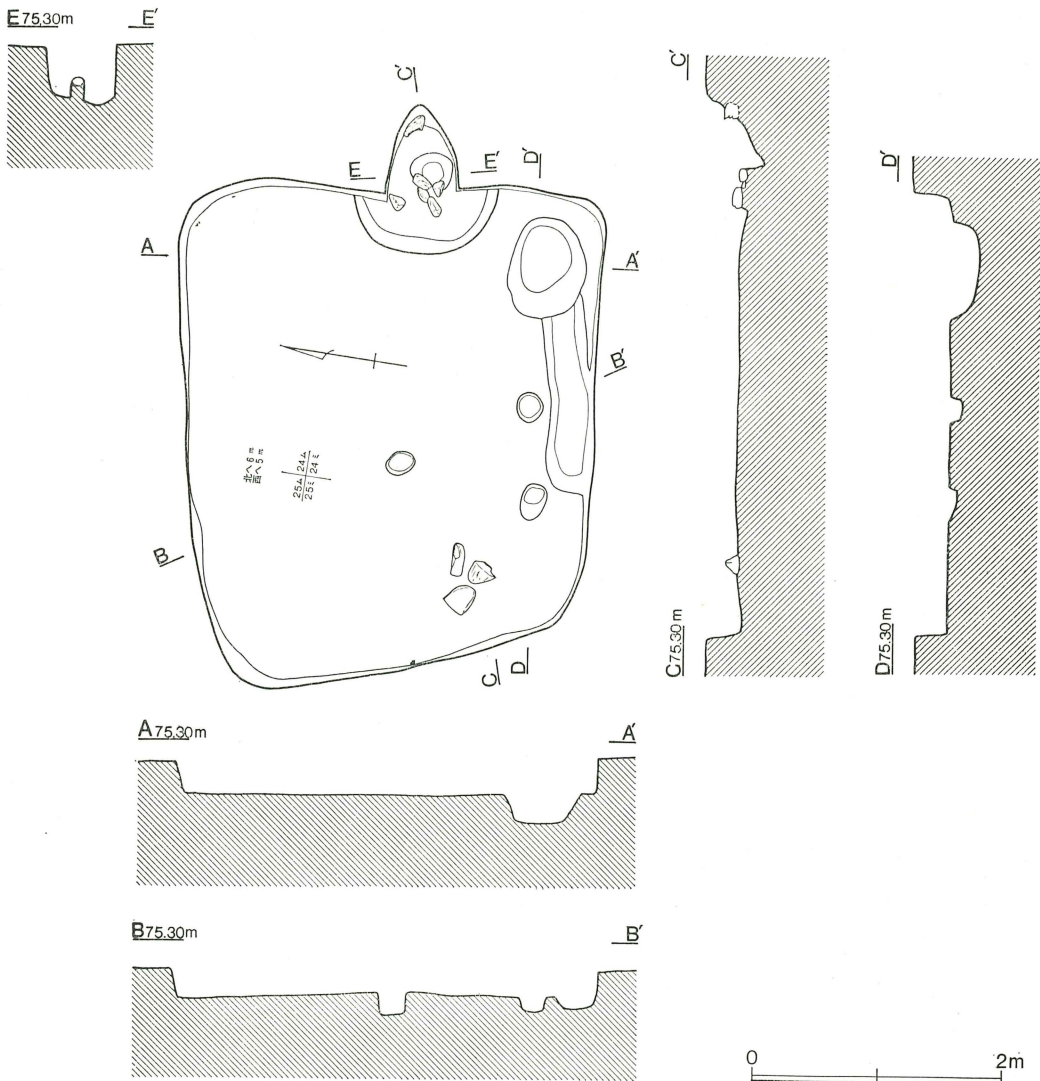
第143図 第86号住居跡
