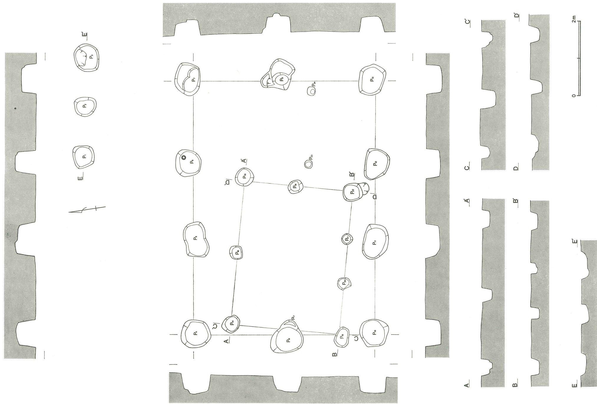
第73図 平原掘立柱建物跡実測図
