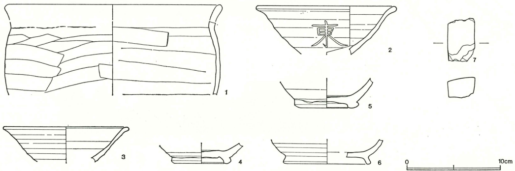
第43図 18号住居跡出土遺物実測図
