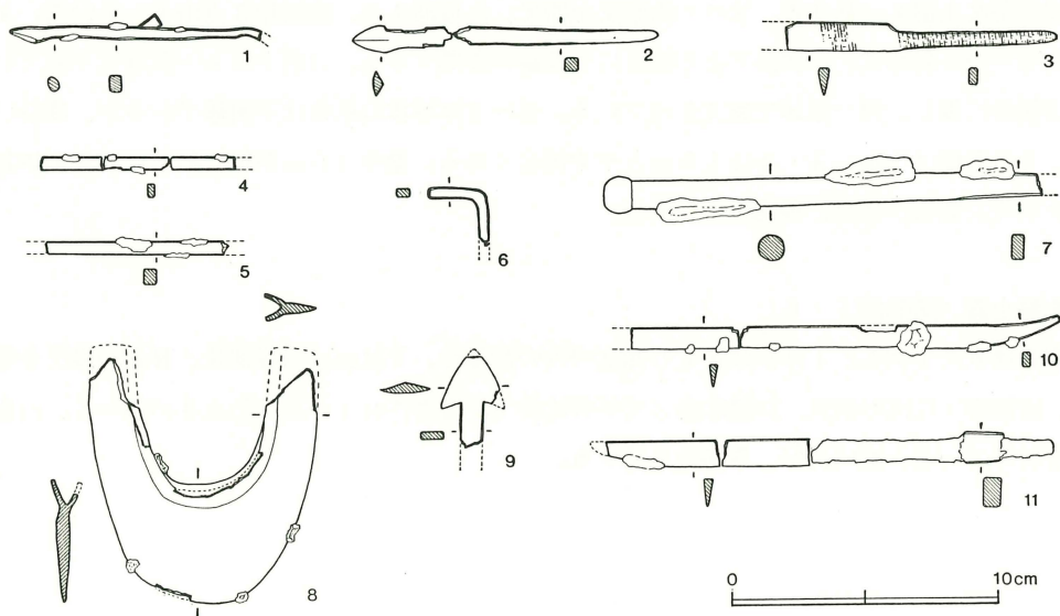
第64図 沼下遺跡出土鉄器実測図
