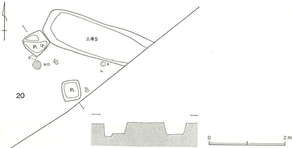
第46図 沼下20号住居跡・5号土塚実測図
