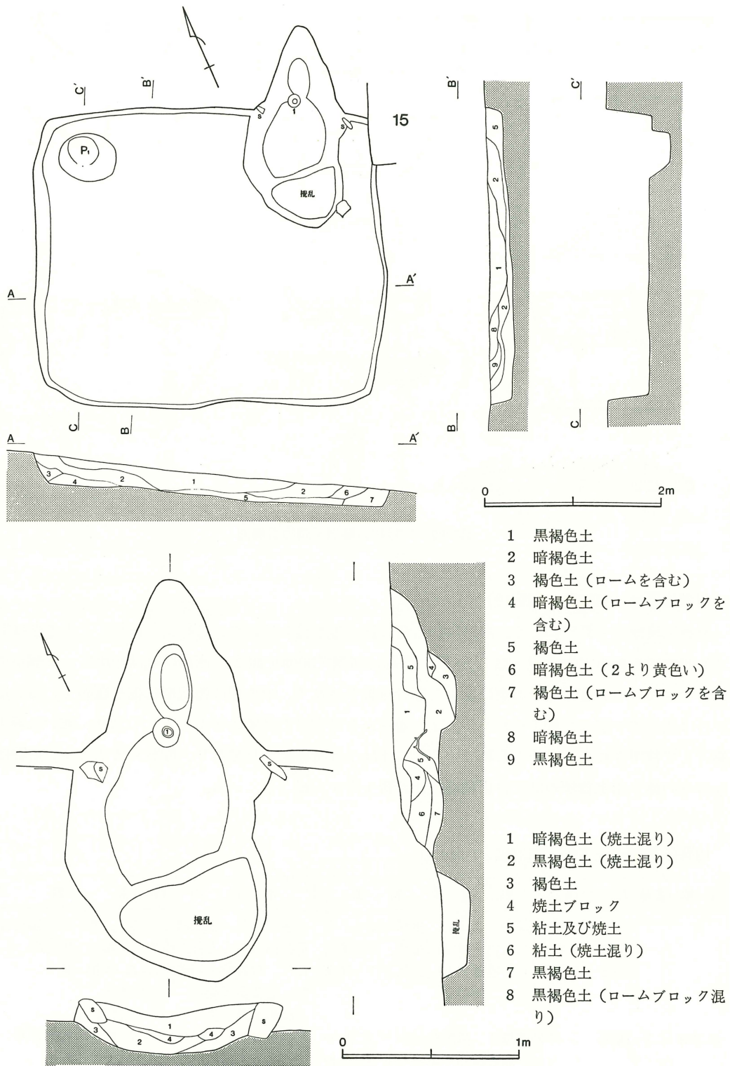
第33図 沼下13号住居跡実測図
