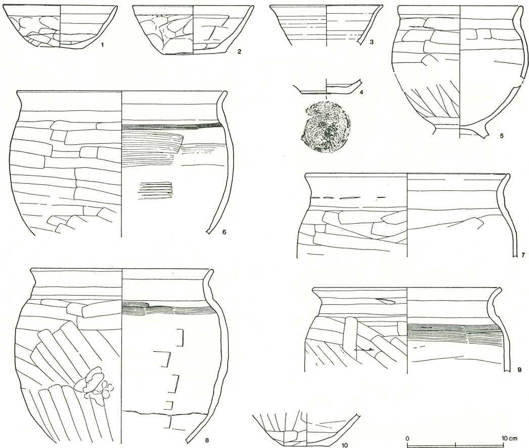
第54図 24号住居跡出土遺物実測図
