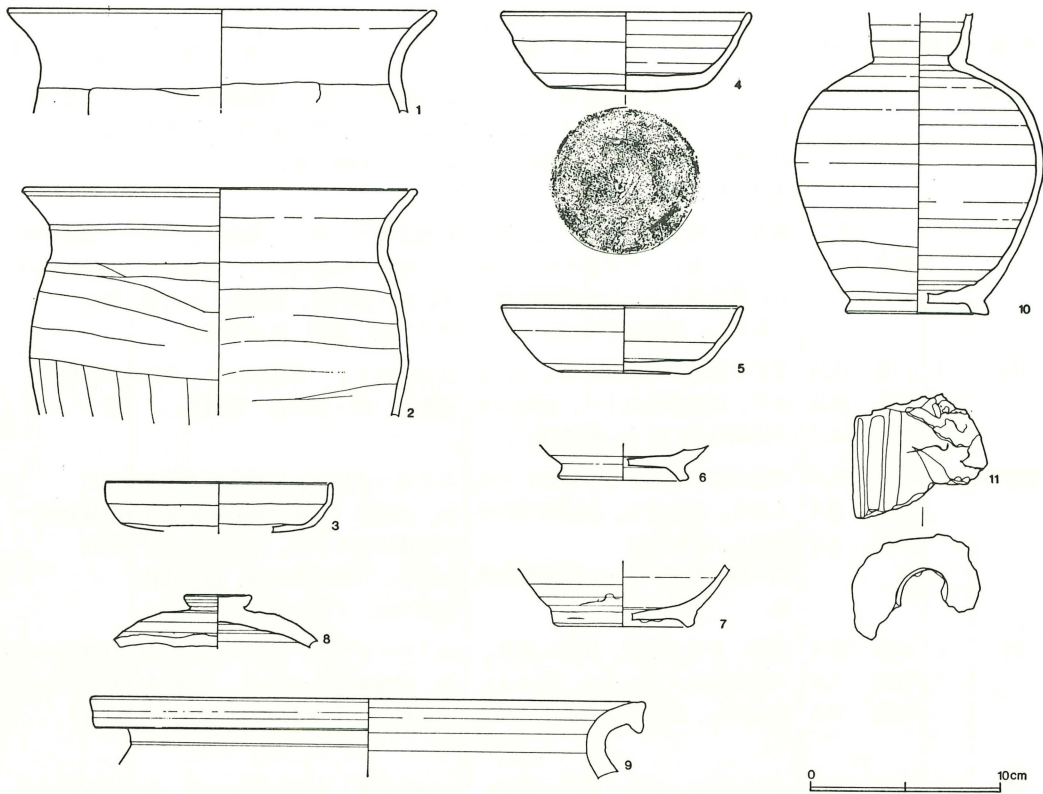
第41図 17号住居跡出土遺物実測図
