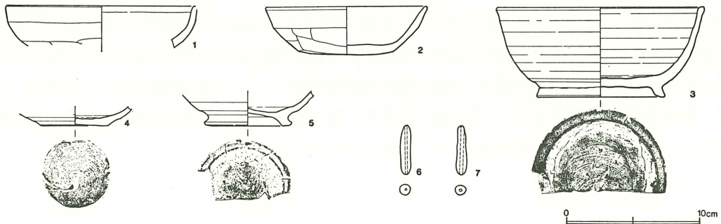
第37図 15号住居跡出土遺物実測図
