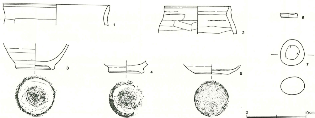
第36図 14号住居跡出土遺物実測図
