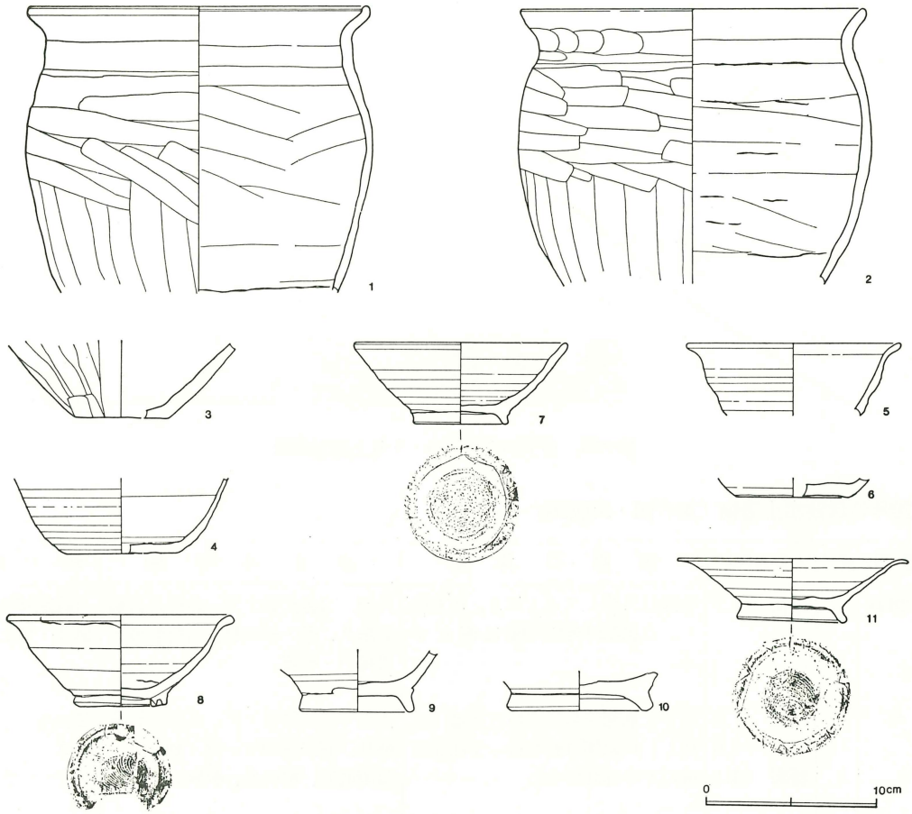
第45図 19号住居跡出土遺物実測図
