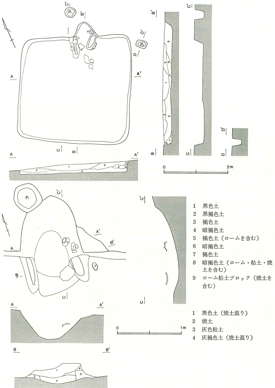
第44図 沼下19号住居跡実測図
