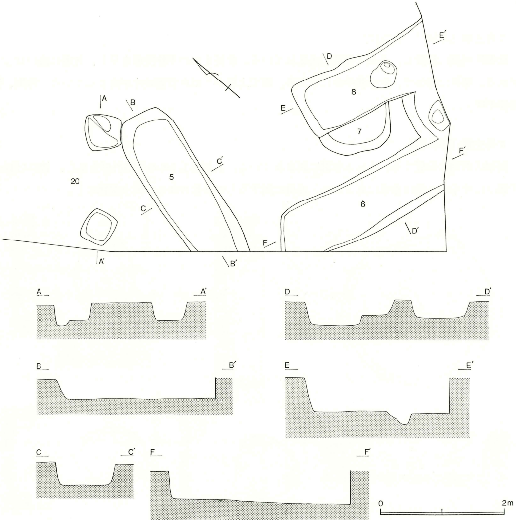
第56図 5・6・7・8号土壇実測図
