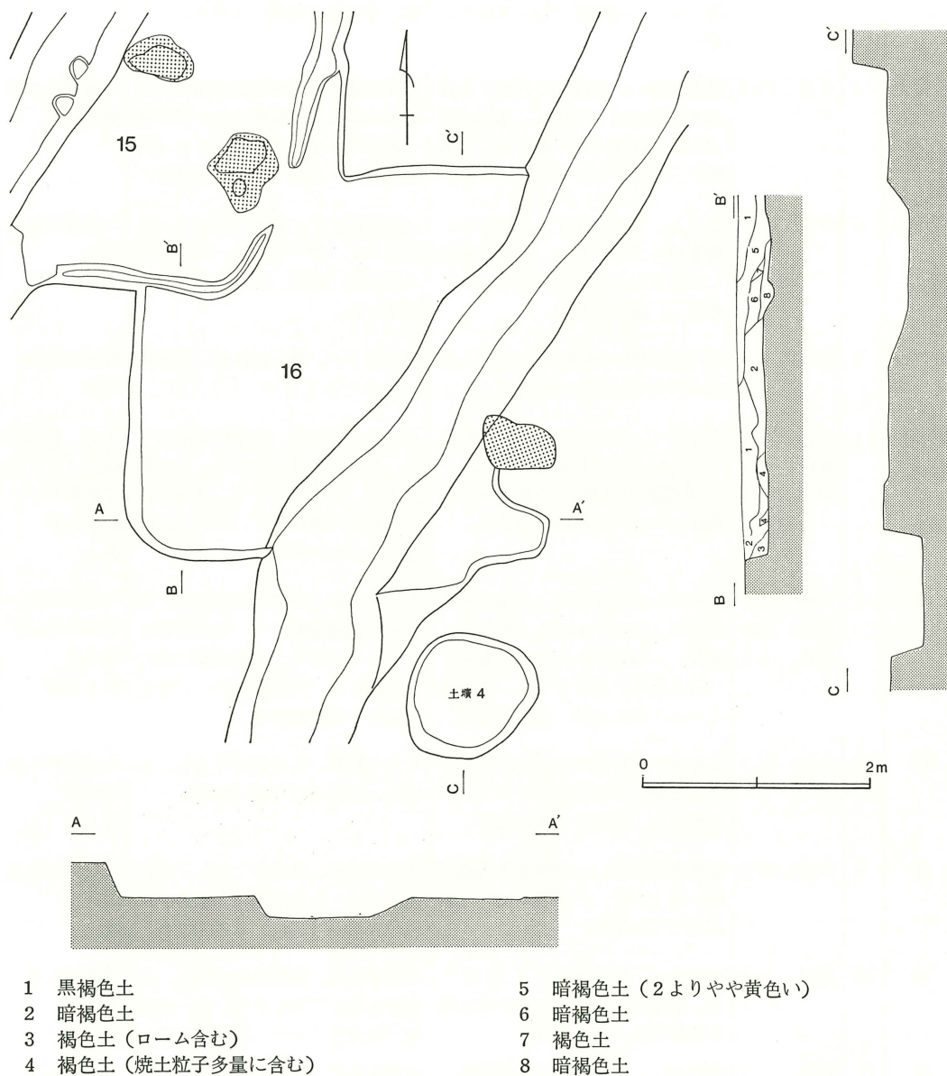
第38図 沼下16号住居跡実測図
