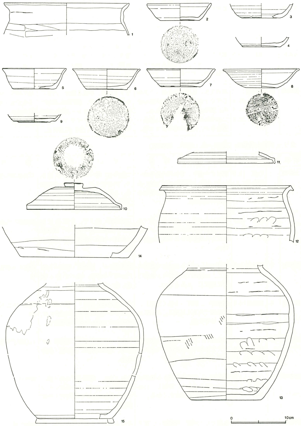
第59図 グリッド出土遺物実測図(1)
