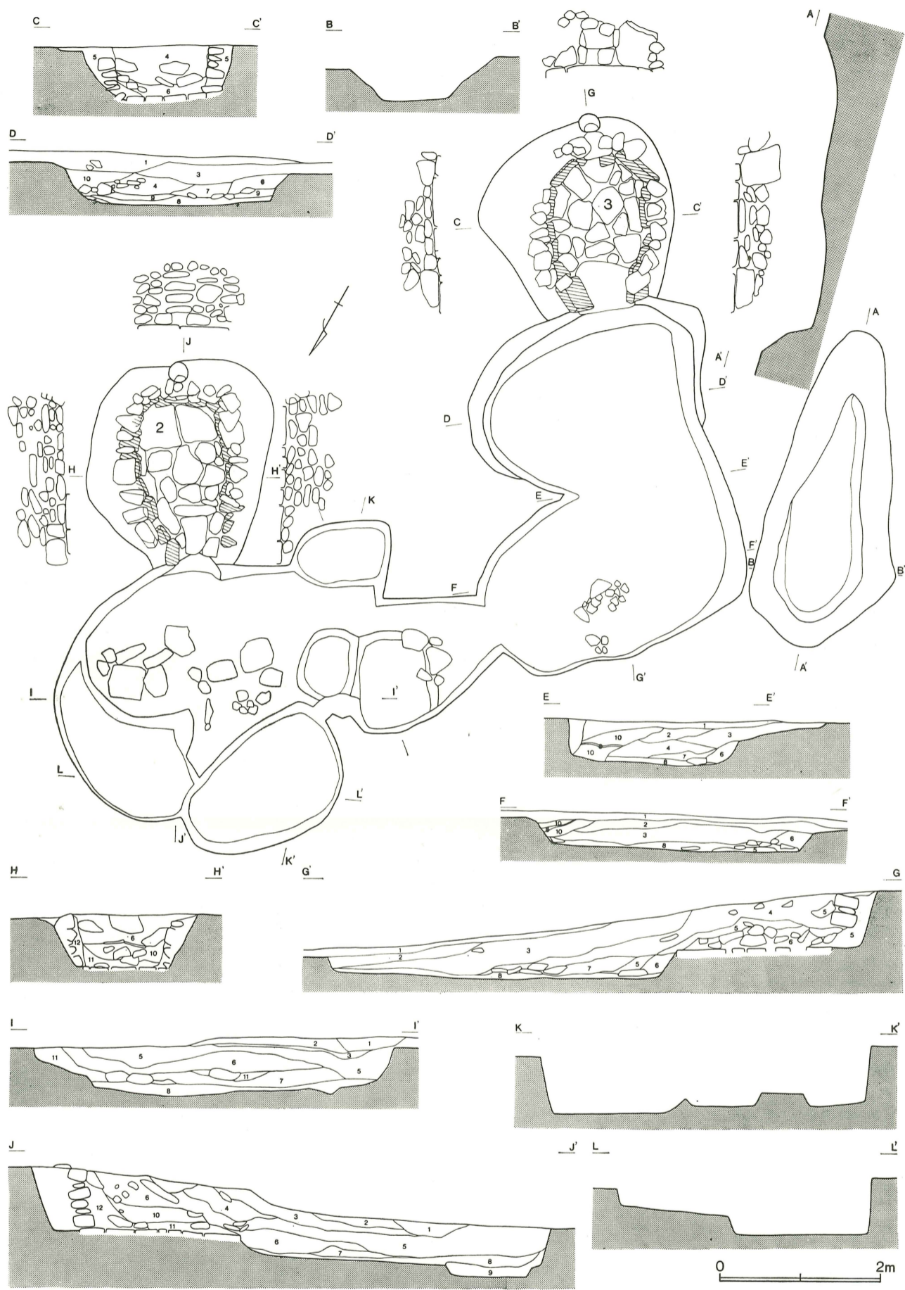
第80図 中山遺跡 2・3号炭焼窯実測図
