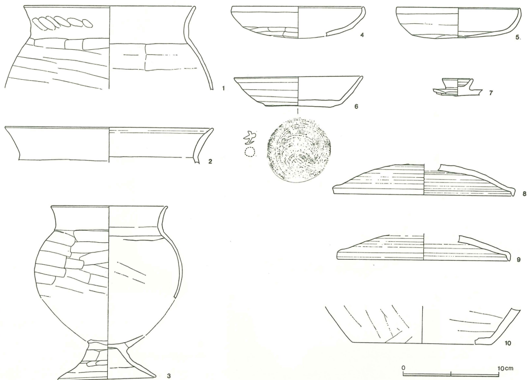
第71図 3号住居跡出土遺物実測図
