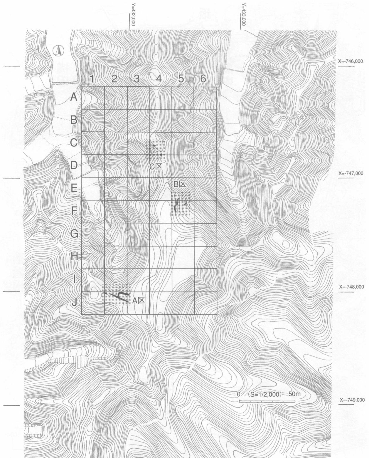
第2図 グリッド配置図
