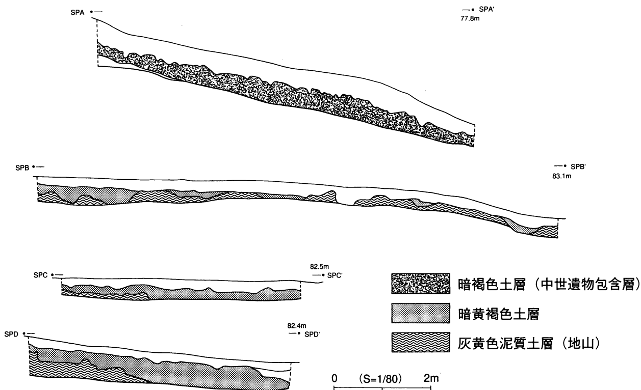
第7図 5～8トレンチセクション図
