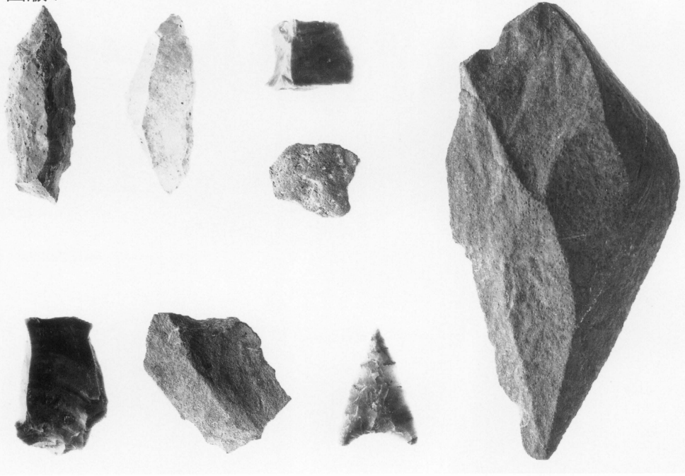
1. 出土石器
