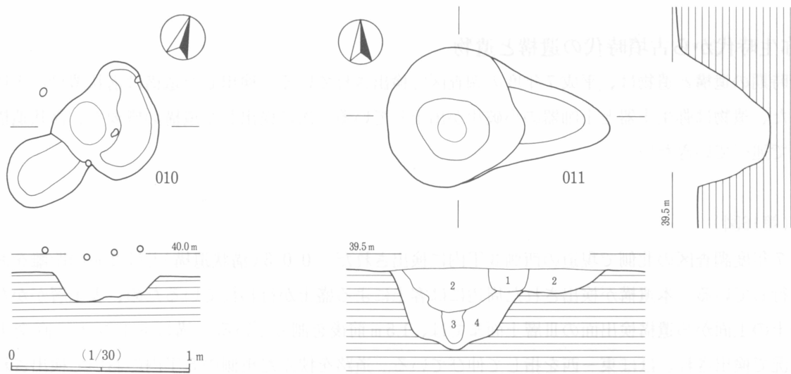
第14図 010・011土坑
