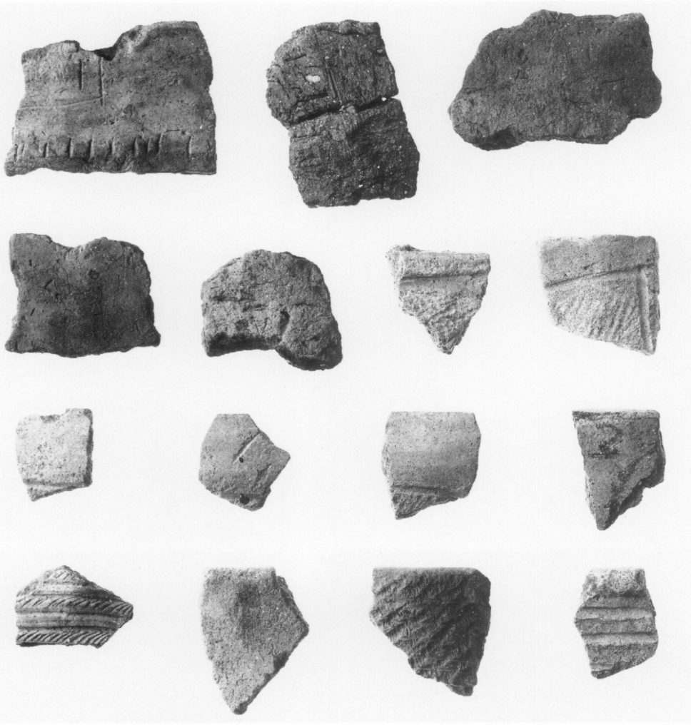
2. 繩文土器
