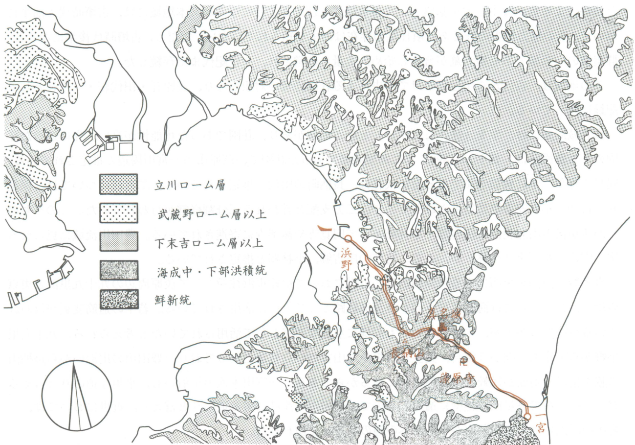
第1図 千葉県中央部地質図
