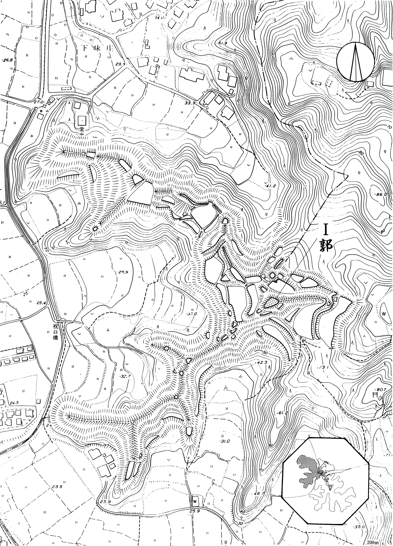
第7図 真名城 I 郭周辺概念図
