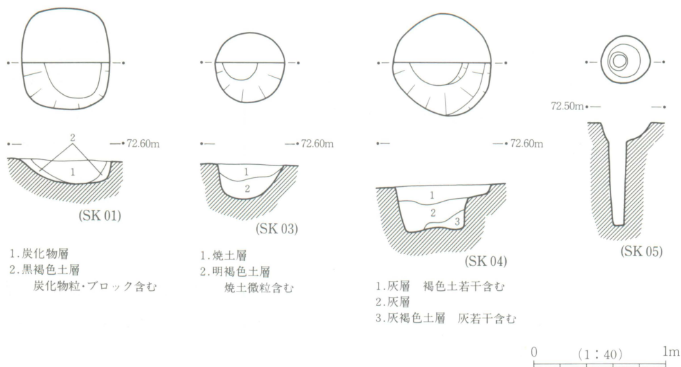
fig. I-4 土坑・柱穴平面図，土層断面図
