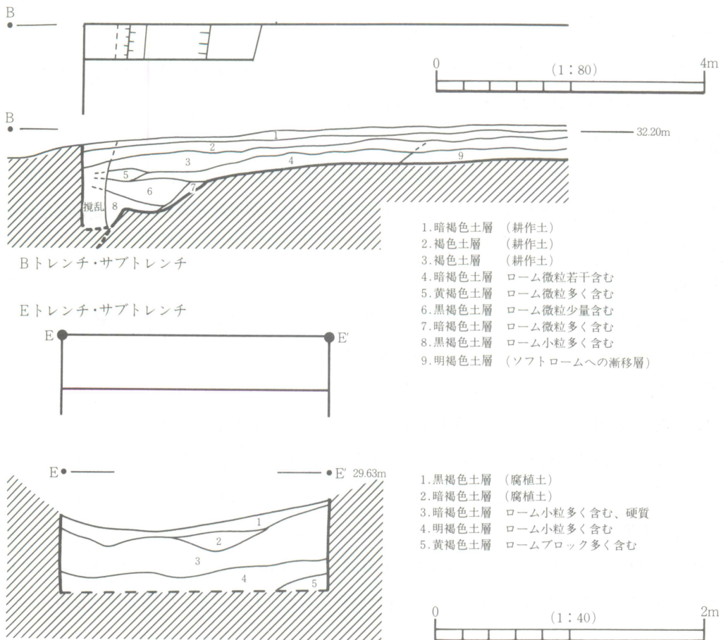
fig.II-10 サブトレンチ平面図・断面図
