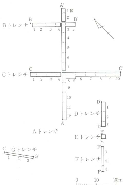
fig.II-8 トレンチ配置図
