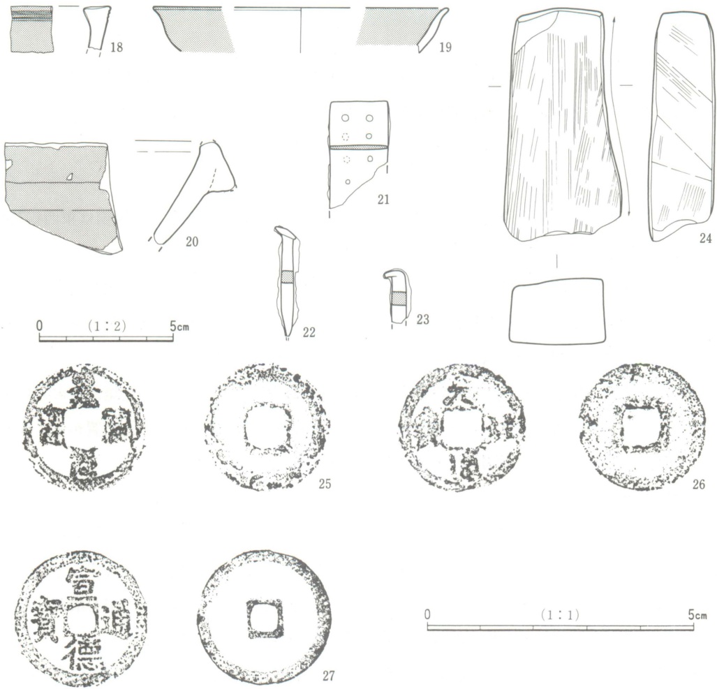
fig. I-6 出土遺物実測図(2)
