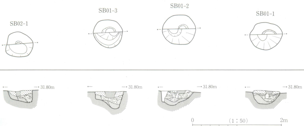
断面図
