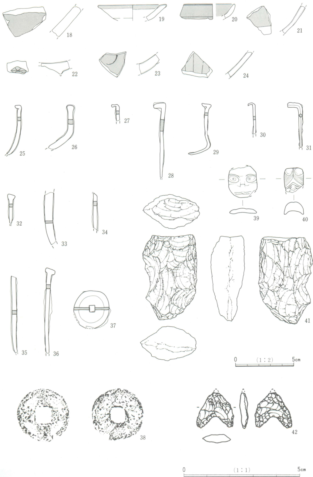
fig.II-12 出土遺物実測図(2)
