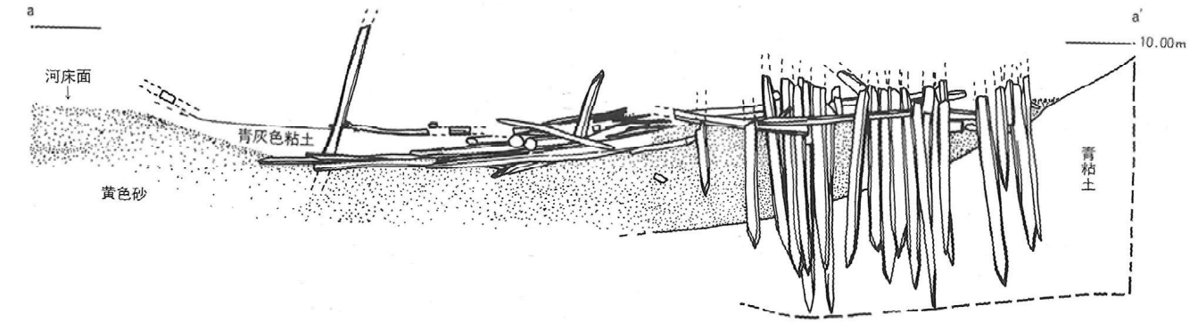
PL. 図-322 テシの杭立面図
