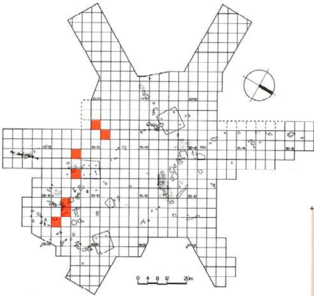
PL. 274 个体番号 坏38の破片分布图
