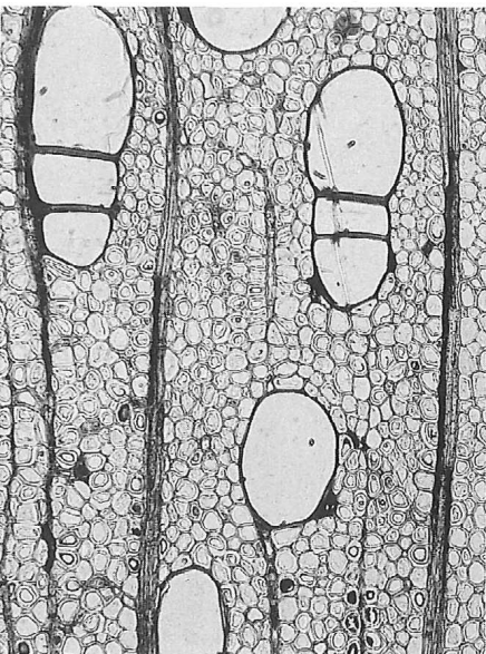
カバノキ属
