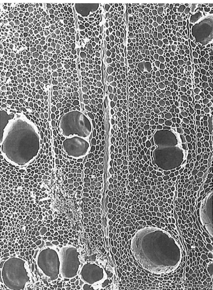
ウルシ属
