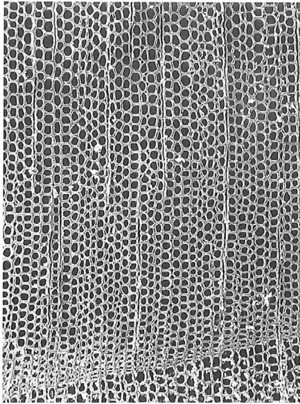
イチイ 1a(×100)
