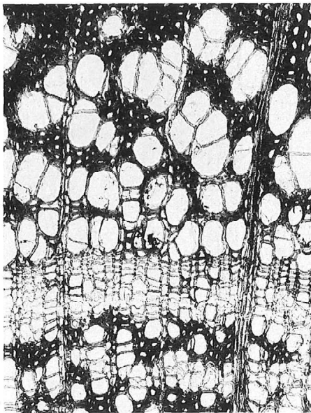
ハシドイ属
