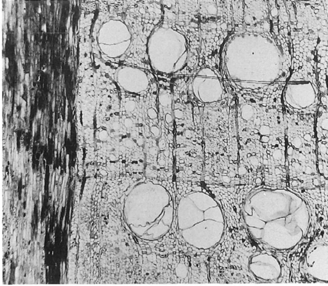
コナラ属
