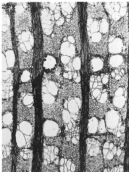
エノキ属
