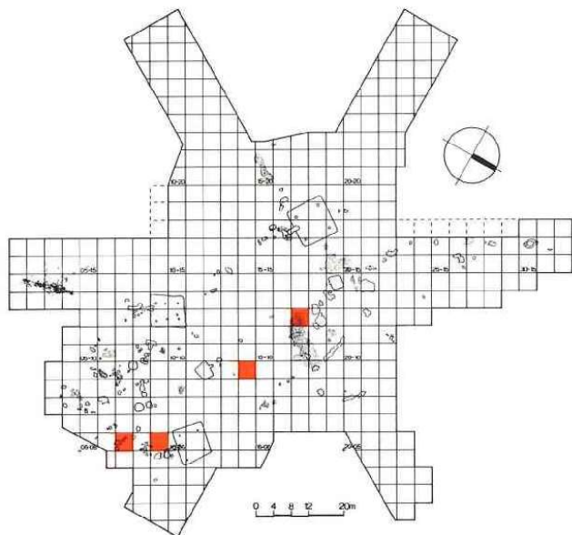
PL. 図-233 個体番号環62の破片分布図
