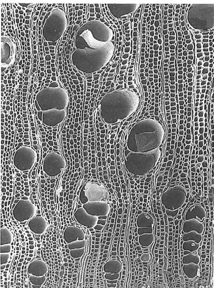
アサダ
