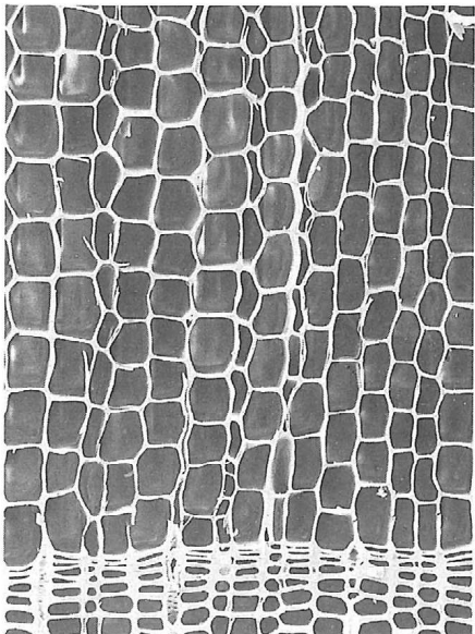
モミ属 2a(×230)
