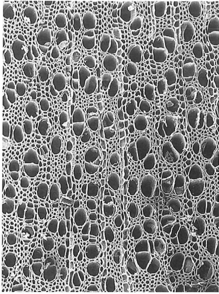
ニワトコ属
