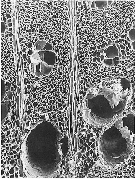
クワ属 7a(140)
