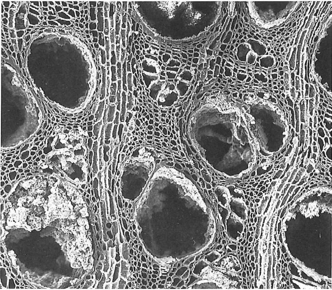
ツル性植物
