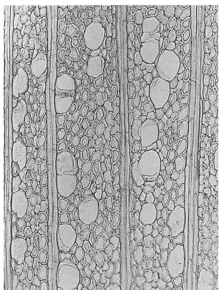
モクレン属
