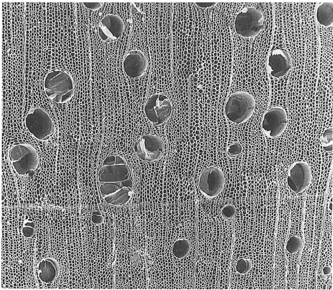
オニグルミ
