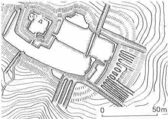
①村岡山城跡 (中井 均 作図)
