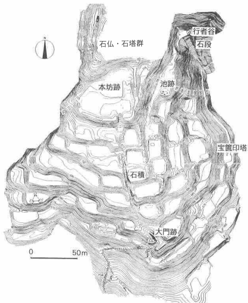
第2図 弥高寺跡平面図
