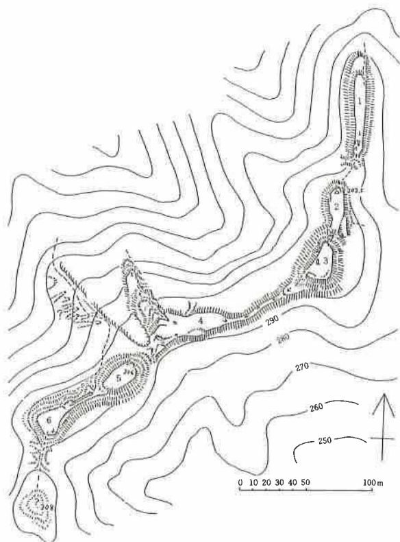
第7図 勝楽寺城跡縄張り図
