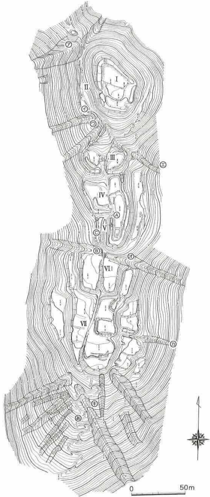
第4図 上平寺城跡測量図
