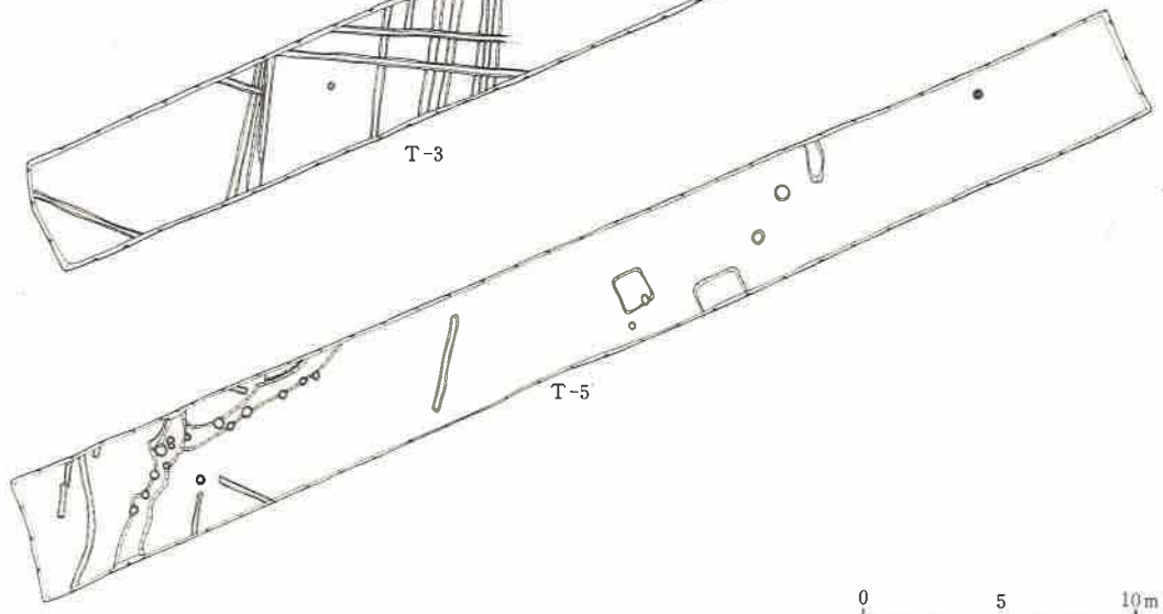
T-1 ~ 5 トレンチ遺構図
