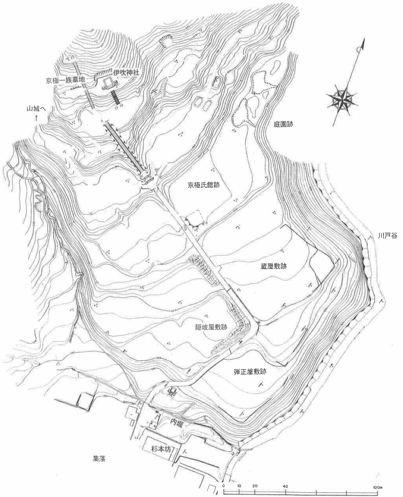
第2図 上平寺館跡平面図
