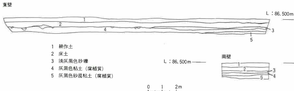
第9図 C地区土層断面図
