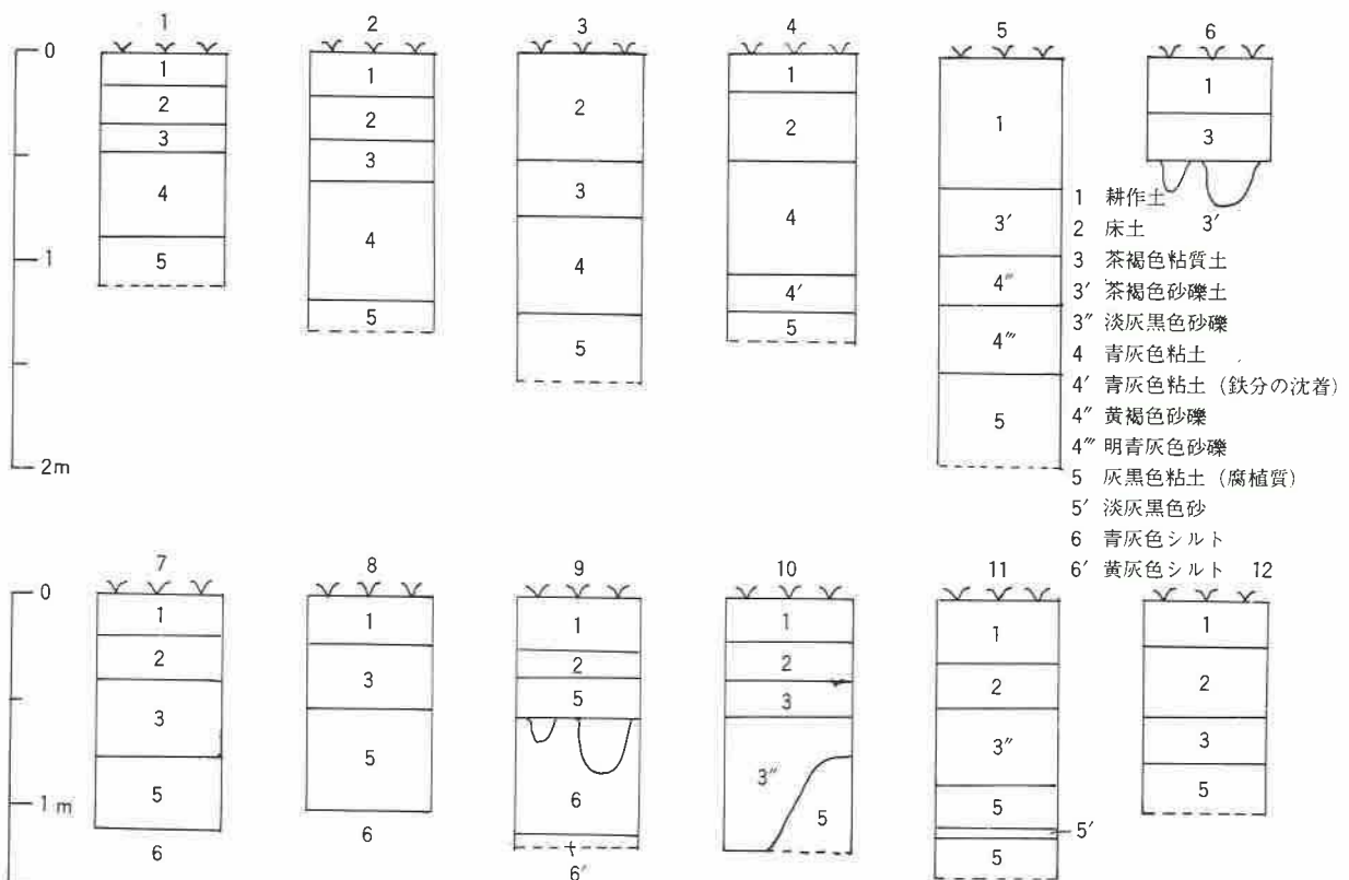
第3図 土層柱状図
