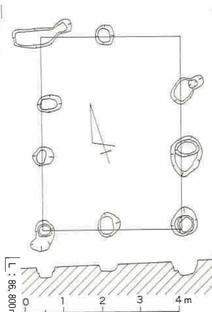
第6図 A地区SB-1平面図
