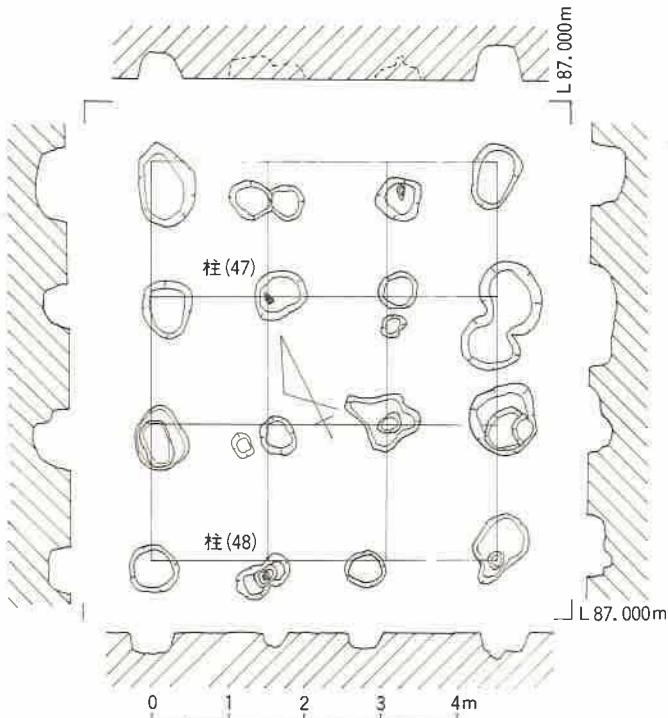
第7図 A地区SB-2平面図
