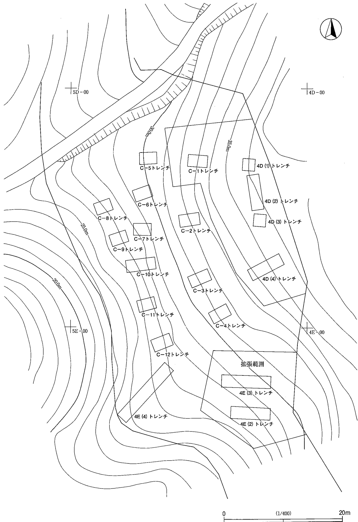
第9図 C区 トレンチ配置図、地形測量図
