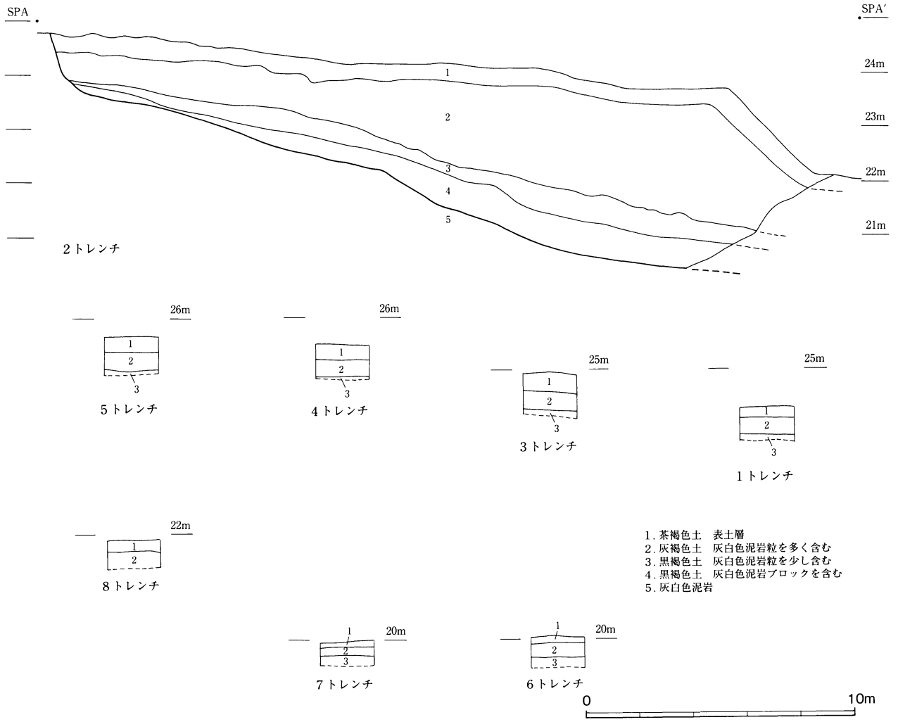
第4図 土層断面図・土層柱状図 (1/100)
