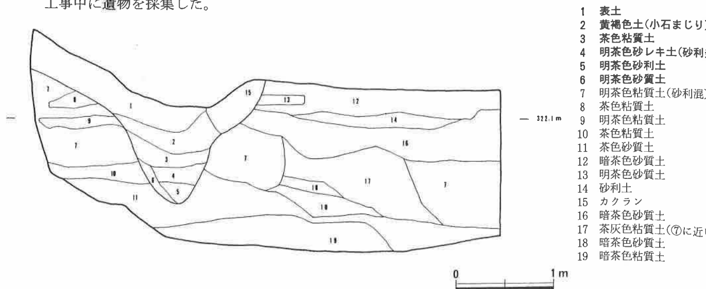
第9図 ST3断面図
