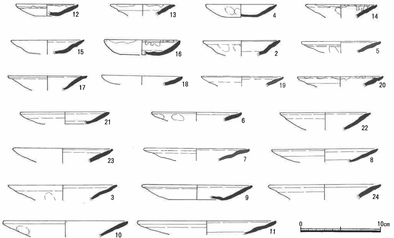
第12図 T1出土遺物実測図
