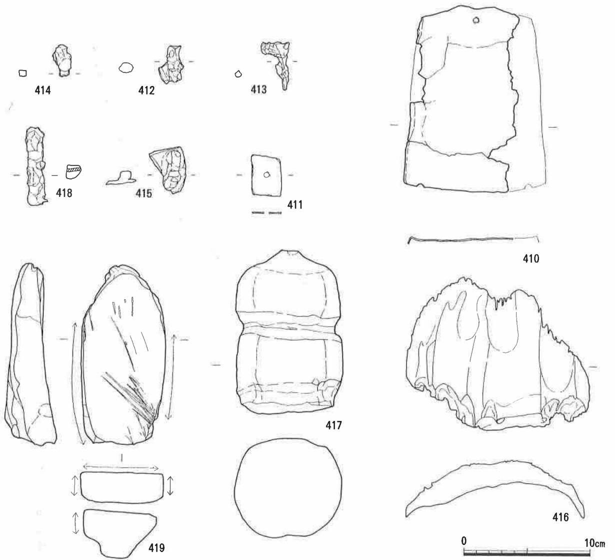
第36図 金属製品・石製品・木製品実測図
