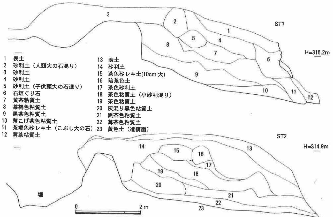
第 23 図 ST1・ST2 断面図
