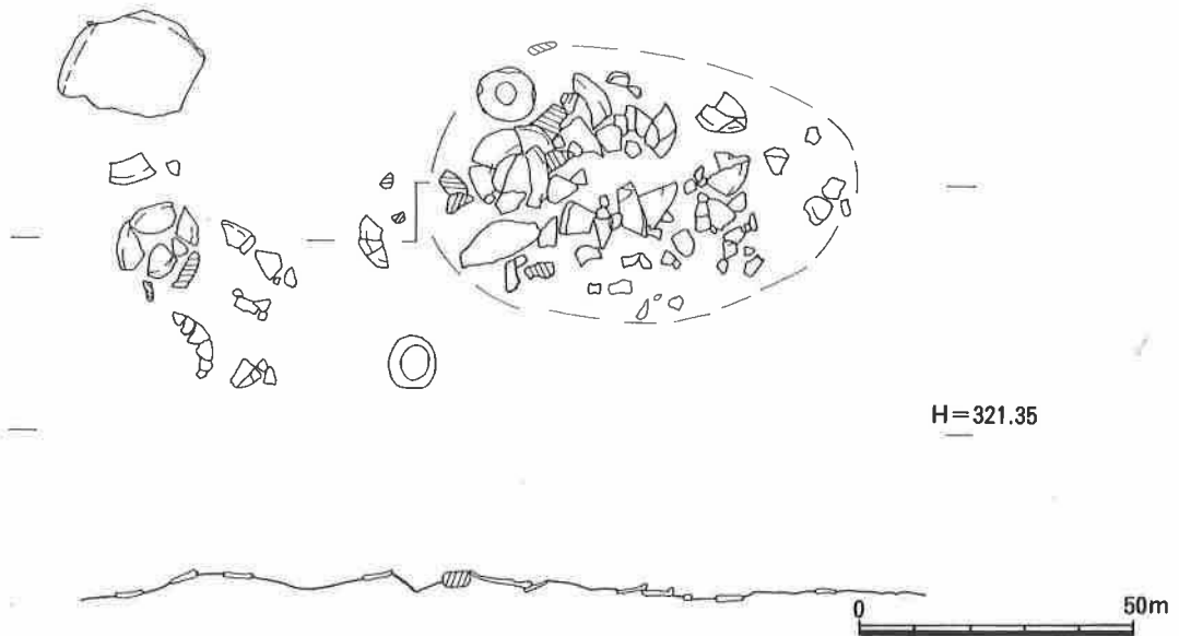
第 27 図 土師皿一括投棄遺構 2 実測図
