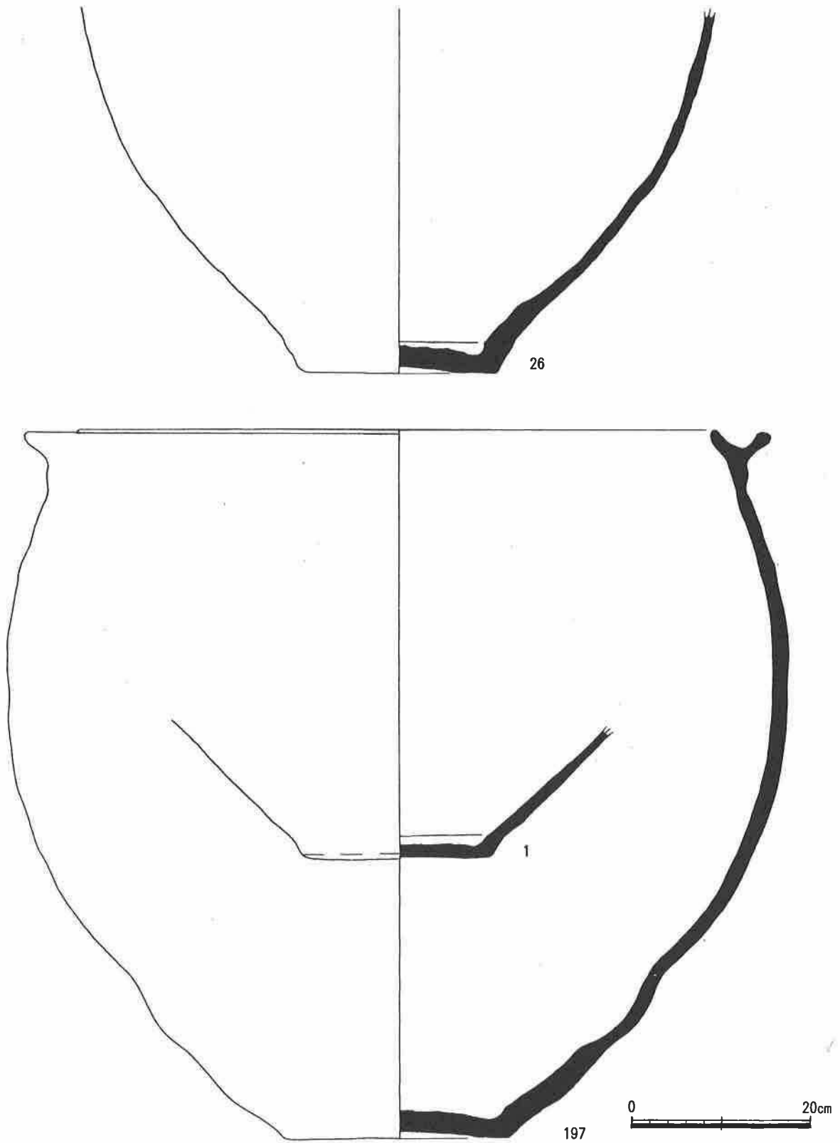
第 35 图 近世陶器实测图
