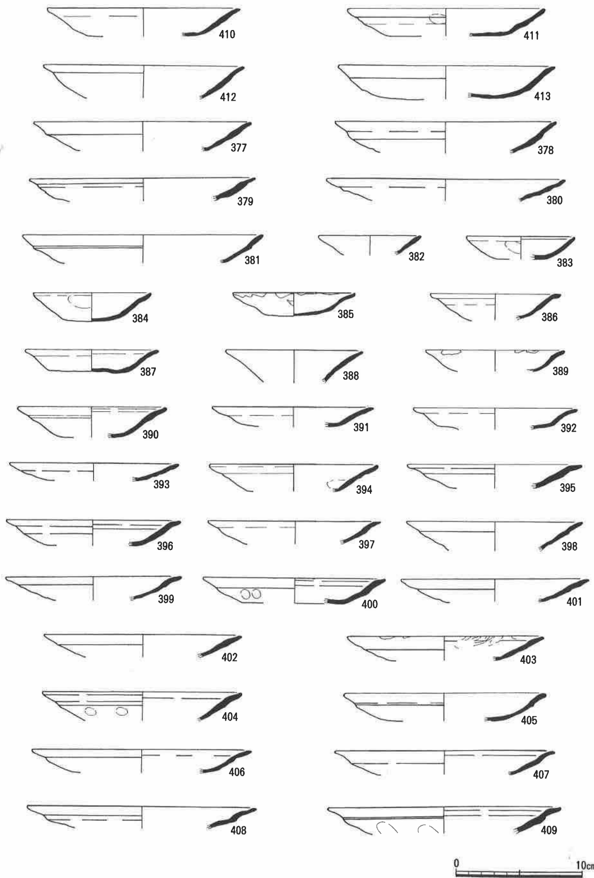
第 34 图 T5 出土遺物実測図 (6)
