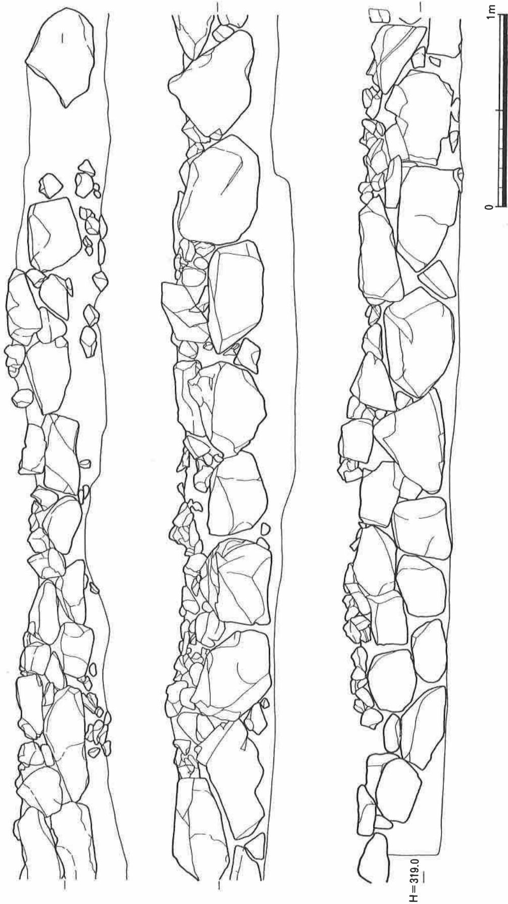
第 14 图 石垣实测图
