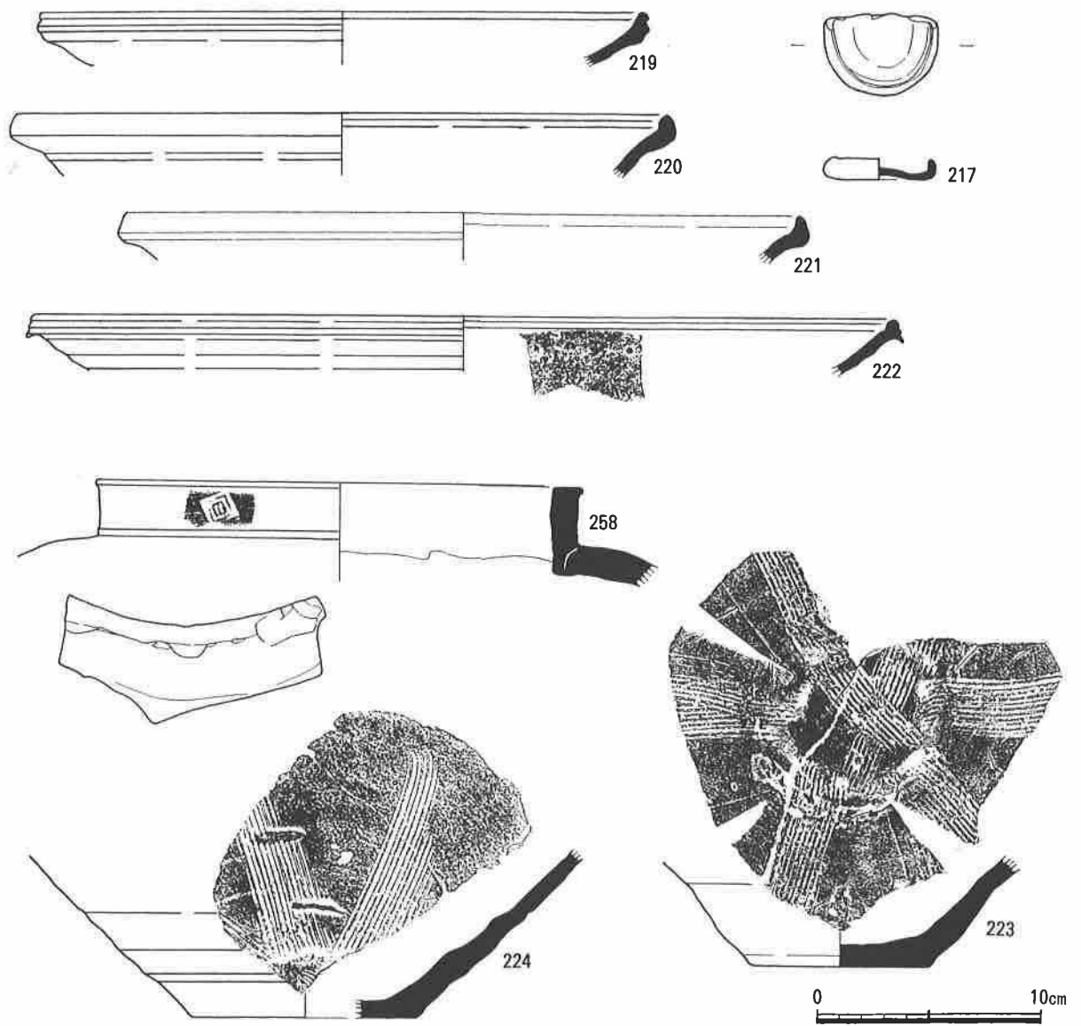
第 30 図 T5 出土遺物実測図 (2)
