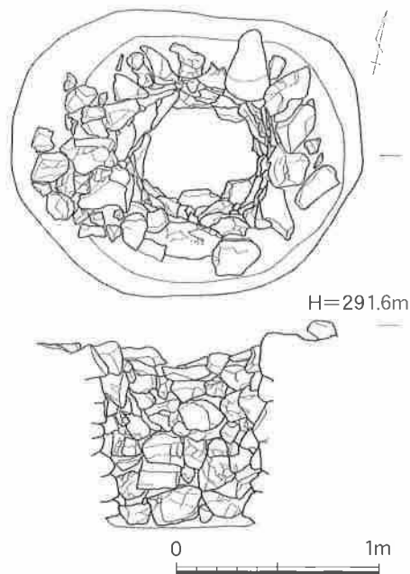
第18図 T4SE1実測図
