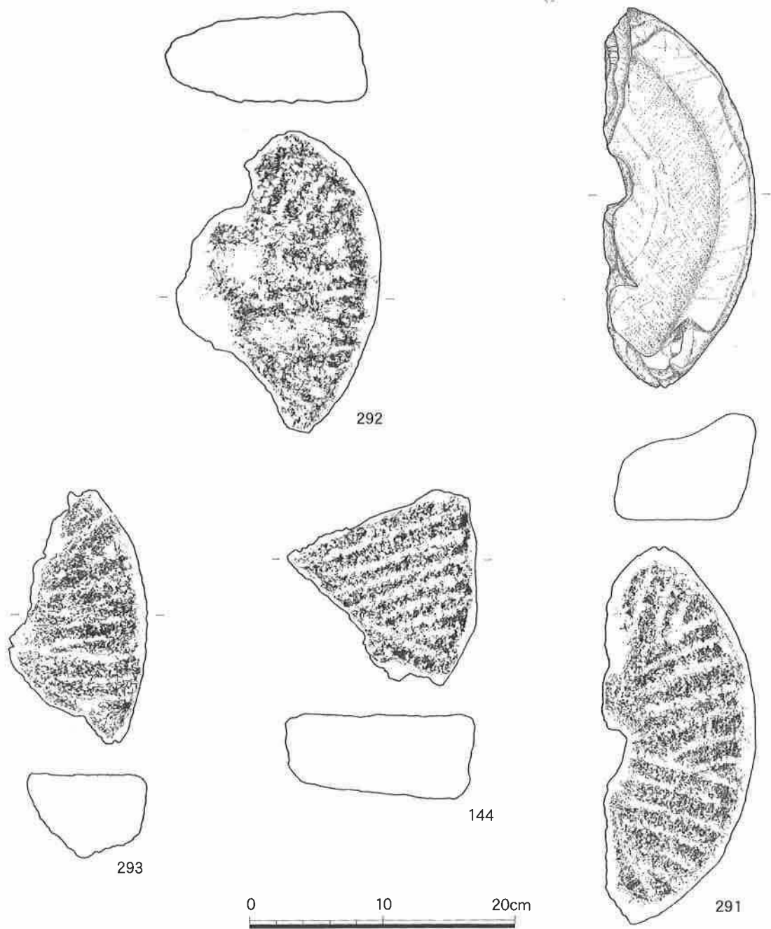
第33図 出土石臼実測図
