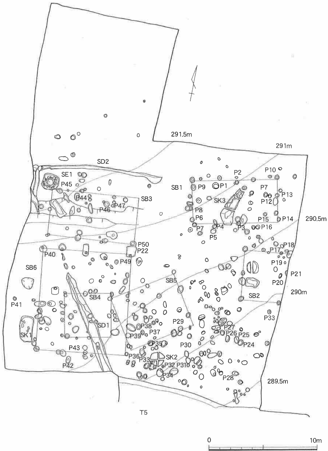
第12図 T4遺構図
