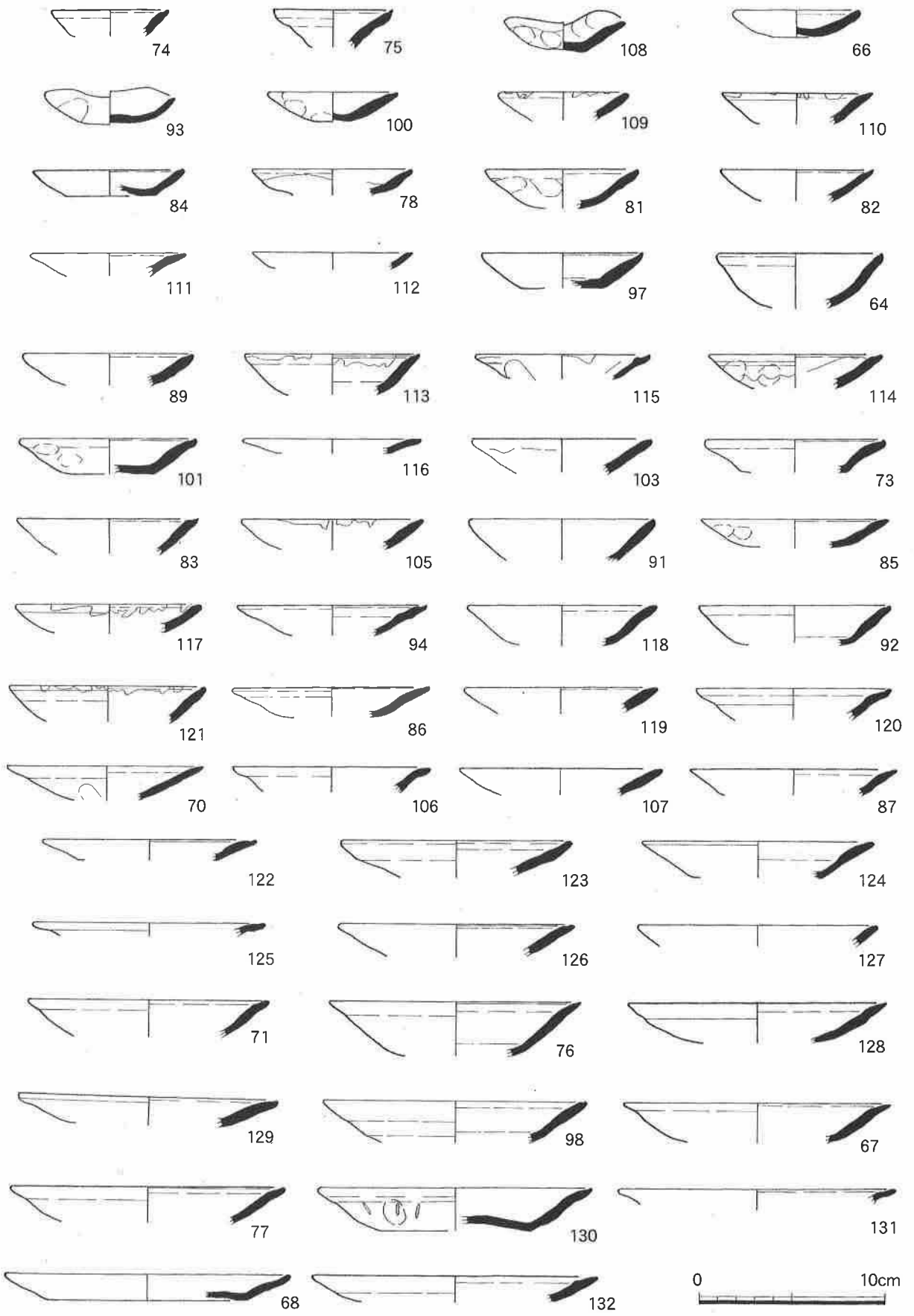
第20图 T4出土遺物実測図 (1)
