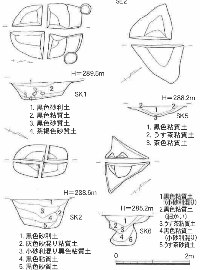
第28図 T5SK1・2・5・6 実測図
