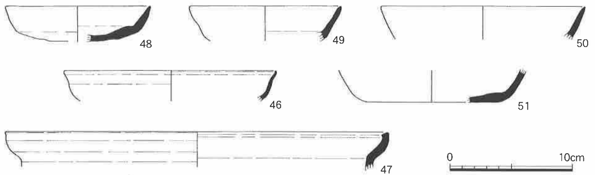
第54図 T11出土遺物実測図 (2)
