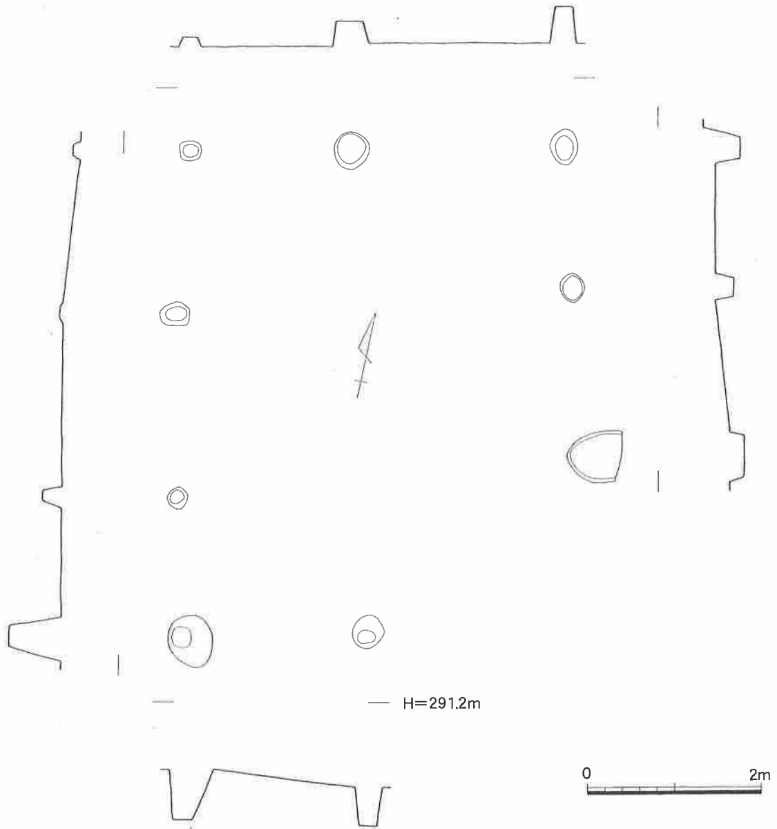
第16図 T4SB4実測図
