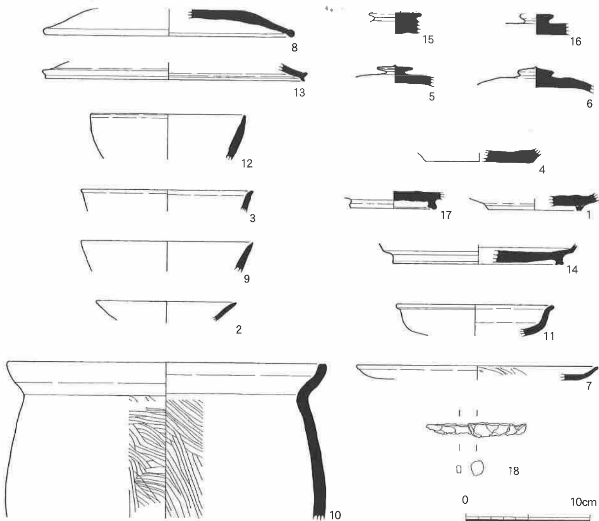
第48図 T1~3出土遺物実測図
