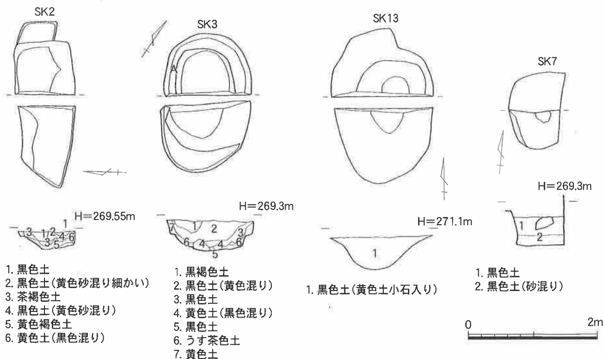
第62図 T12 土坑実測図
