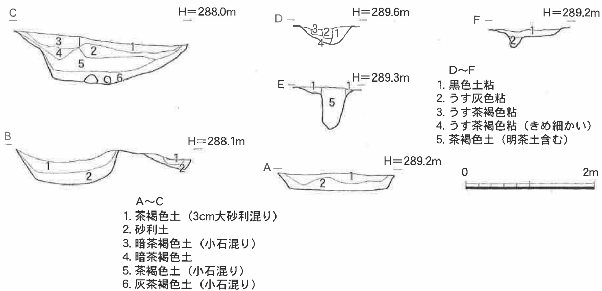
第24図 T5SD1・SD2断面図
