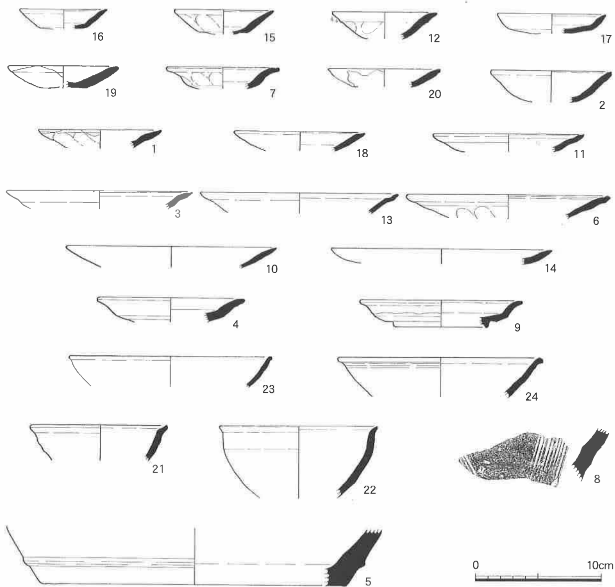
第8図 T2 出土遺物実測図
