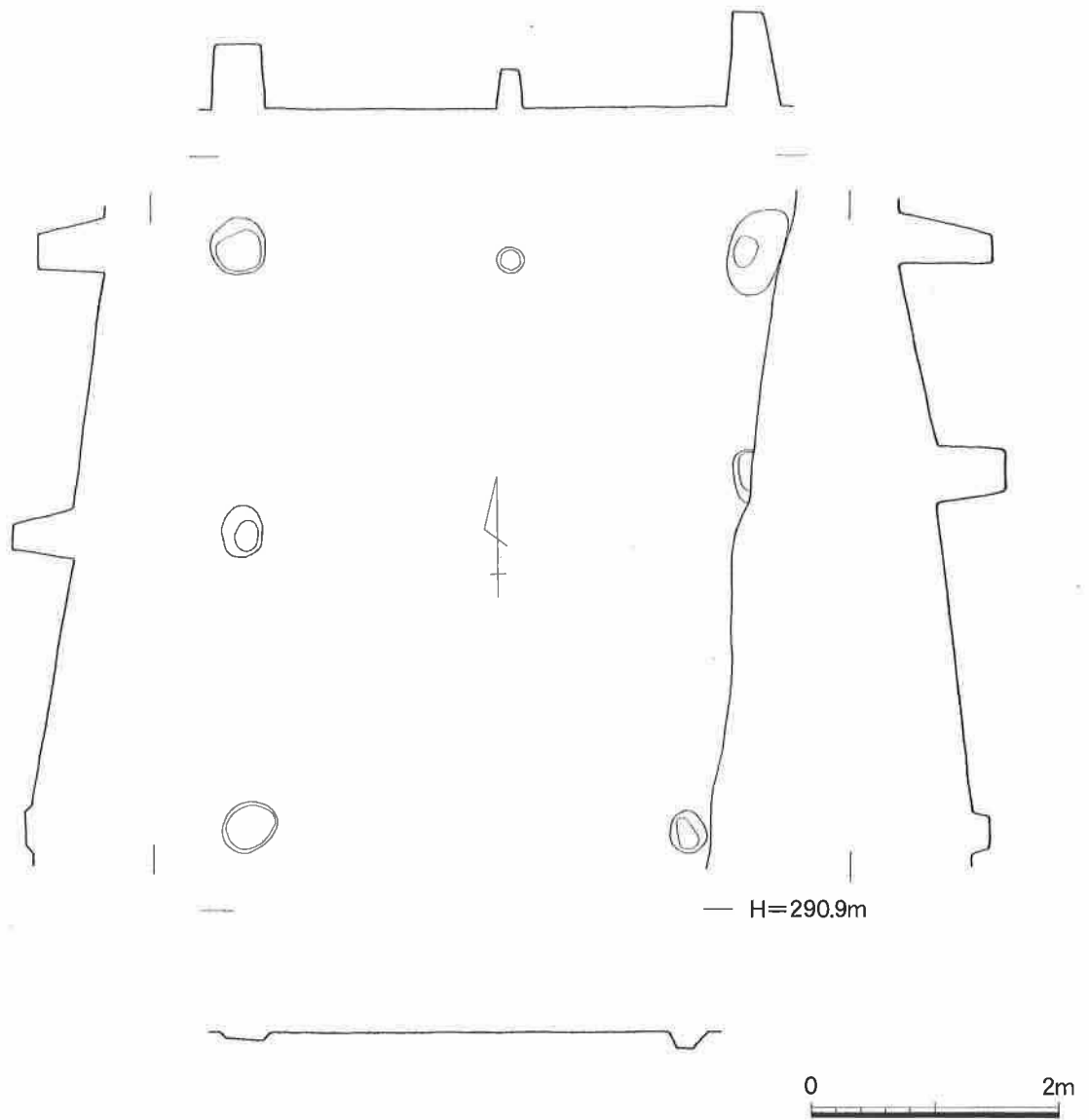
第14図 T4SB2実測図
