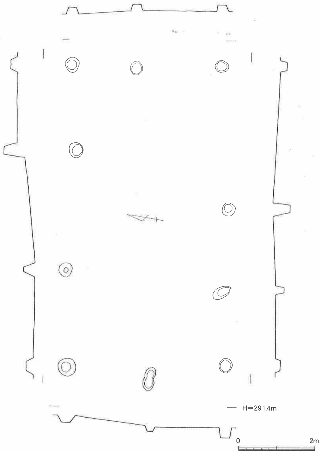
第13図 T4SB1実測図
