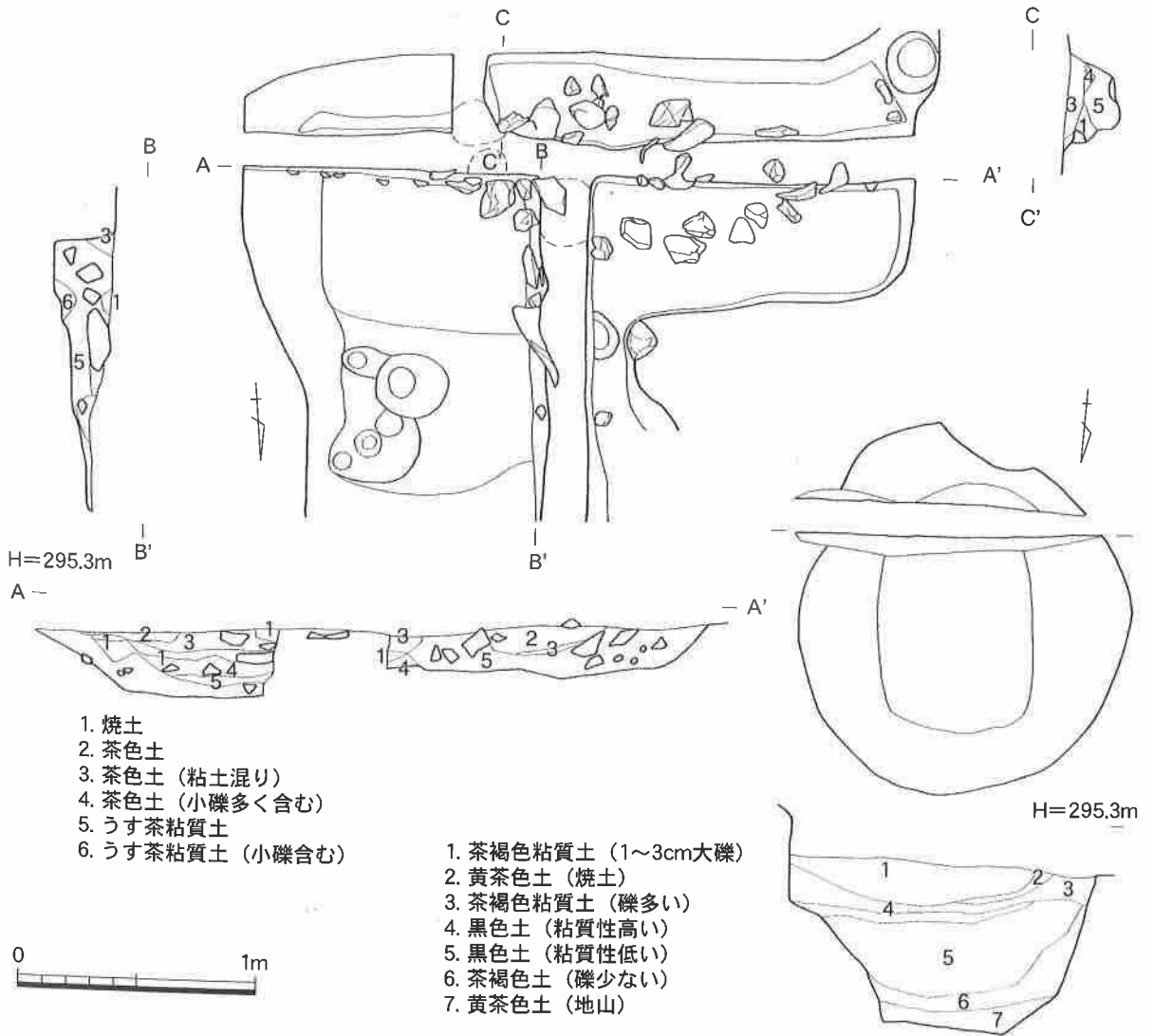
第10図 T3SK1・SK2 実測図
