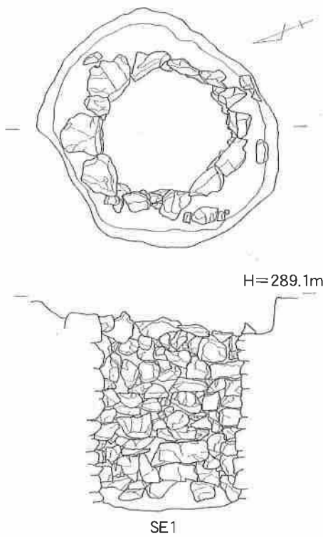
第27図 T5SE1~3 実測図
