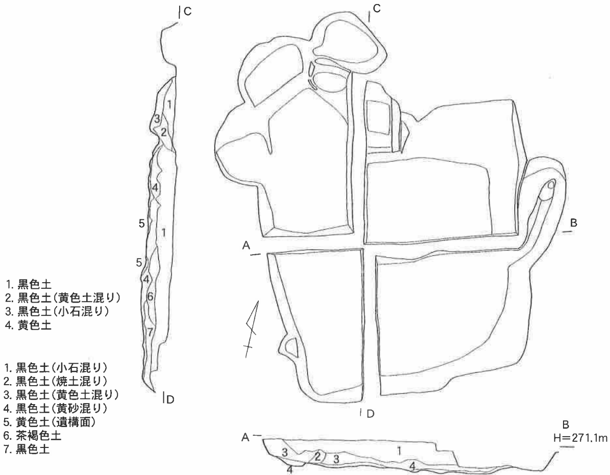
第61図 T12 SH2 実測図
