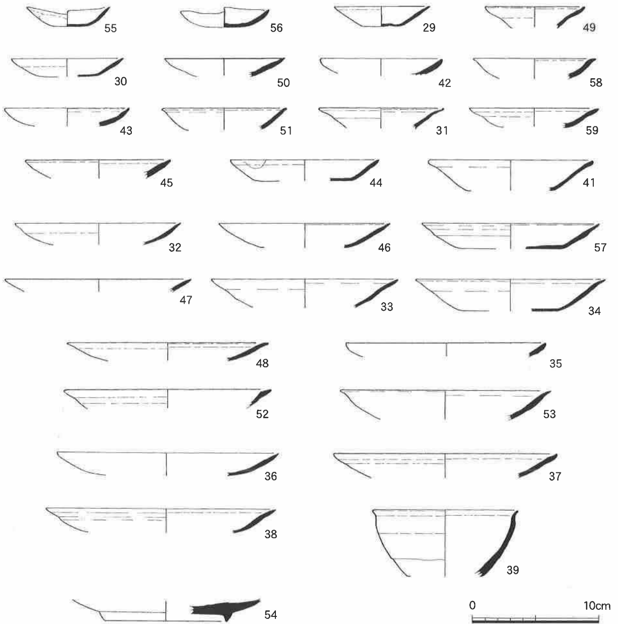
第11図 T3出土遺物実測図
