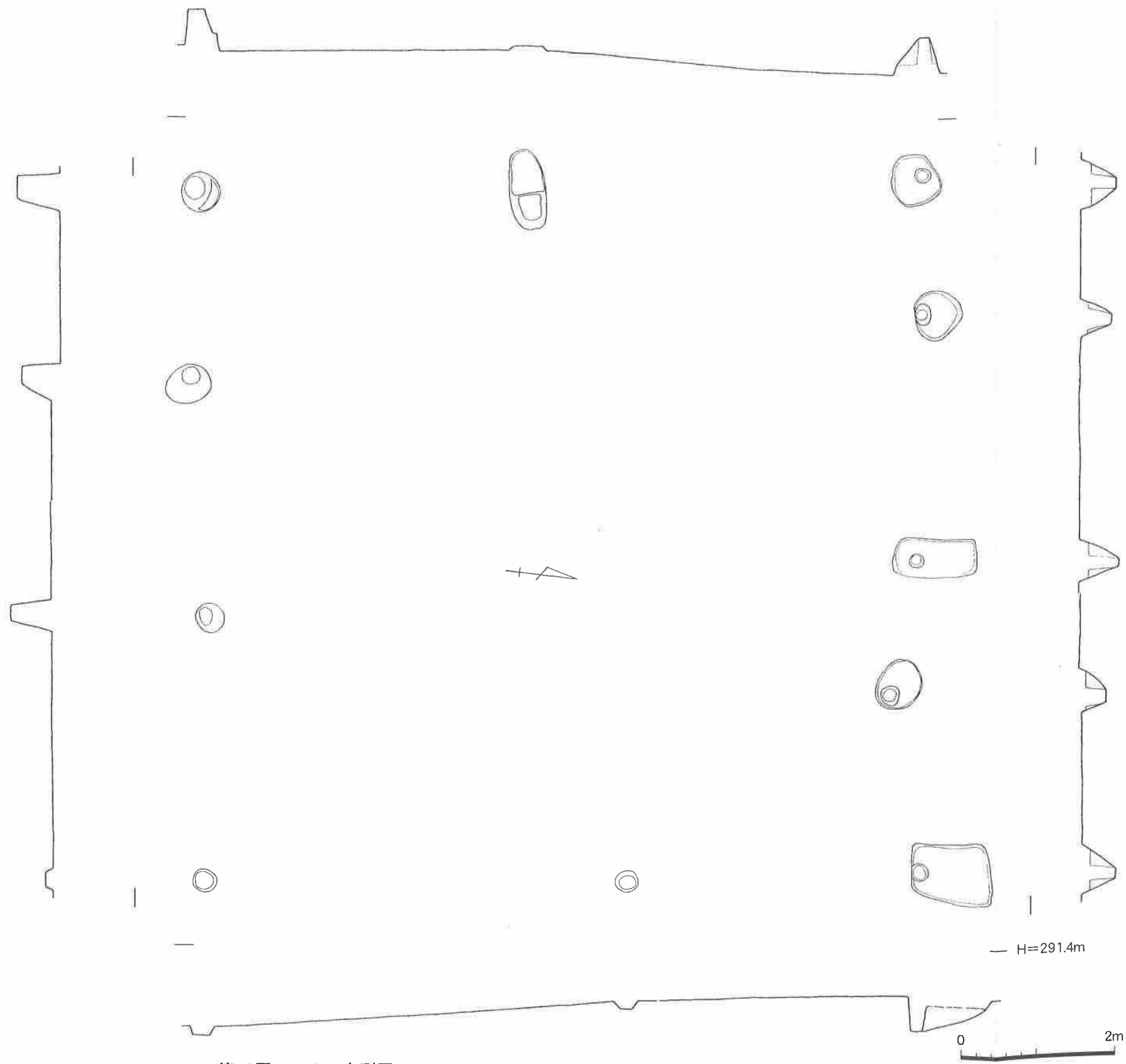
第19図 T4SB6実測図
