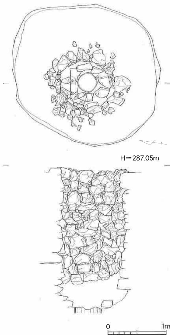
第37図 T7SE1実測図
