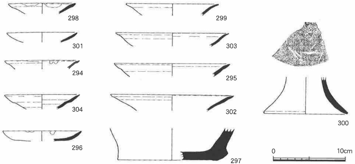
第38図 T7出土遺物実測図
