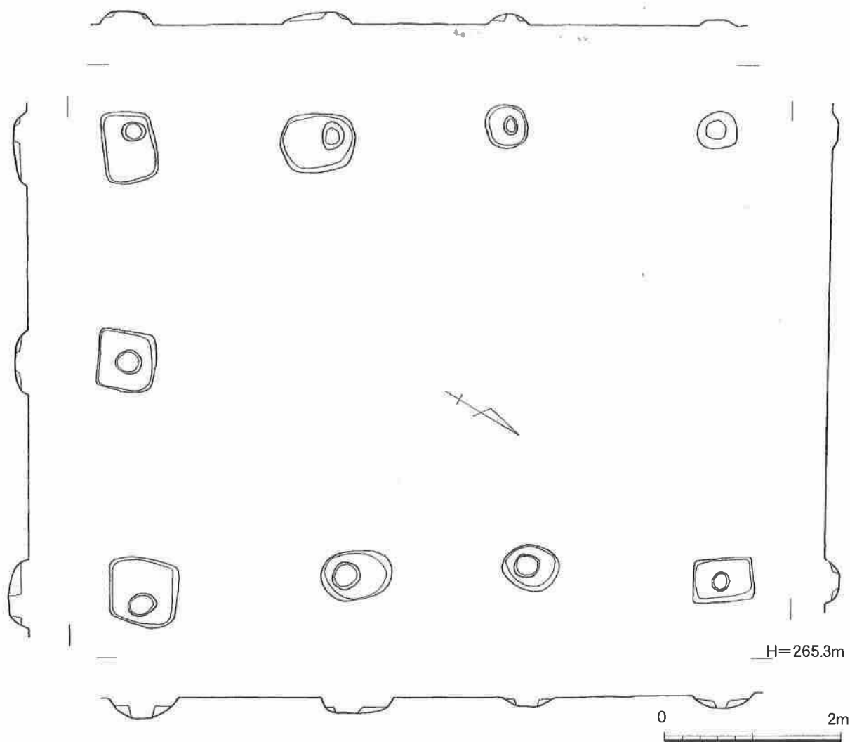
第47図 T3SB1実測図
