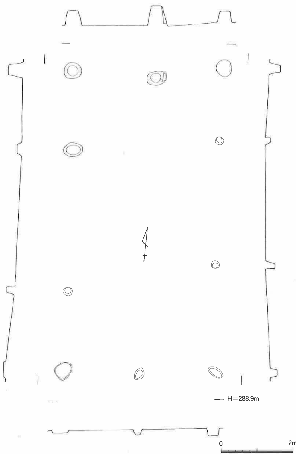
第25図 T5SB2実測図
