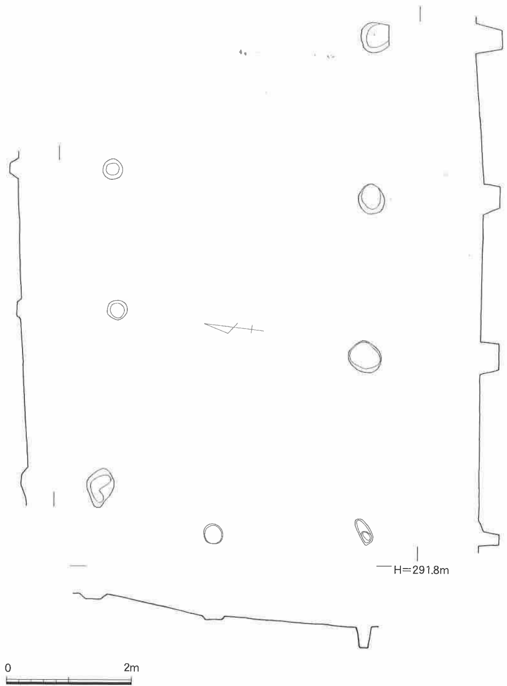
第15図 T4SB3実測図
