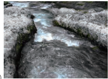
写真3 北坂本累層の凝灰角礫
