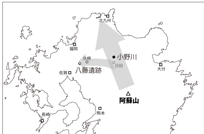
第13図 小野川への阿蘇4火砕流の流れ
