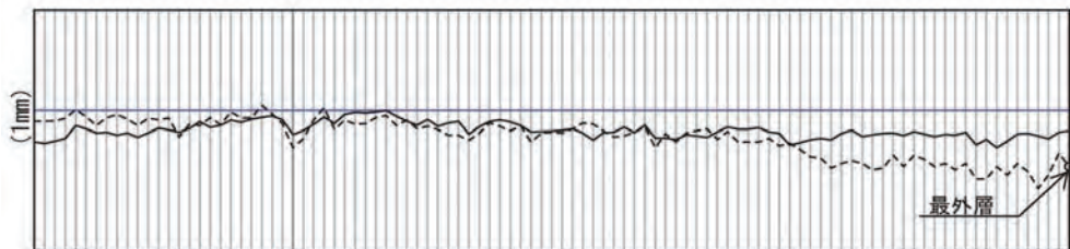
第12図 八藤遺跡出土トウヒ属6点（実線）の平均値パターングラフと小野川埋没林トウヒ属4点（点線）の平均値パターングラフの一致状況
