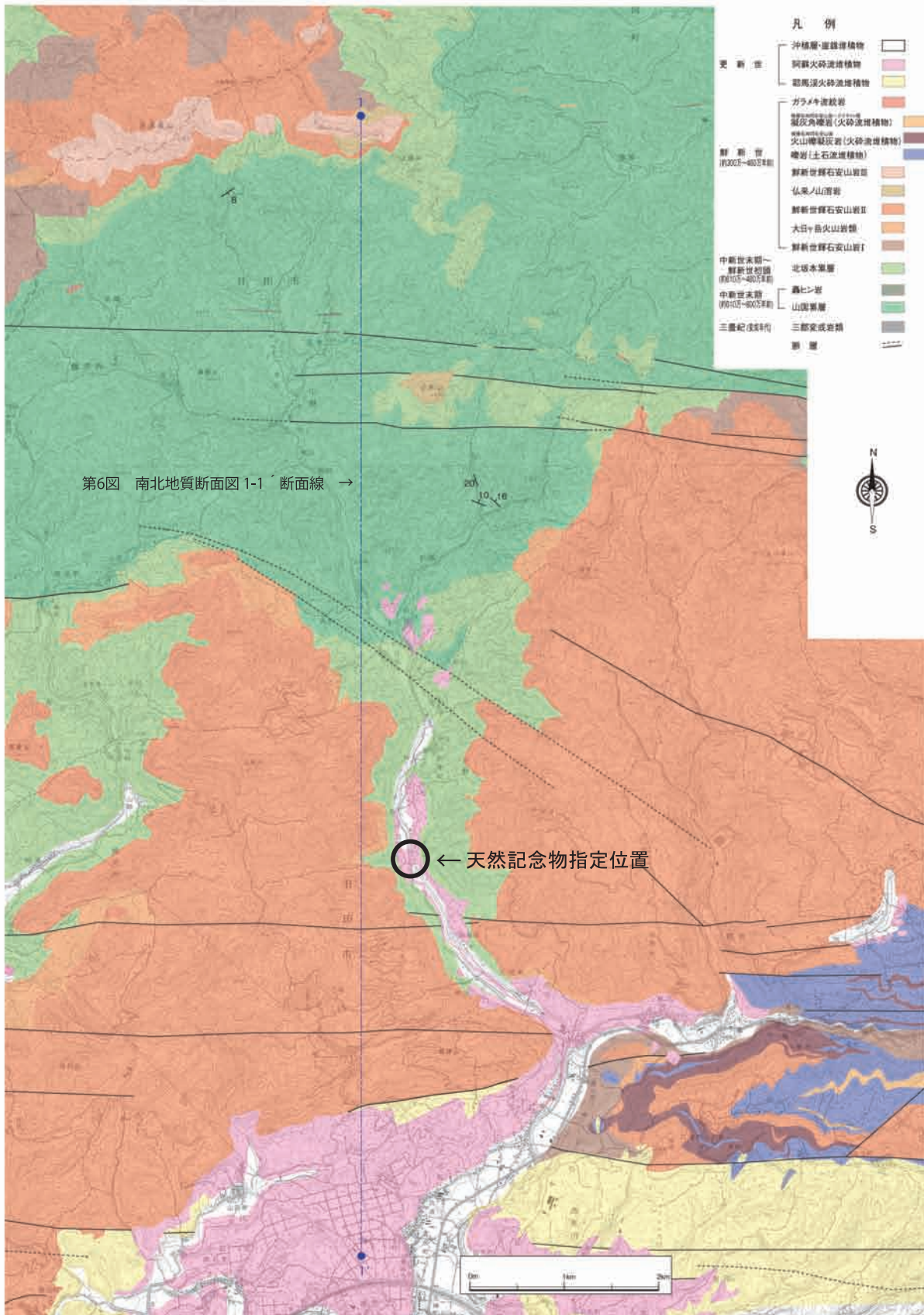
第5図 小野川流域の地質図
