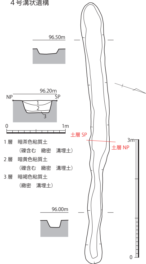
第11図 溝状遺構実測図 (1/60・土層 1/40)
