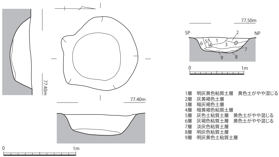
第14図 2号土坑実測図 (1/30・土層 1/40)
