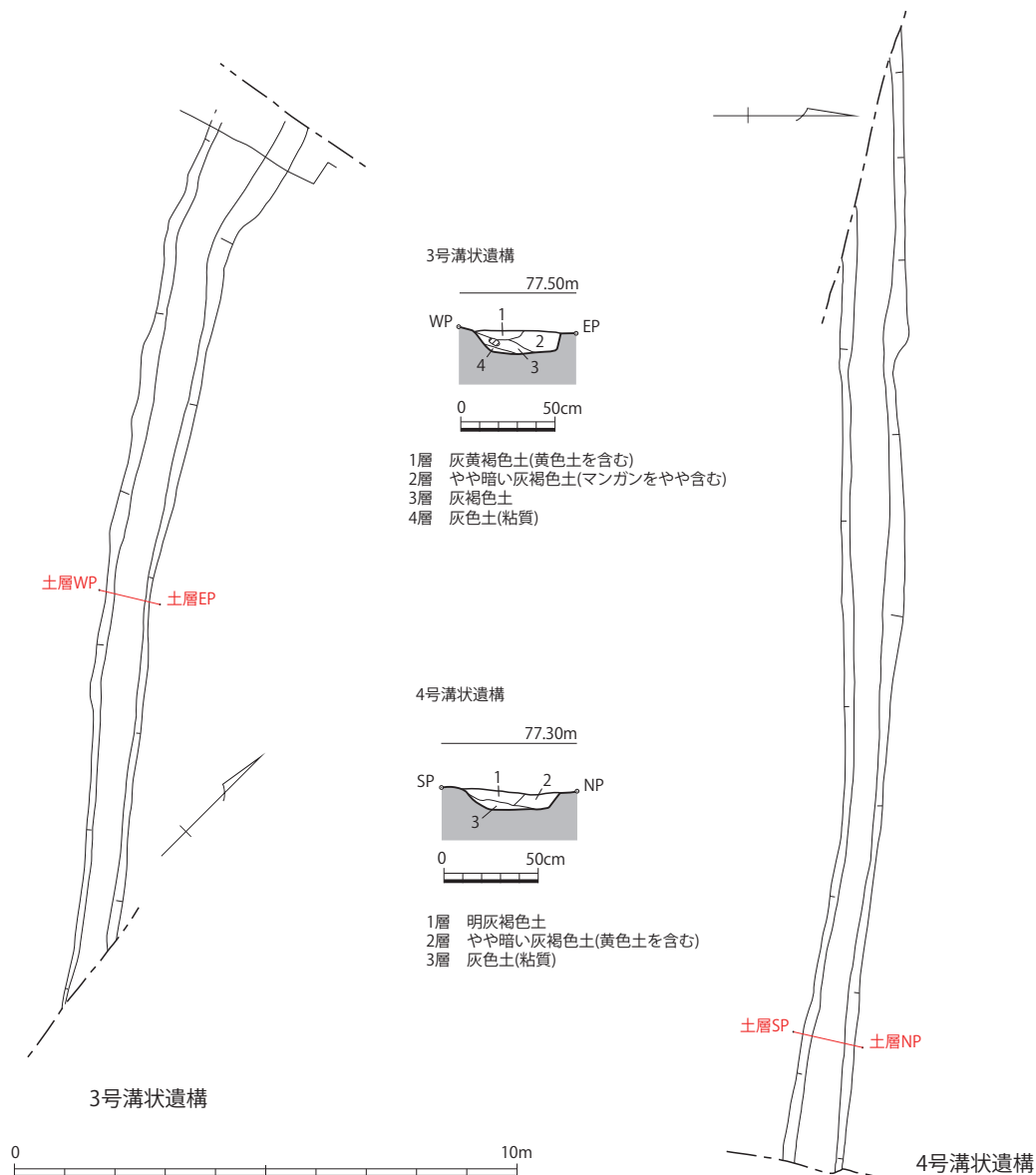
第27図 3・4号溝状遺構実測図 (1/150・土層 1/40)
