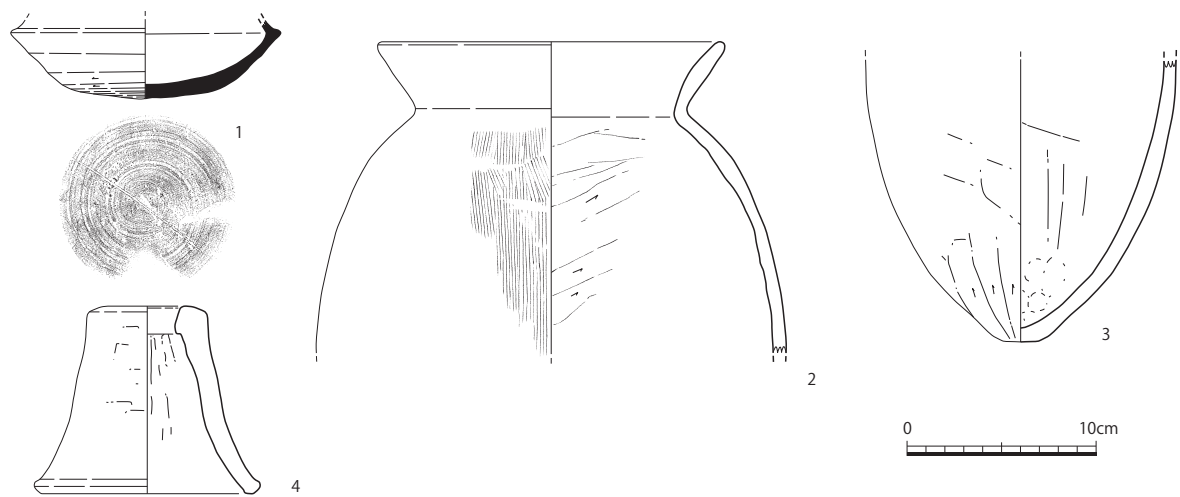
第26图 1・2号溝状遺構出土遺物実測図 (1/4)
