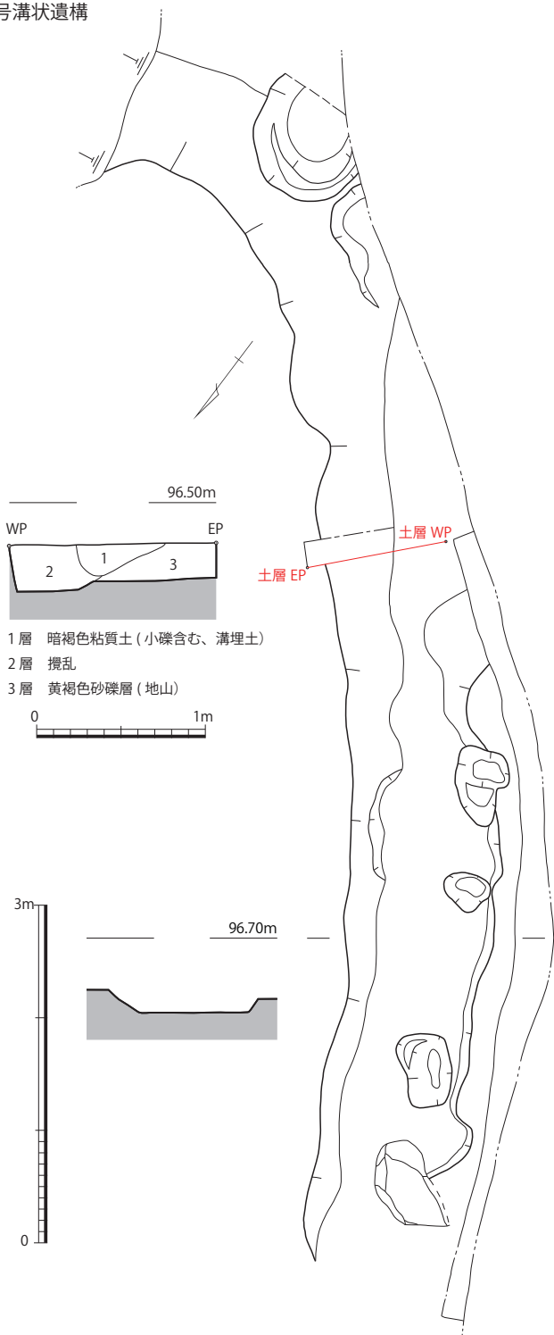
第11図 溝状遺構実測図 (1/60・土層 1/40)
