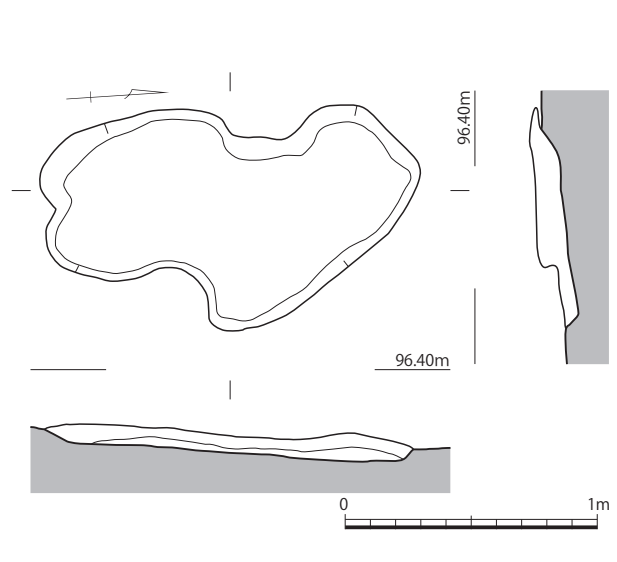
第10図 土坑実測図(1/30)
