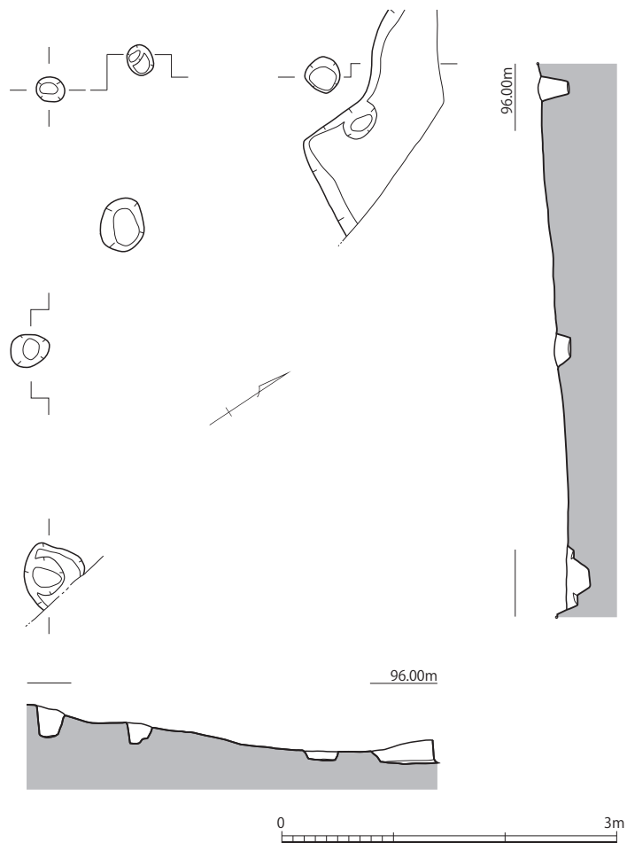
第6図 2号掘立柱建物実測図（1/60）
