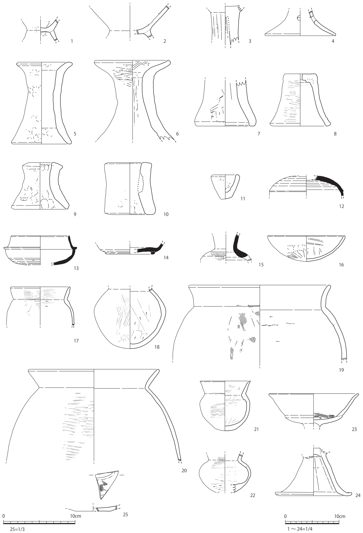
第20图 1号溝状遺構出土遺物実測図(3)(1/3・1/4)
