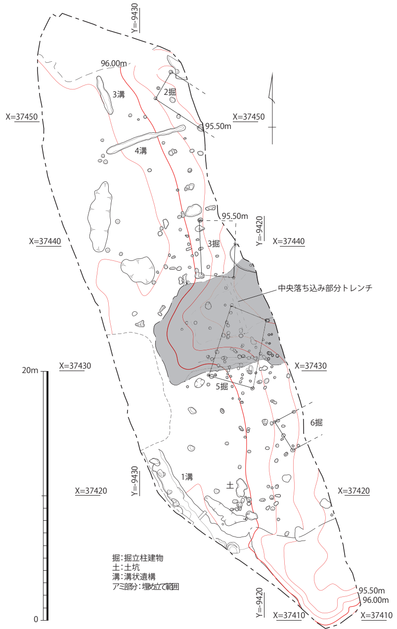
第4図 遺構配置図 (1/300)
