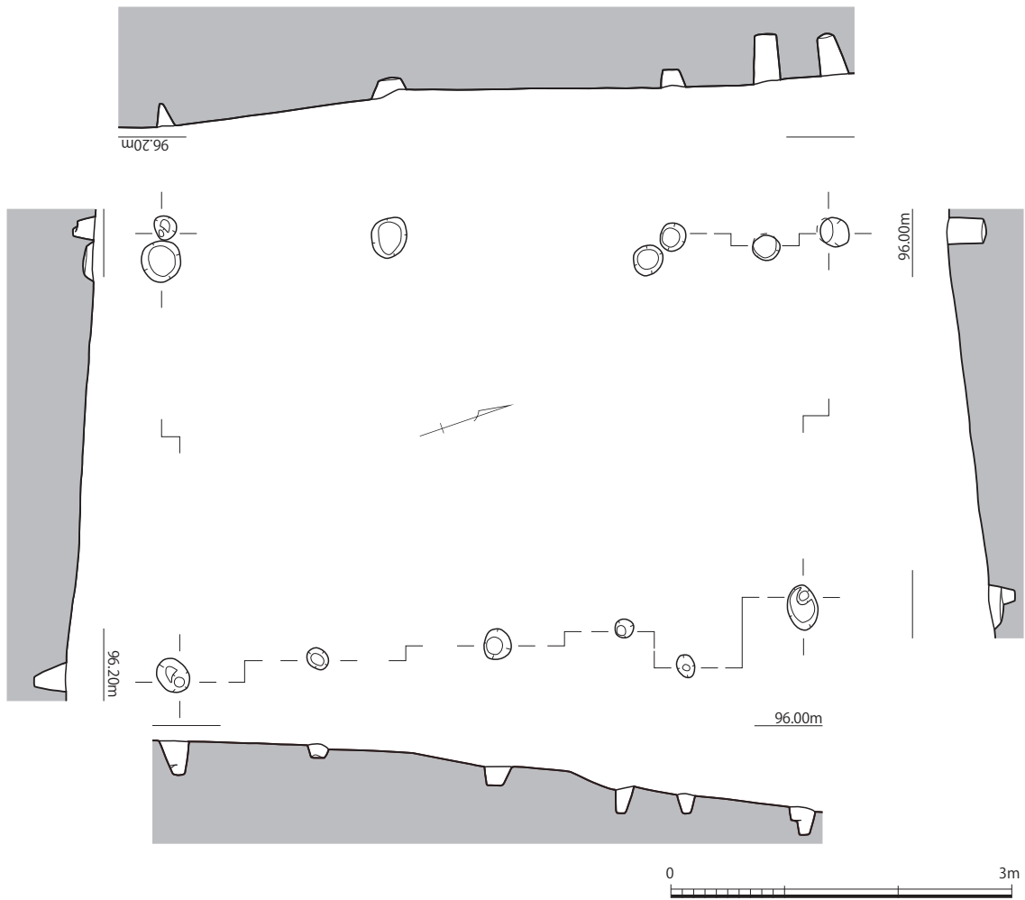
第8图 5号掘立柱建筑物实测图 (1/60)
