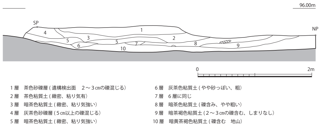
第5図 中央落ち込み部分土層実測図 (1/40)
