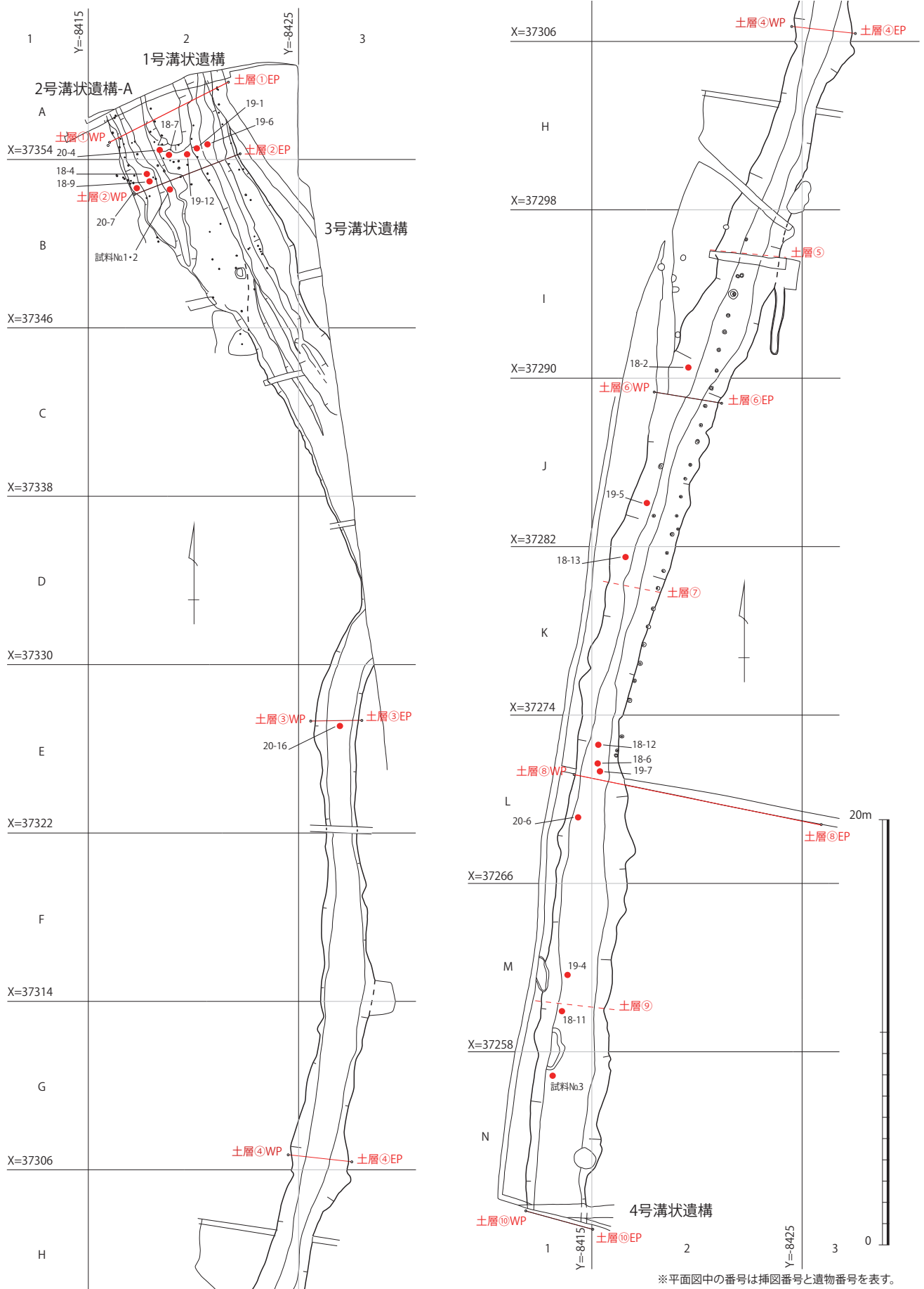
第 16 図 1号溝状遺構実測図 (1/250)
