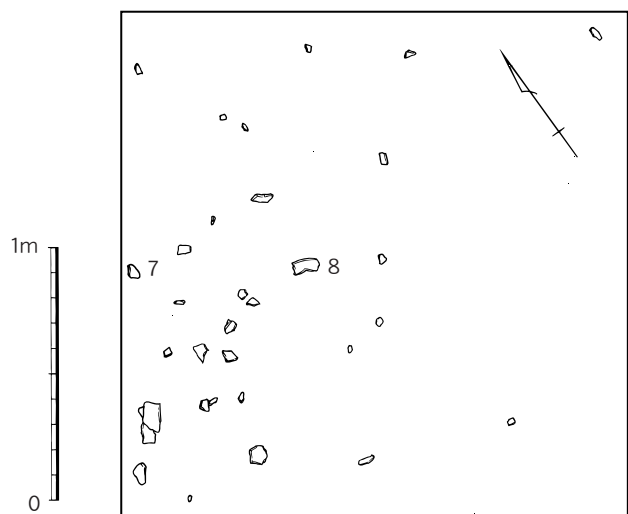
第6図 1トレンチ実測図② (1/30)
