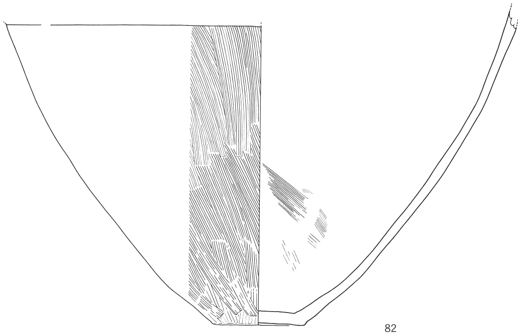
第24図 表採土器実測図② (1/4)
