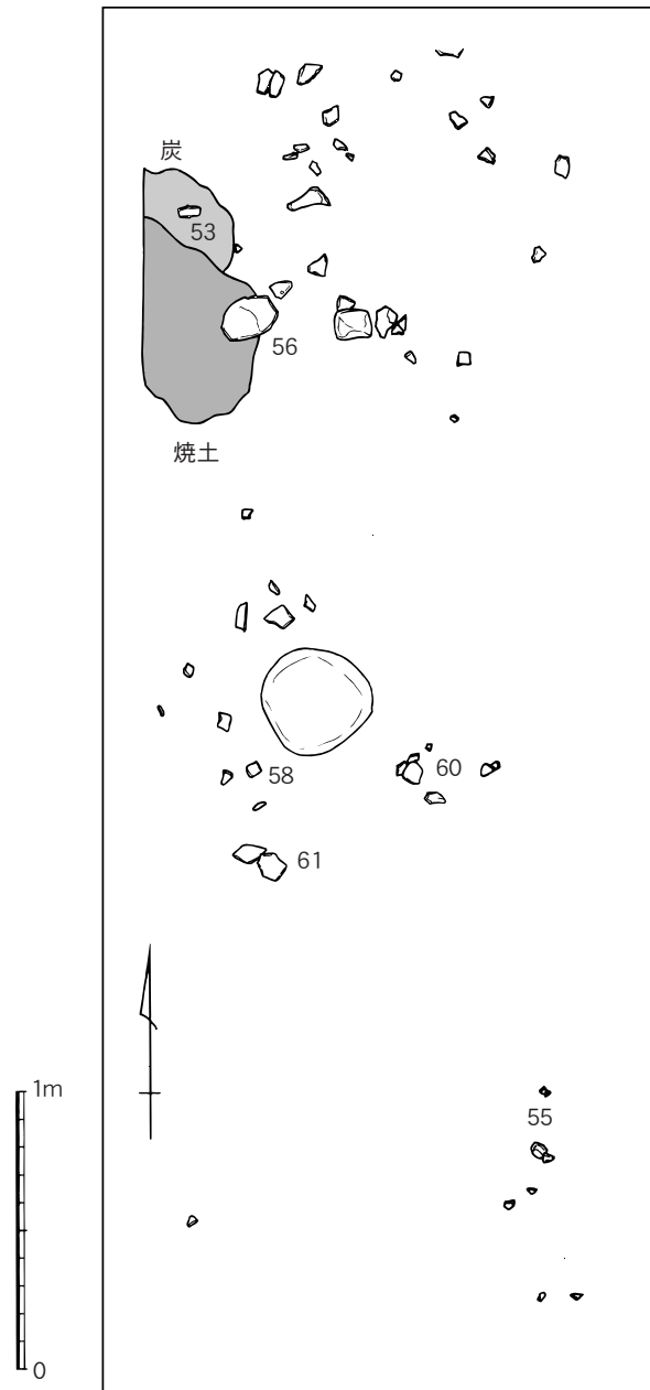
第19図 6 トレンチ実測図 (1/30)
