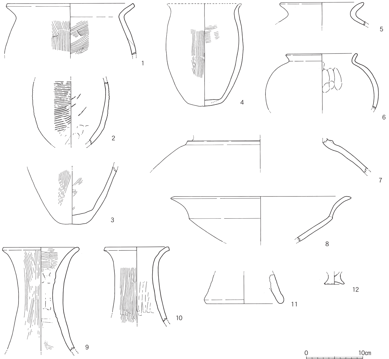
第7図 1トレンチ出土土器実測図(1/4)
