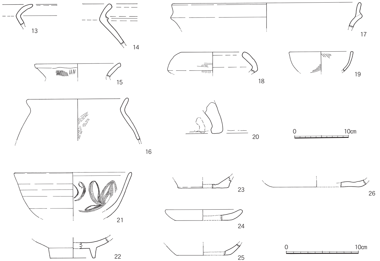
第9図 2トレンチ出土土器実測図 (1/4・1/3)
