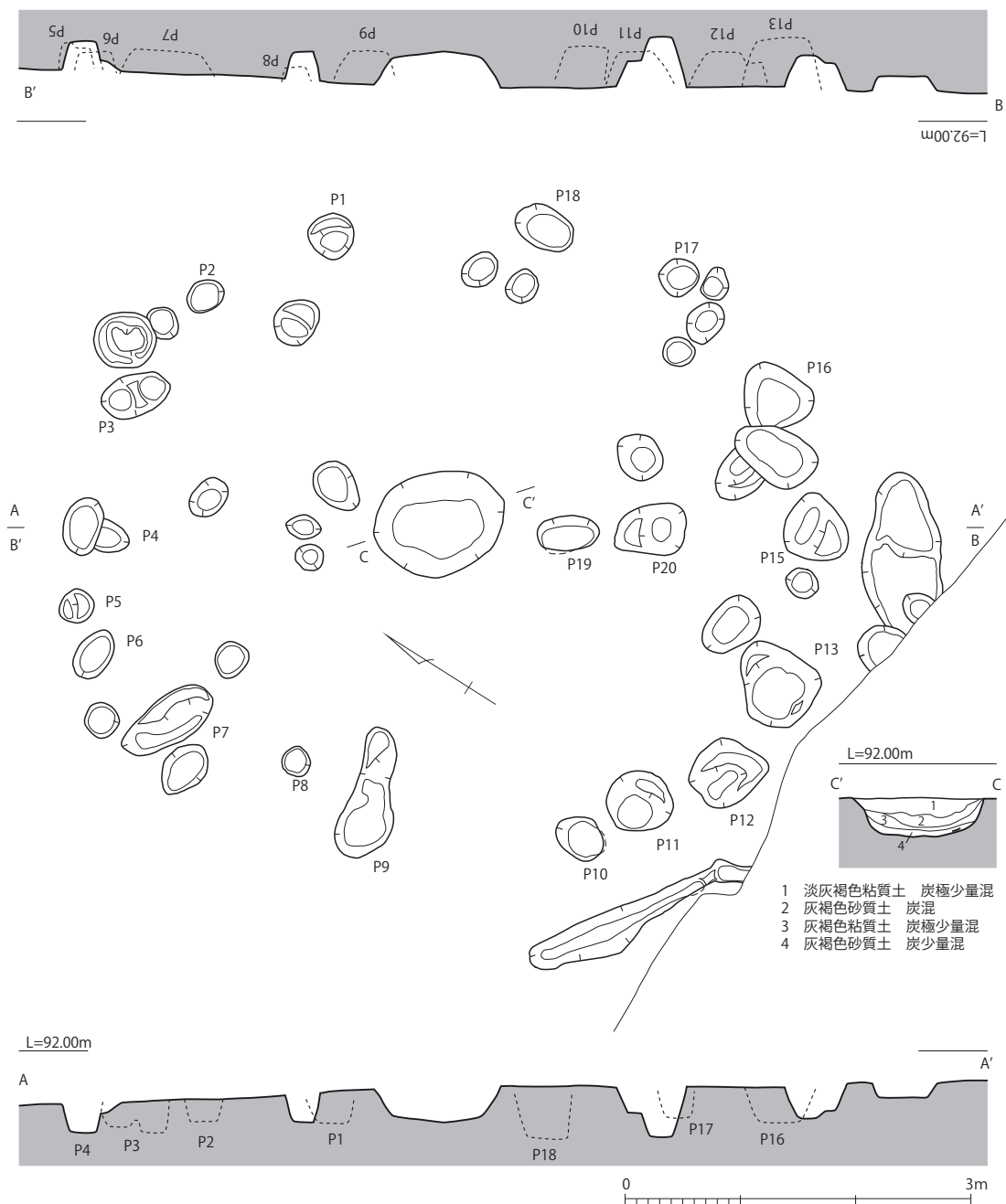
第5図 竪穴建物実測図 (1/60)
