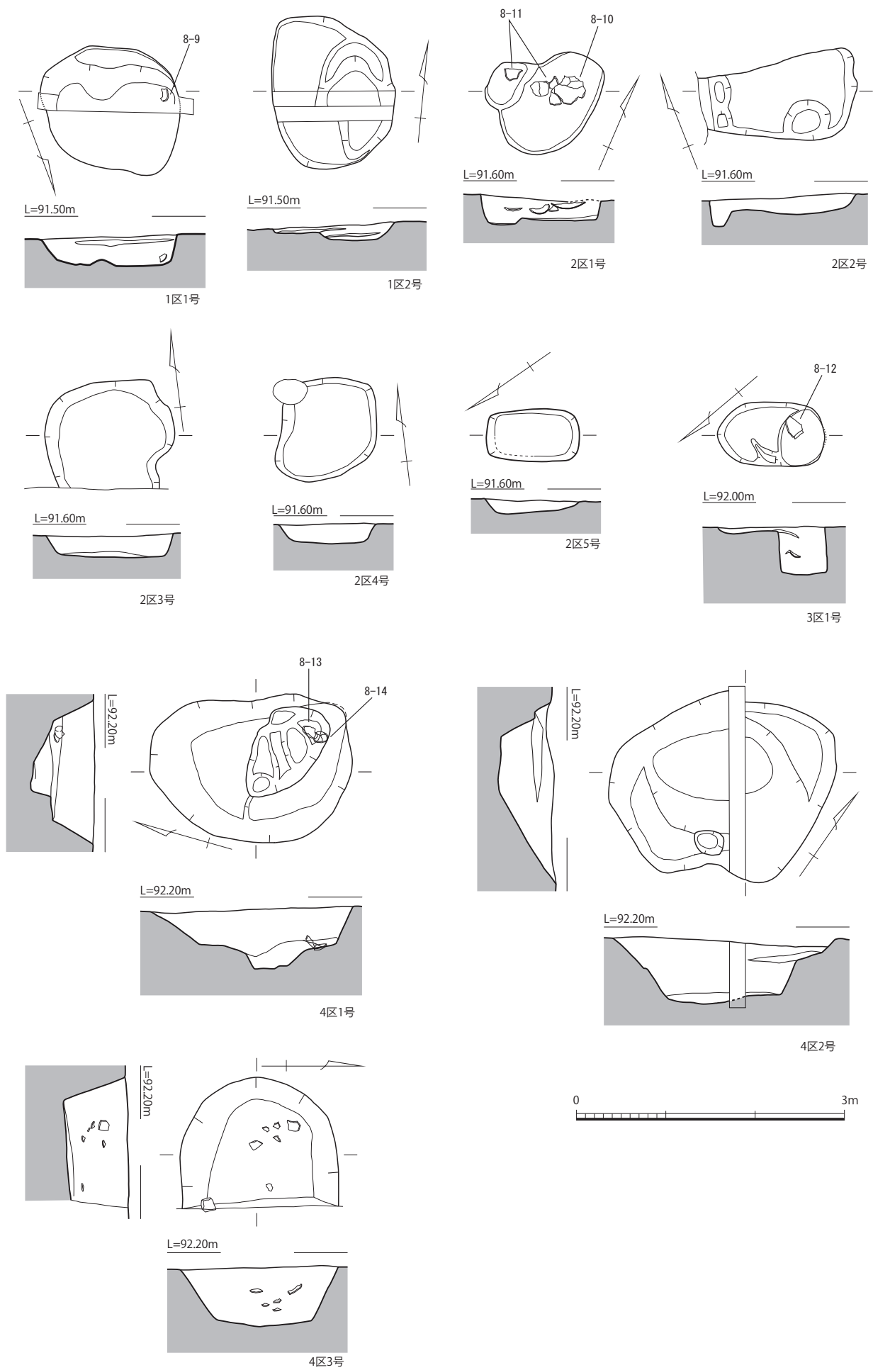
第 6 图 土坑实测图 (1/60)
