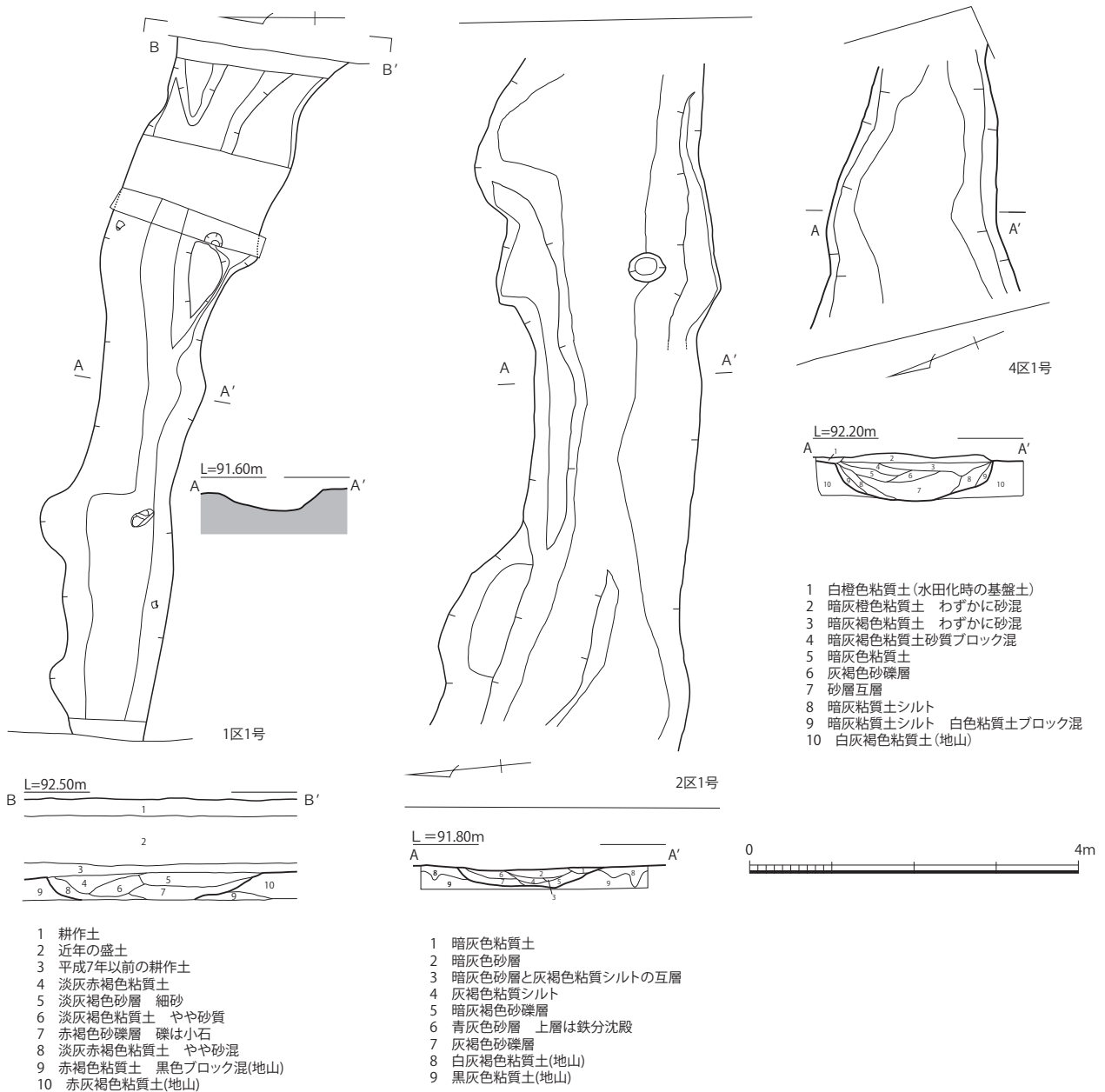
第7図 溝状遺構実測図 (1/80)
