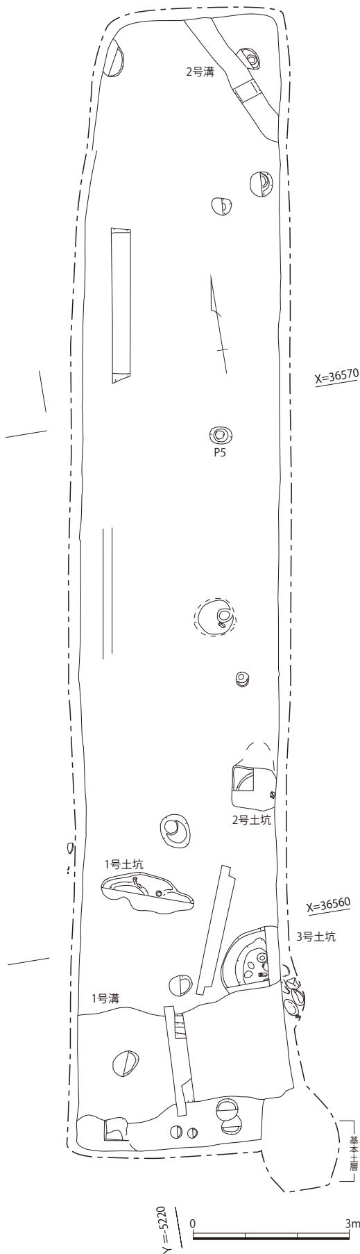
第5図 遺構配置図 (1/100)
