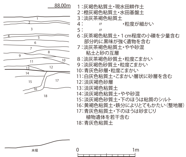
第4図 基本土層図 (1/40)
