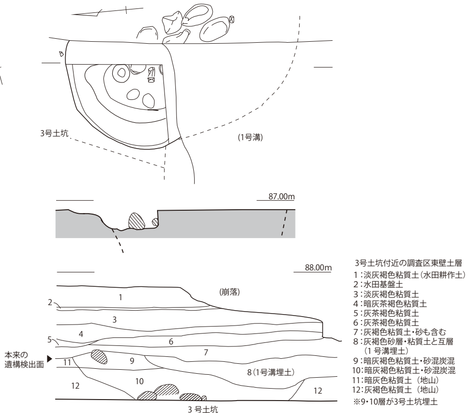
第6図 1～3号土坑、1・2号溝実測図 (1/40、1/80)
