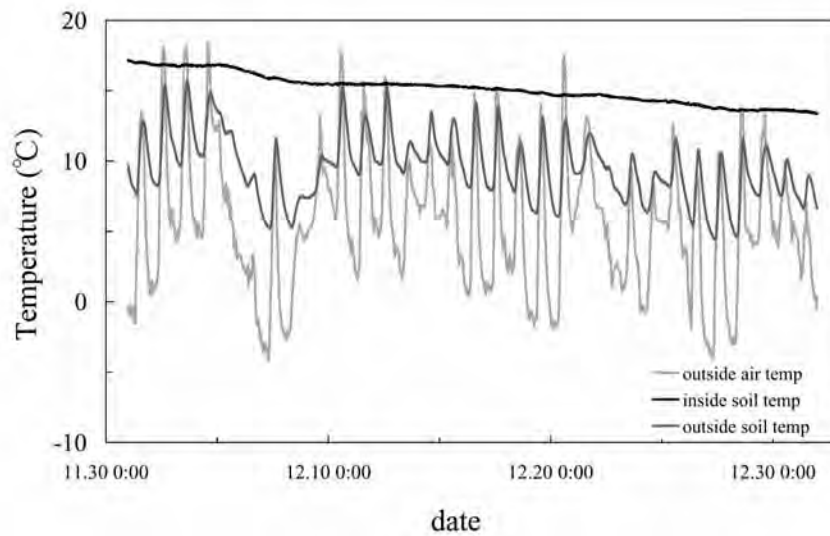
第 40 図 外気温と土壌温度（冬季）
