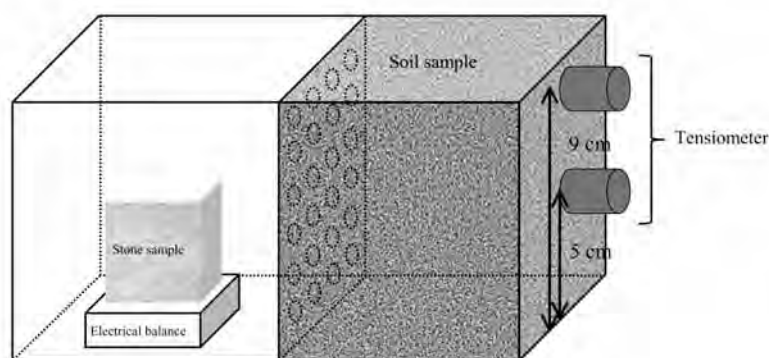
第 38 図 模擬石室実験模式図
