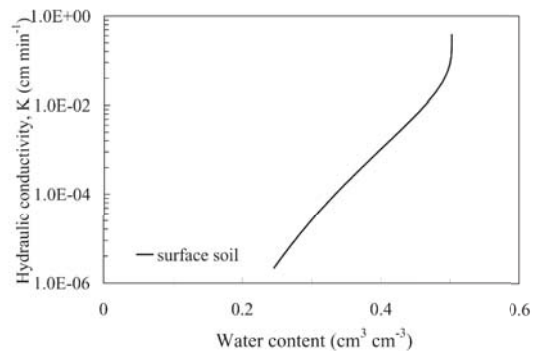
第 43 図 1号墳表土の不飽和透水係数
