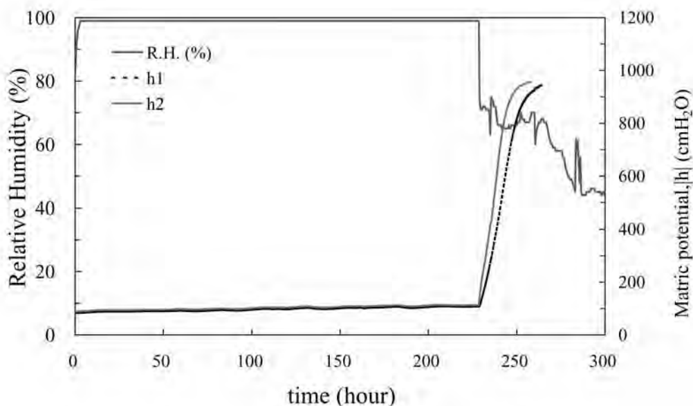
第 47 図 マトリックポテンシャルと相対湿度
