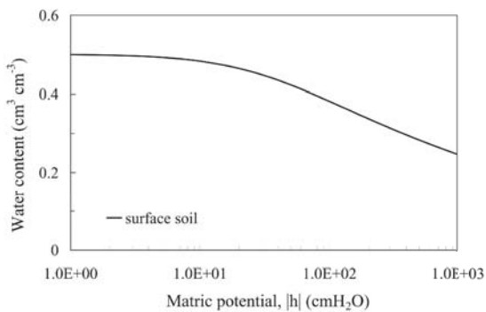
第 42 図 1号墳表土の水分特性曲線
