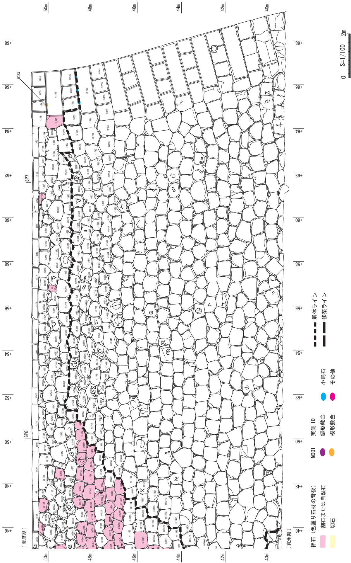
第211図 押石・敷金等使用色分け図7 口面北 (2120E) (S=1/100)
