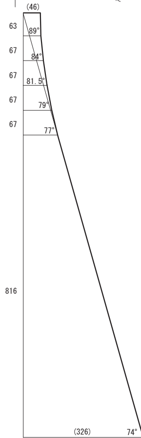
第220図 石垣勾配の比較 (S = 1/100)
