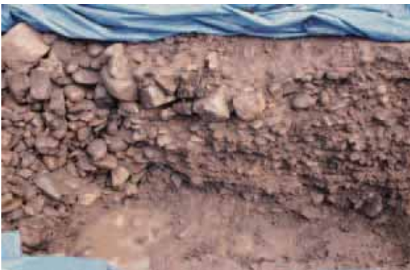
橋爪門続櫓台南北土層断面 SP11 L=49.3_48m付近東壁北側 1
