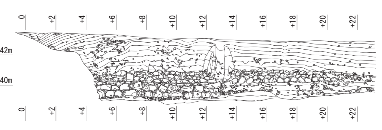
石垣立面图 1 (S=1/150)
