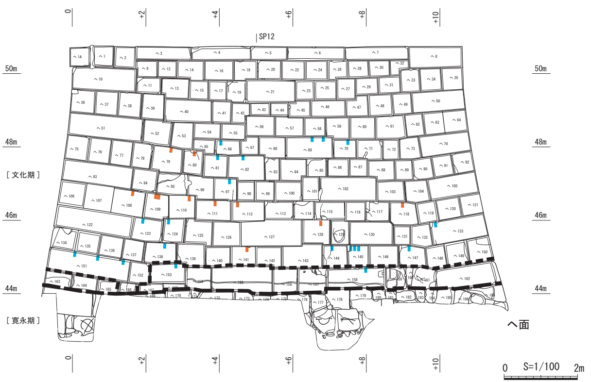
第203図 「梃子穴」立面投影図3 イ (2110N)・へ面 (2110E) (S=1/100)
