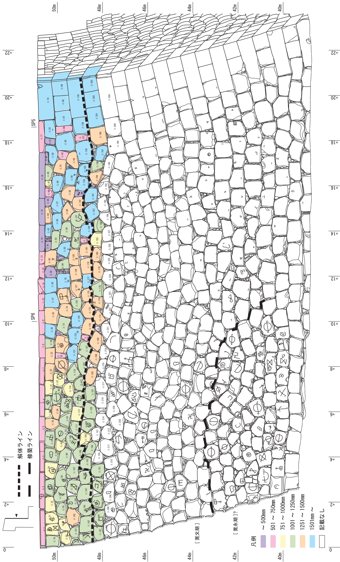
第169図 控え長別色分け図2 二面 (2140E) (S=1/100)
