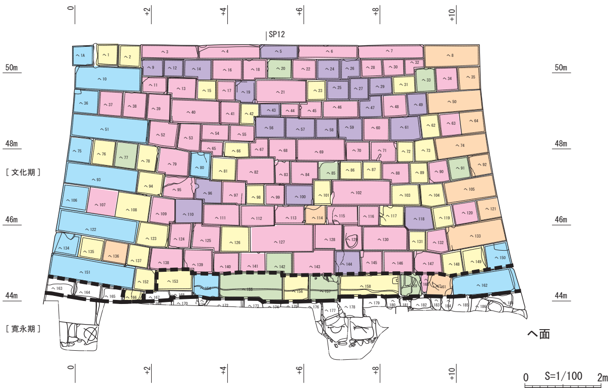
第177図 控え長別色分け図 10 イ (2110N)・ハ面 (2110E) (S=1/100)
