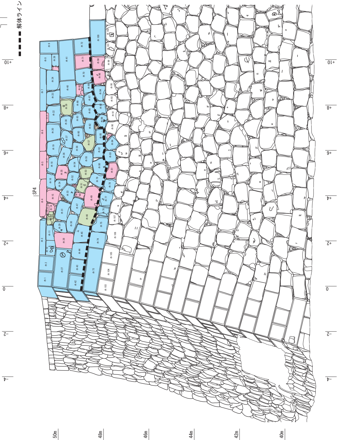
第190図 石材(色調)別色分け図1 赤面(2140N) (S=1/100)
