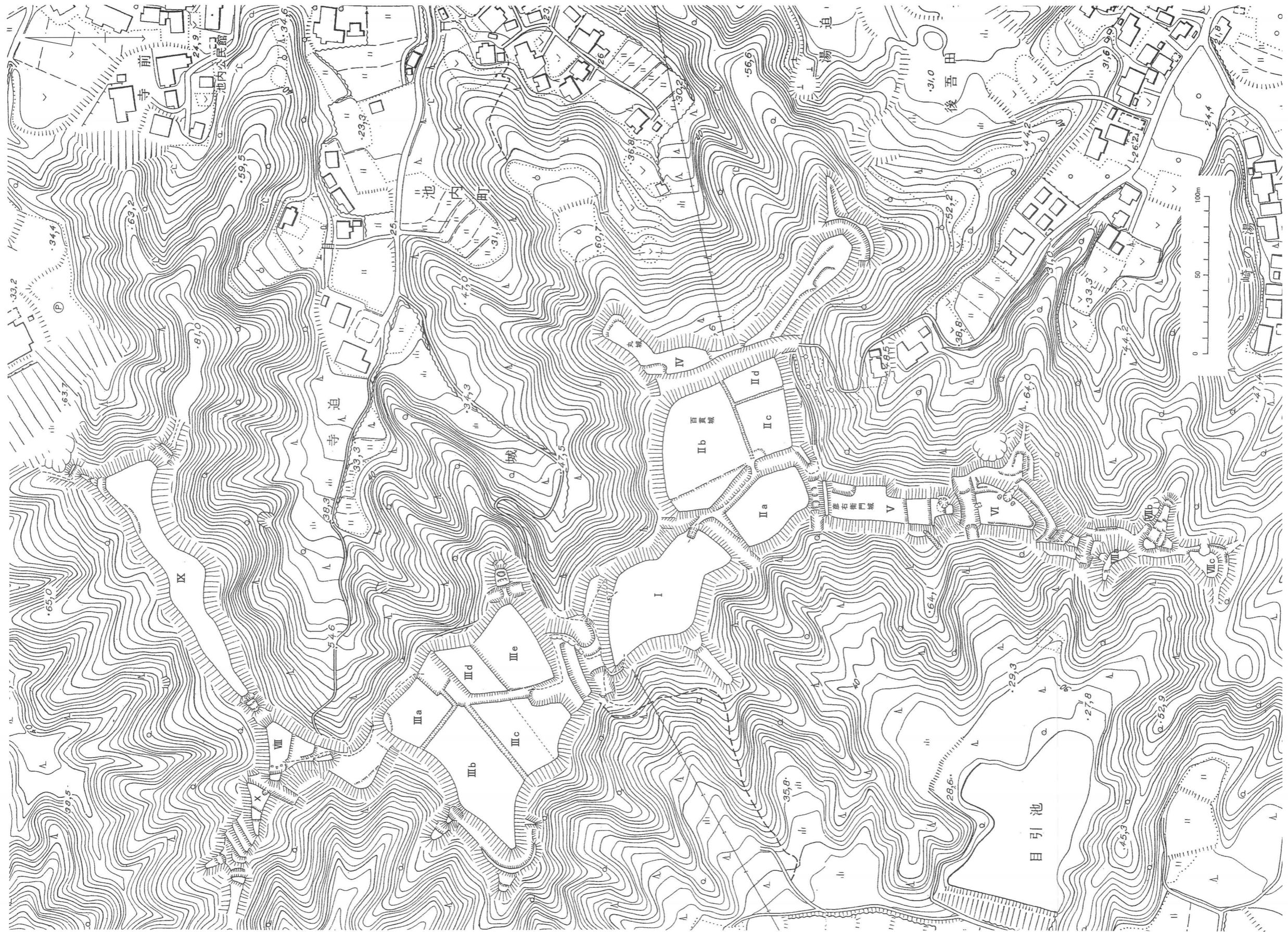
第6図 宮崎城縄張図
