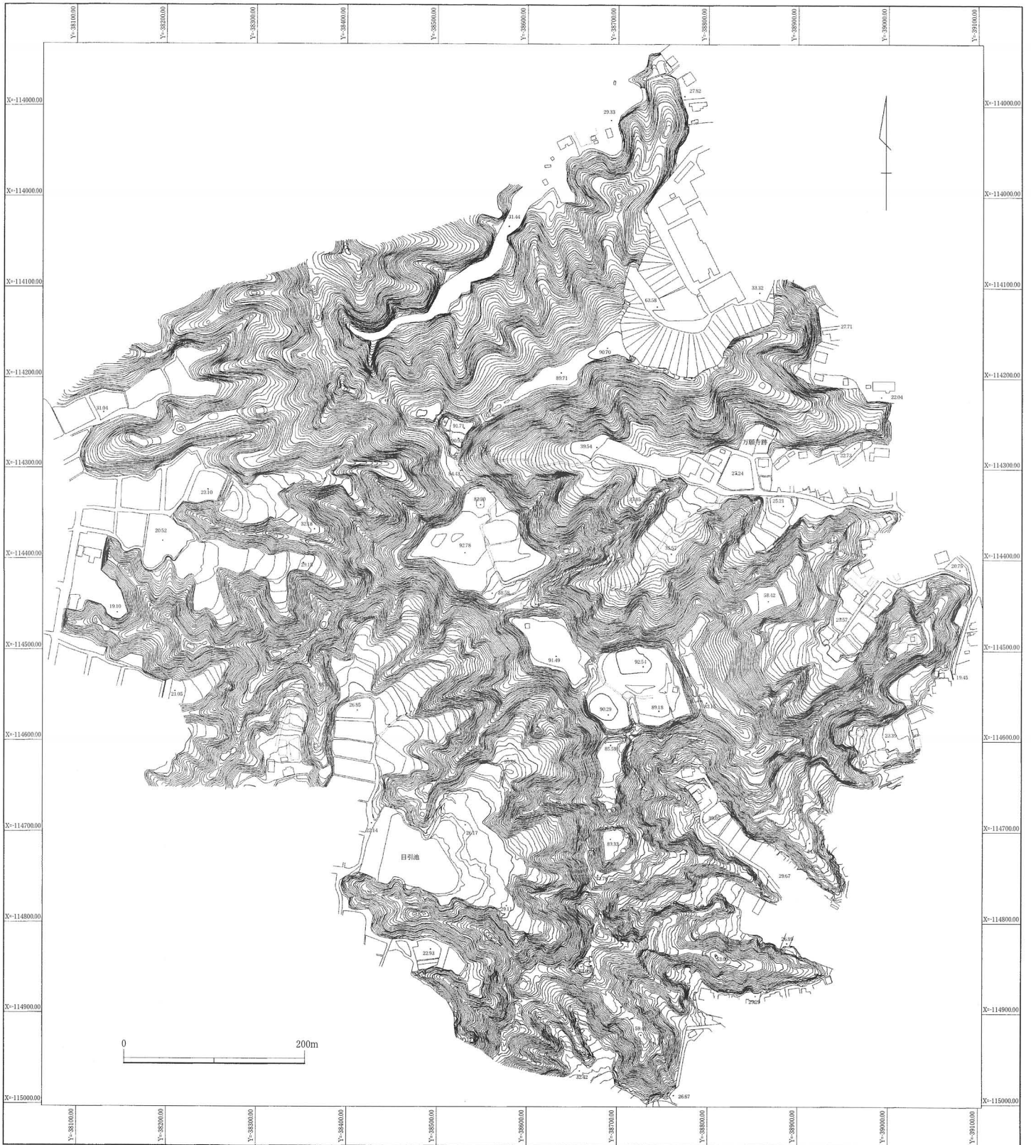
第7図 宮崎城現況地形測量図
