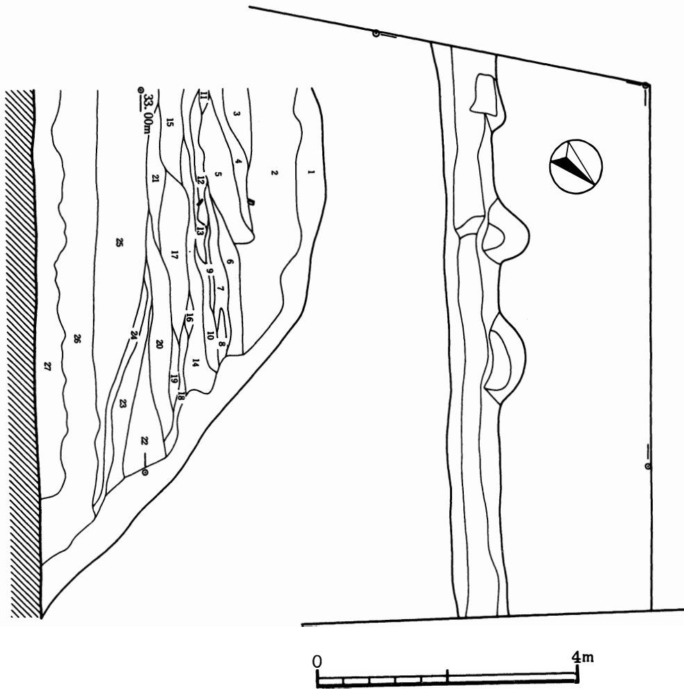
第14図 二の丸土層断面図
