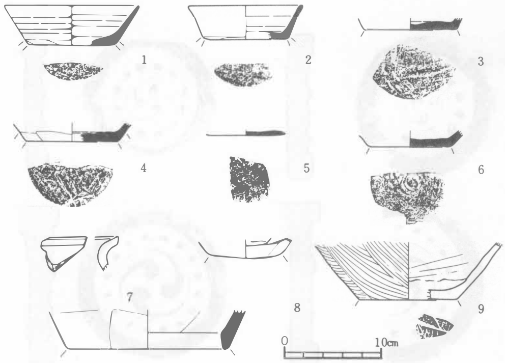
第15図 出土遺物実測図 (001号住居跡)
