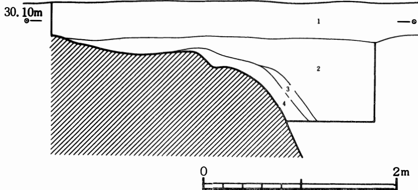
第13図 001号住居跡実測図
