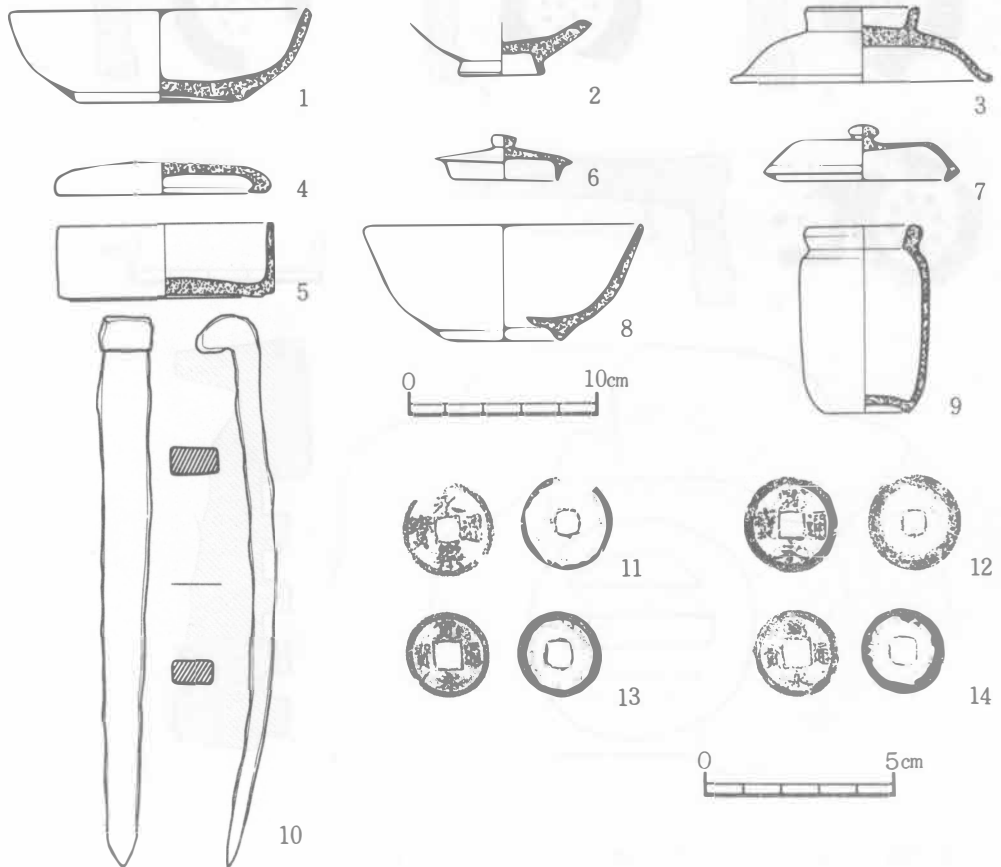
第16図 出土遺物実測図 (B3. B4 トレンチ)
