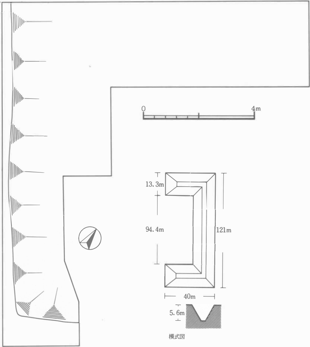
第2図 B1トレンチ遺構検出状況（馬出濠コーナー部）
