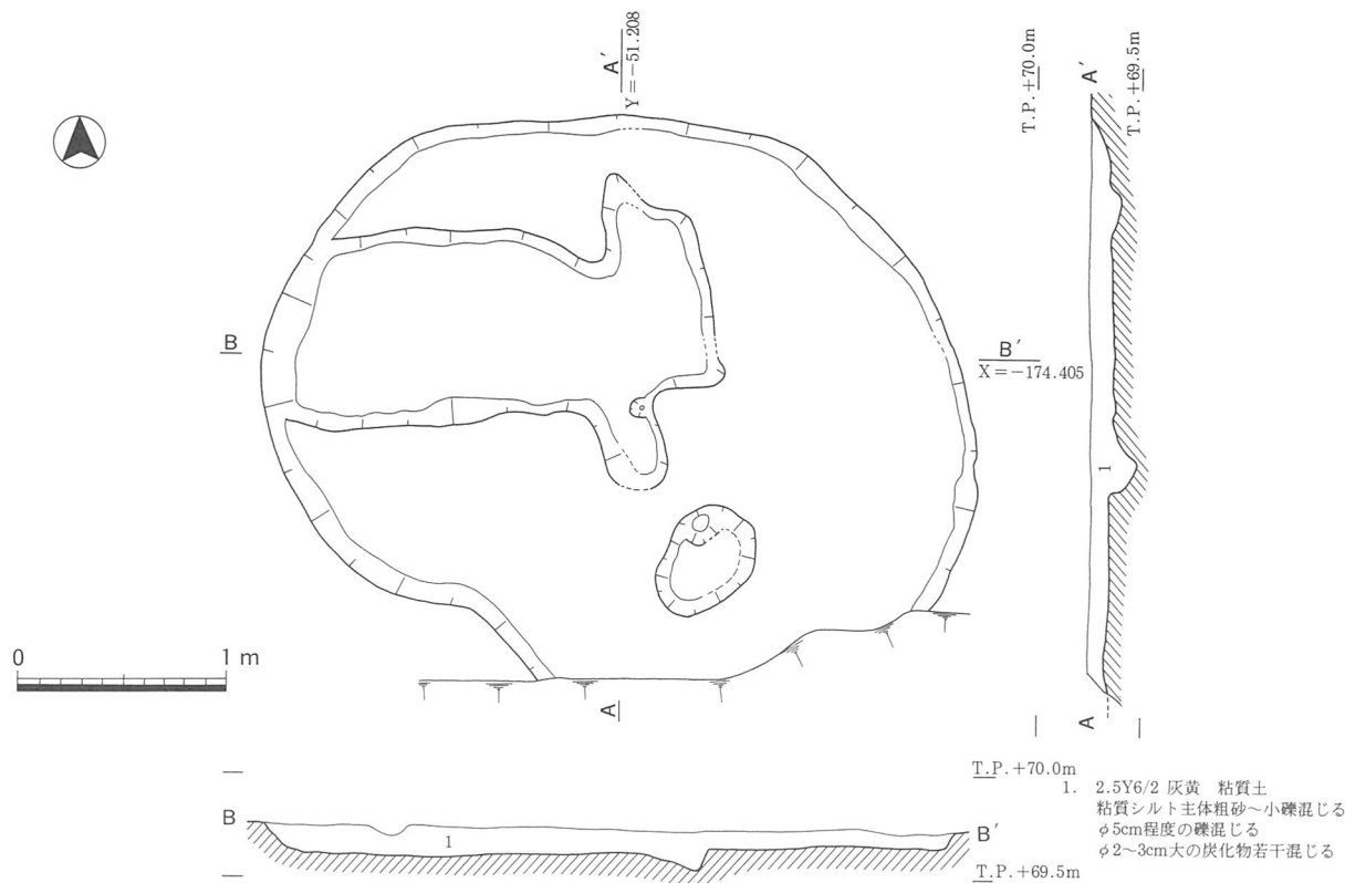
図20 土坑25 平・断面図
