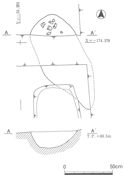
図11 土坑3 平・断面図
