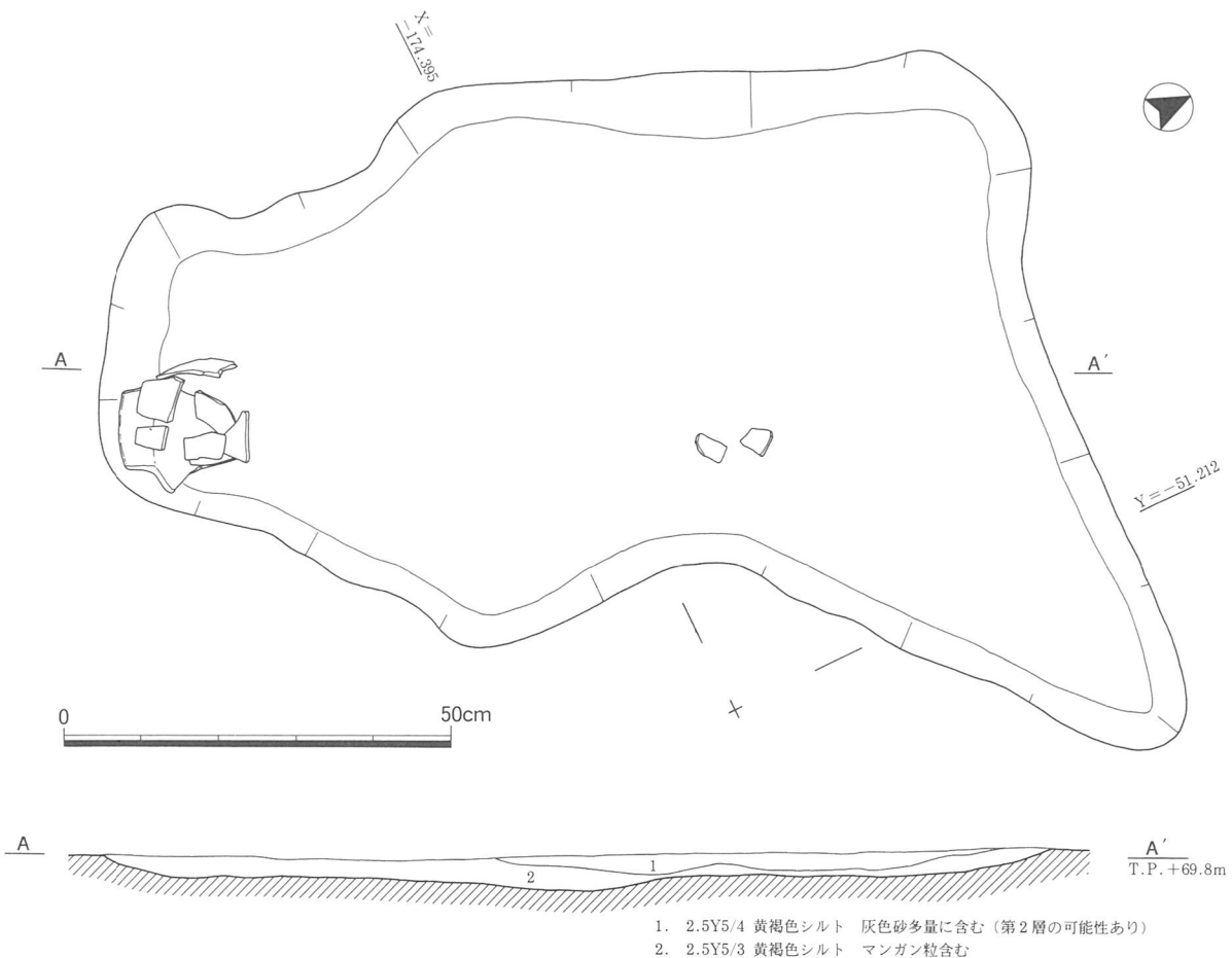
図16 土坑18 平・断面図
