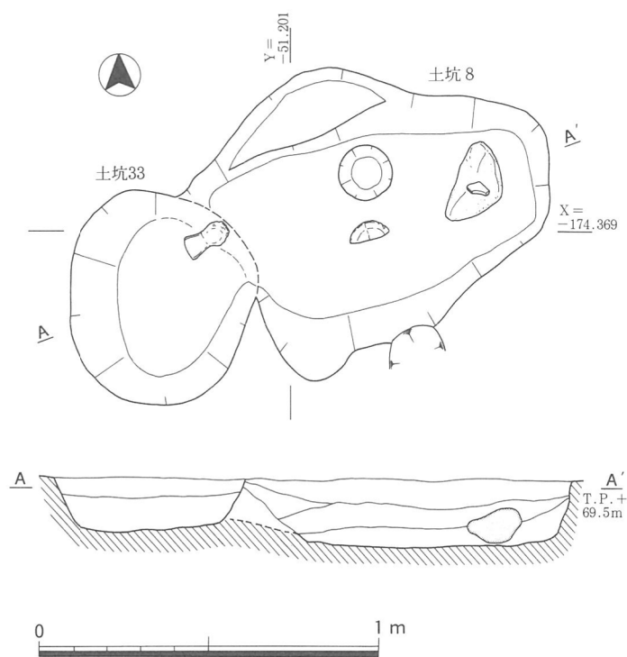
図10 土坑8・33 平・断面図
