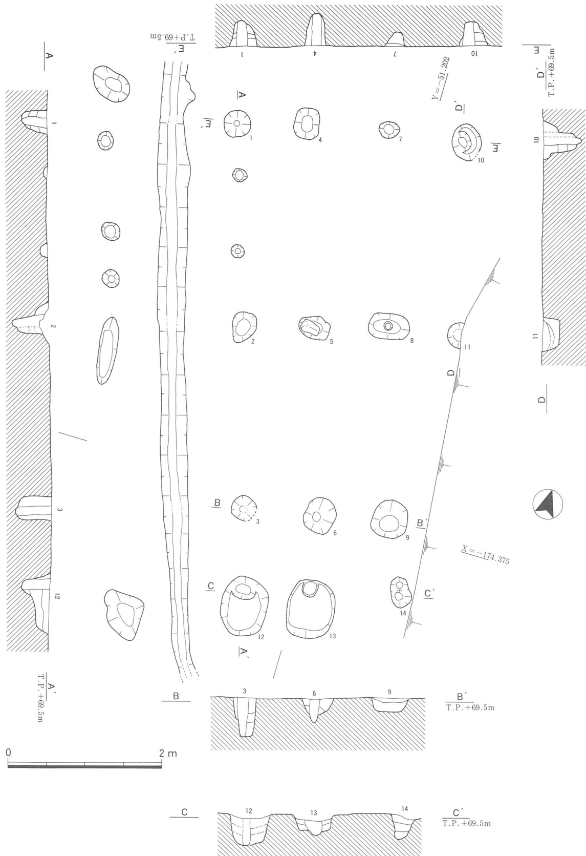
图8 建物7 平・断面図
