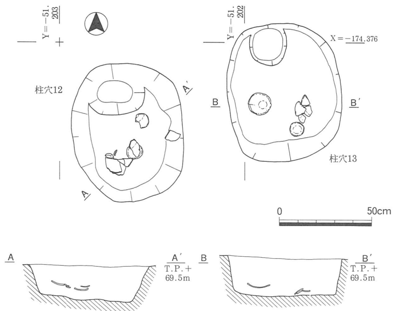
図9 建物7 柱穴12・13 平・断面図
