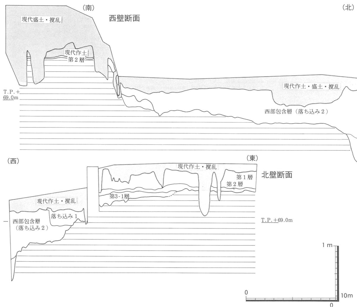
図4 調査地地形断面模式図
