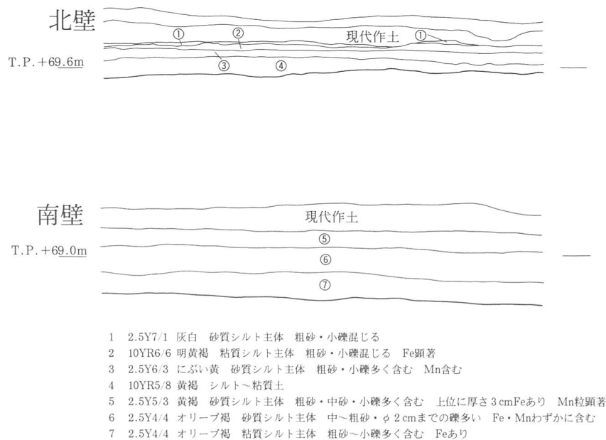
図5 土層断面図 (S = 1 / 40)
