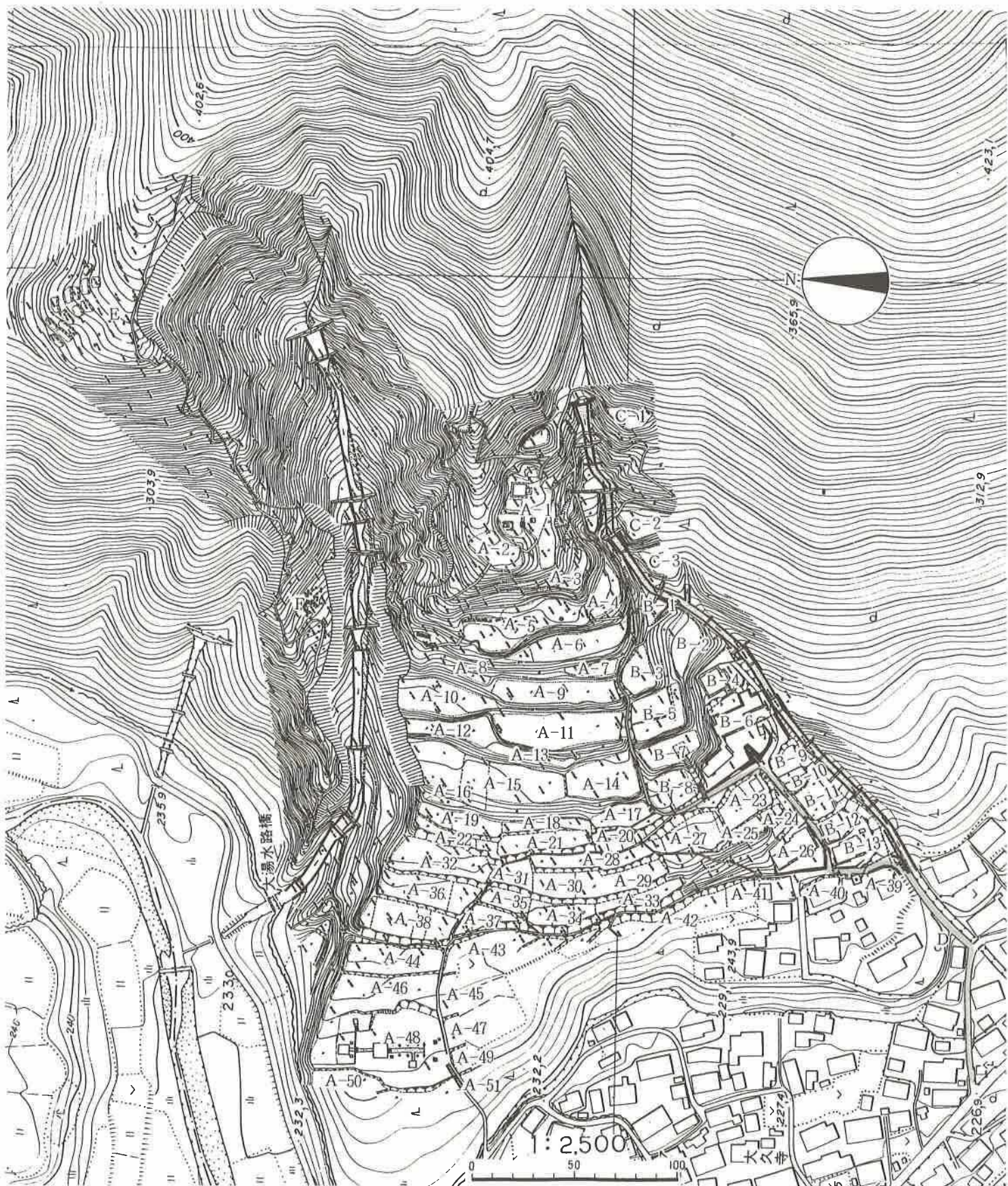
第3図 長尾寺跡平面図 (1/2500)
