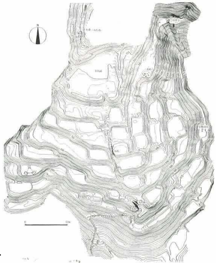
第8図 弥高寺跡測量図
