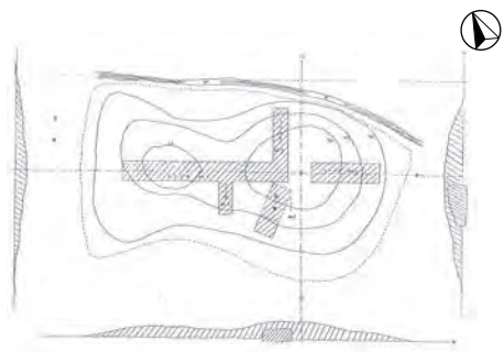
1号墳測量図
