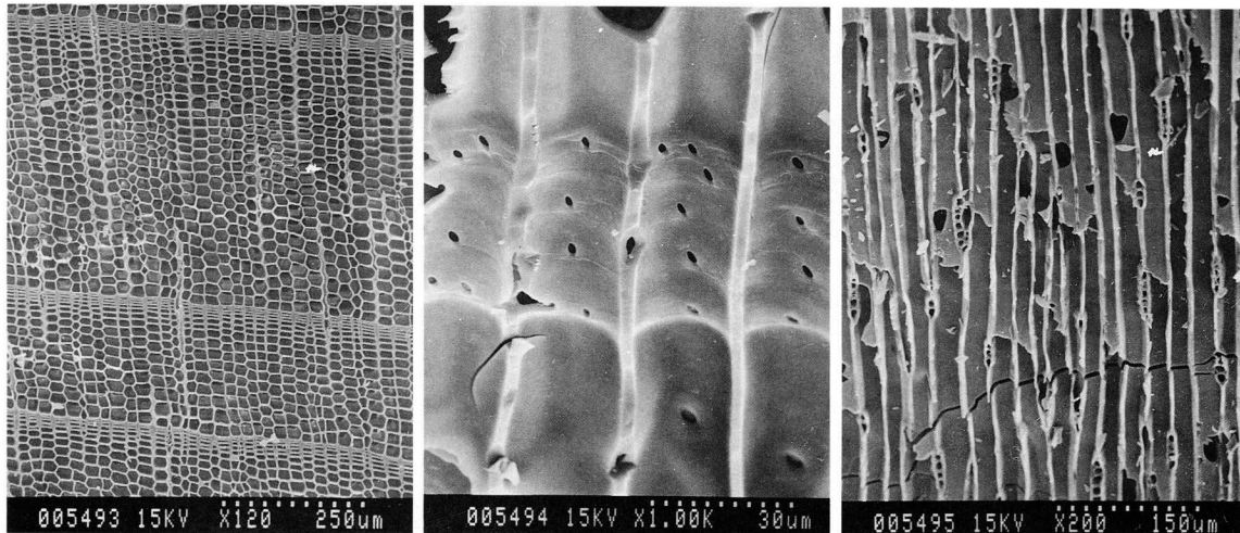
写真1 ヒノキ
