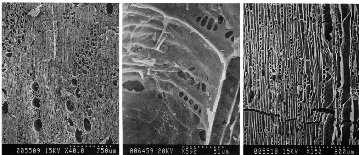
写真2 スダジイ
