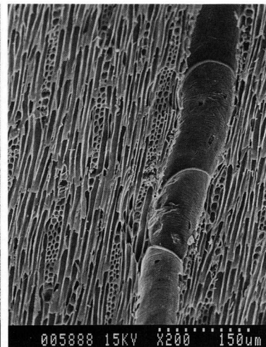
写真9 ムクノキ
