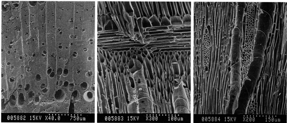
写真4 ヤマグワ
