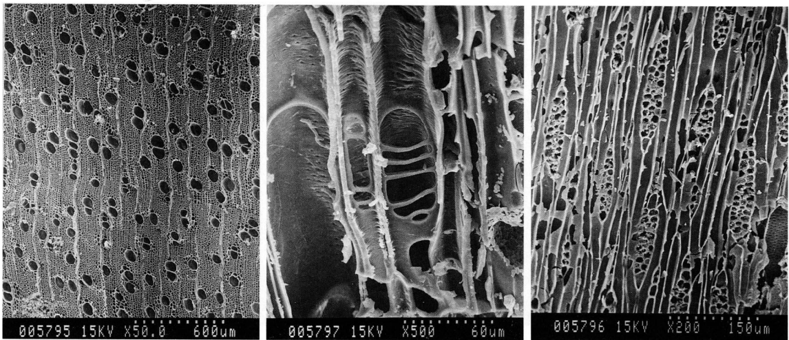
写真5 タブノキ
