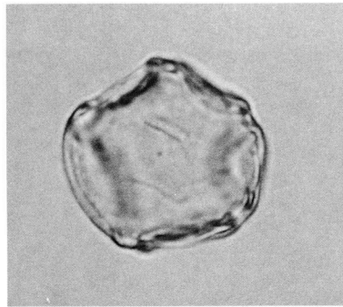
3 ハンノキ属
