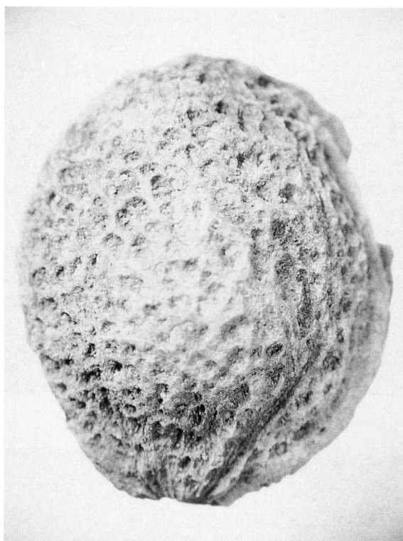
2 試料 2 ウメ核
