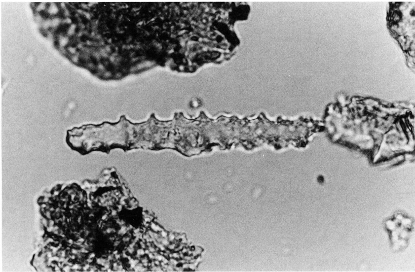
8 棒状珪酸体
