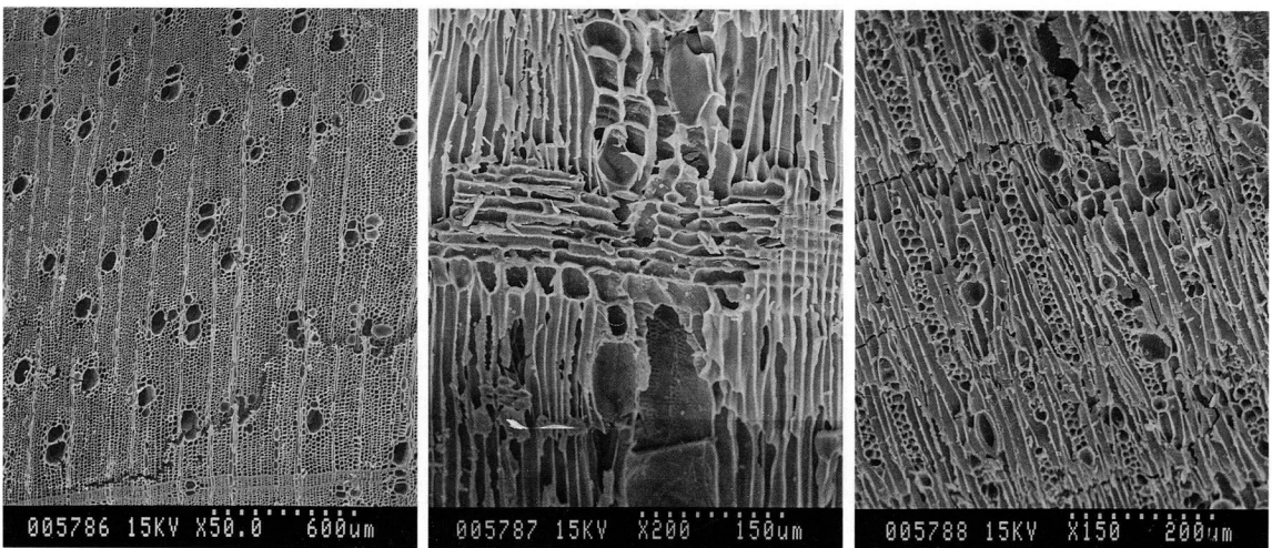
写真6 クスノキ
