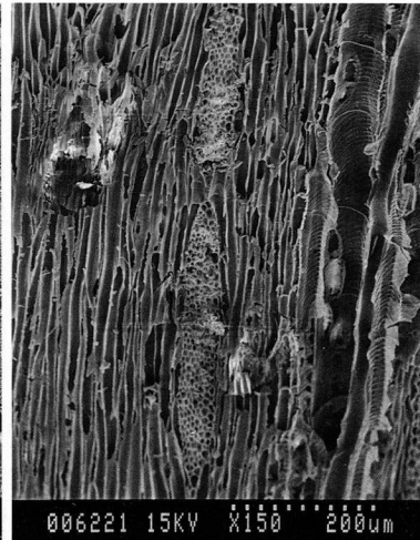
写真8 ケヤキ
