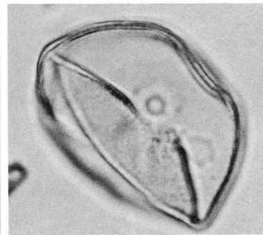
7 イネ科
