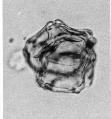
2 ハンノキ属
