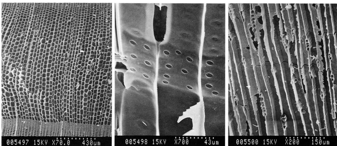
写真3 スギ
