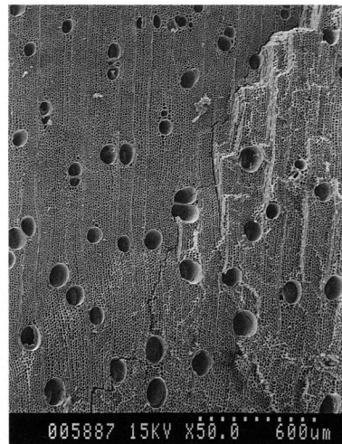
写真9 ムクノキ
