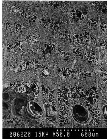
写真8 ケヤキ
