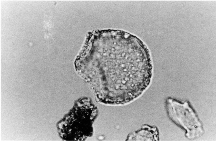
1 ヨシ属
