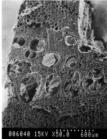
写真7 クリ
