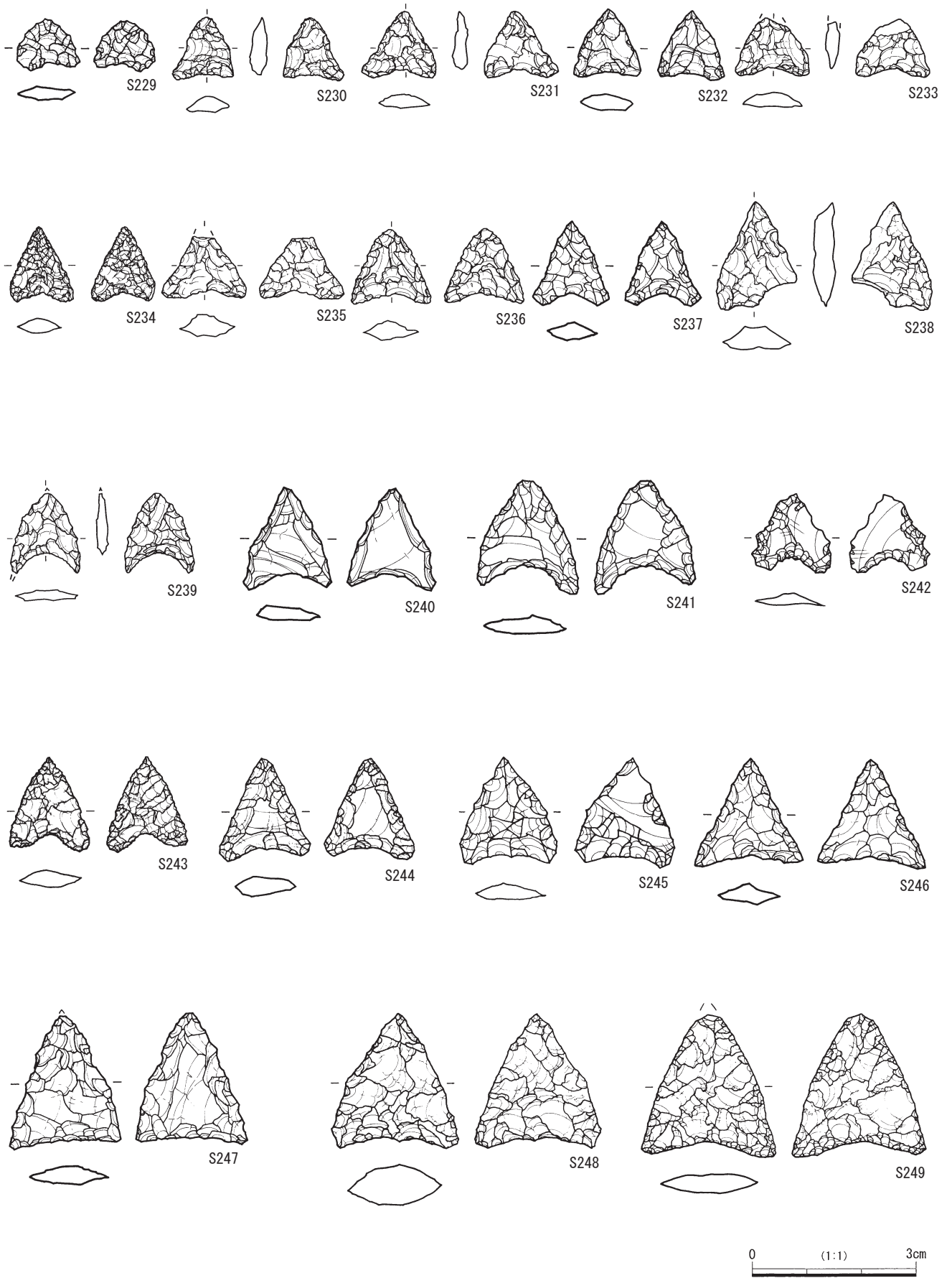
第2-134図 石鏃(1)
