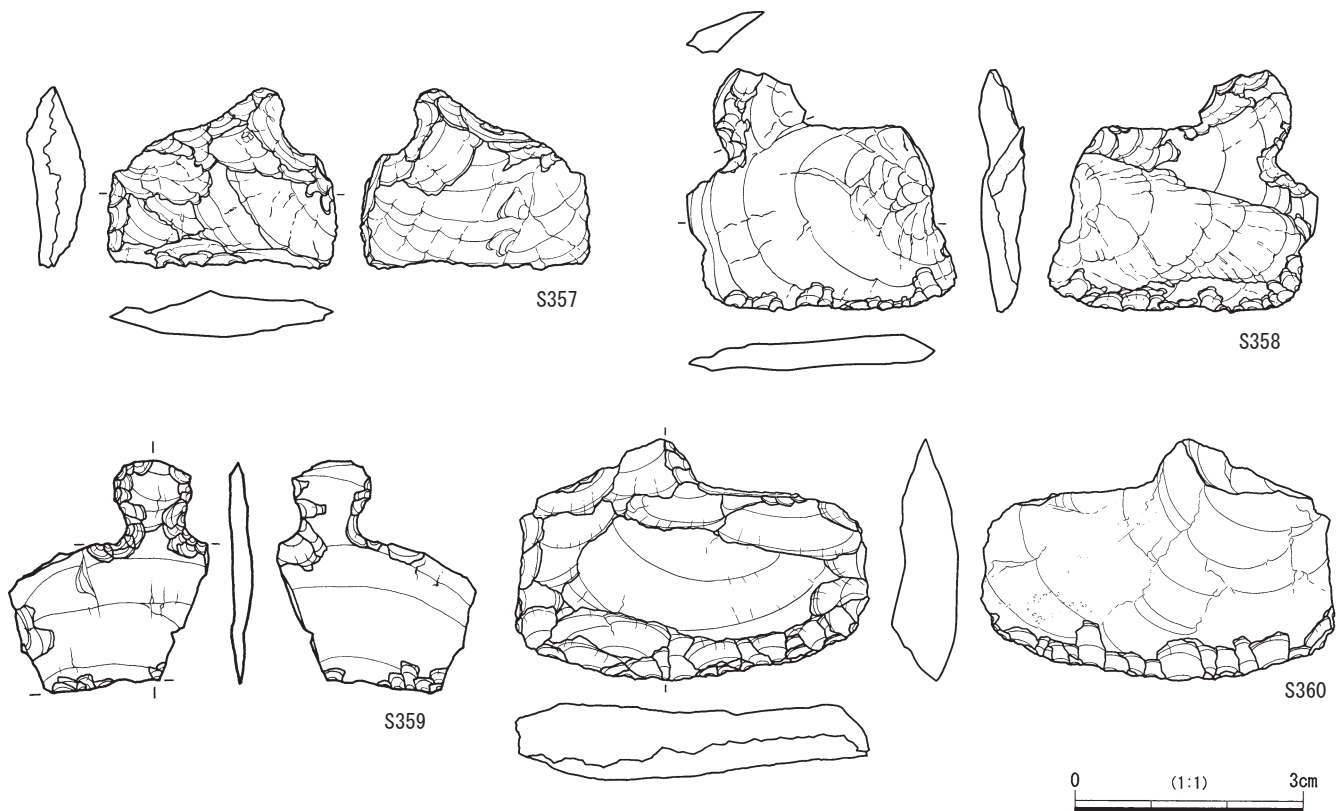
第2-143図 石匙(4)
