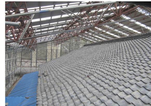
令和2年 解体調査前の屋根
