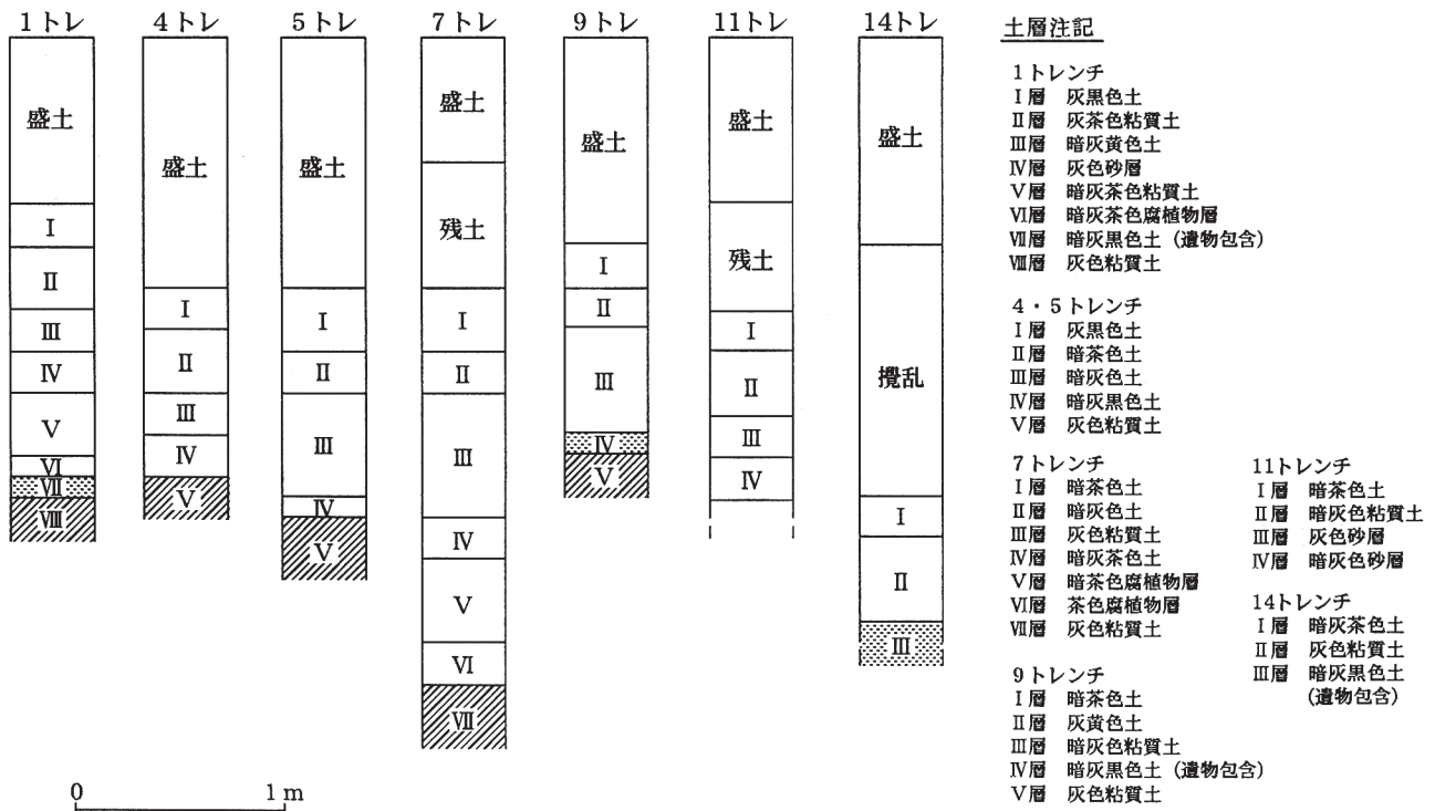
第14図 大塚遺跡土層柱状図
