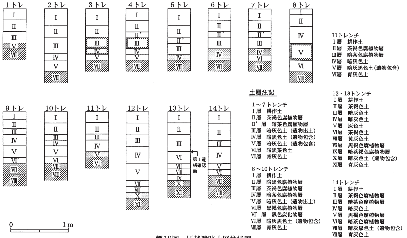
第18図 馬越遺跡土層柱状図
