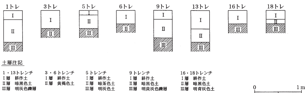
第4図 たて屋敷遺跡土層柱状図
