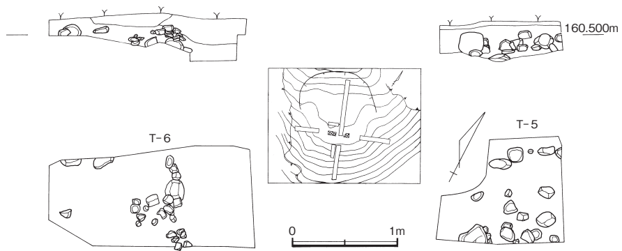
第10図 T-5・T-6実測図 (S=1/50)
