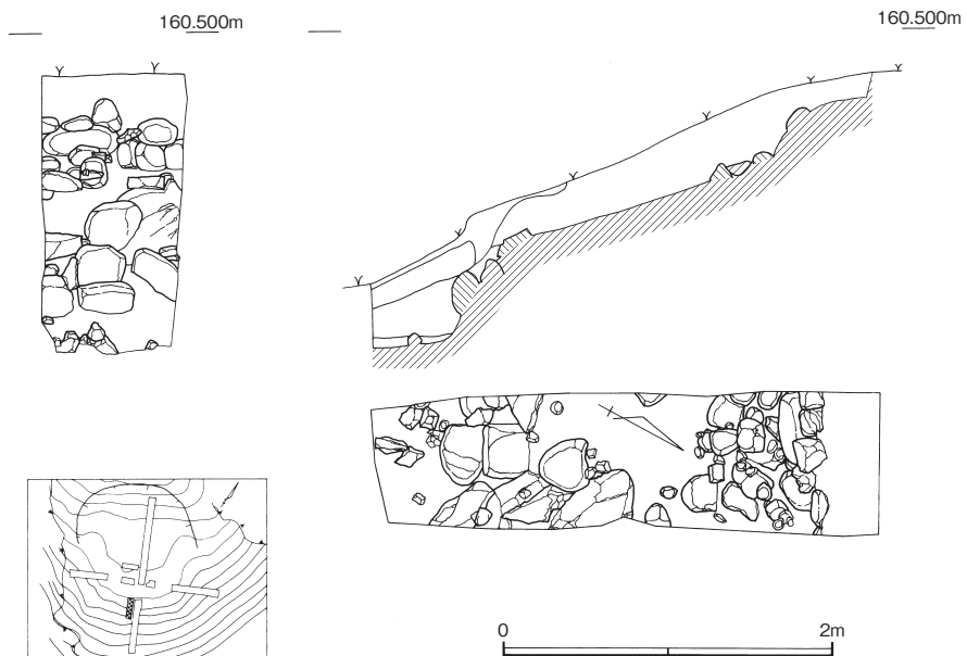
第13図 T-8 実測図（S=1/50）
