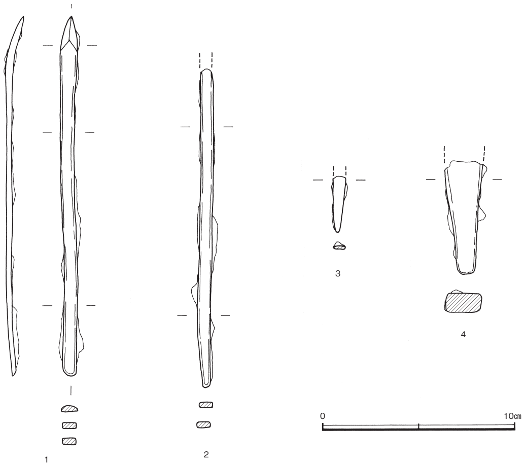
第15図 出土鉄器 (S=1/2)
