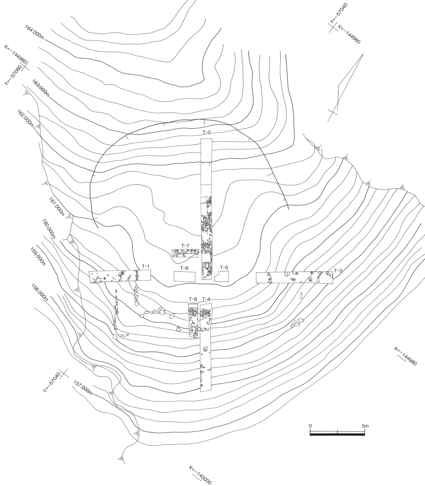
第5図 墳丘測量図とトレンチ配置図 (S=1/200)
