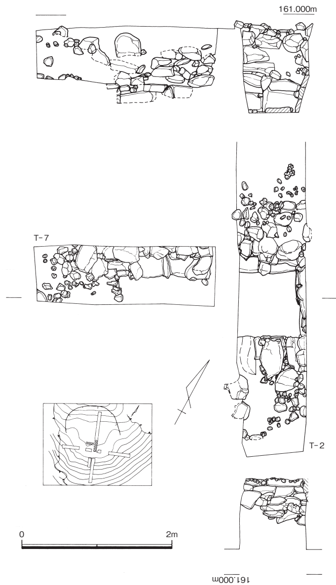
第11図 T-2・T-7実測図 (S=1/50)
