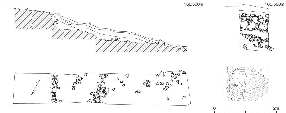
第6図 T-1 実測図 (S=1/60)
